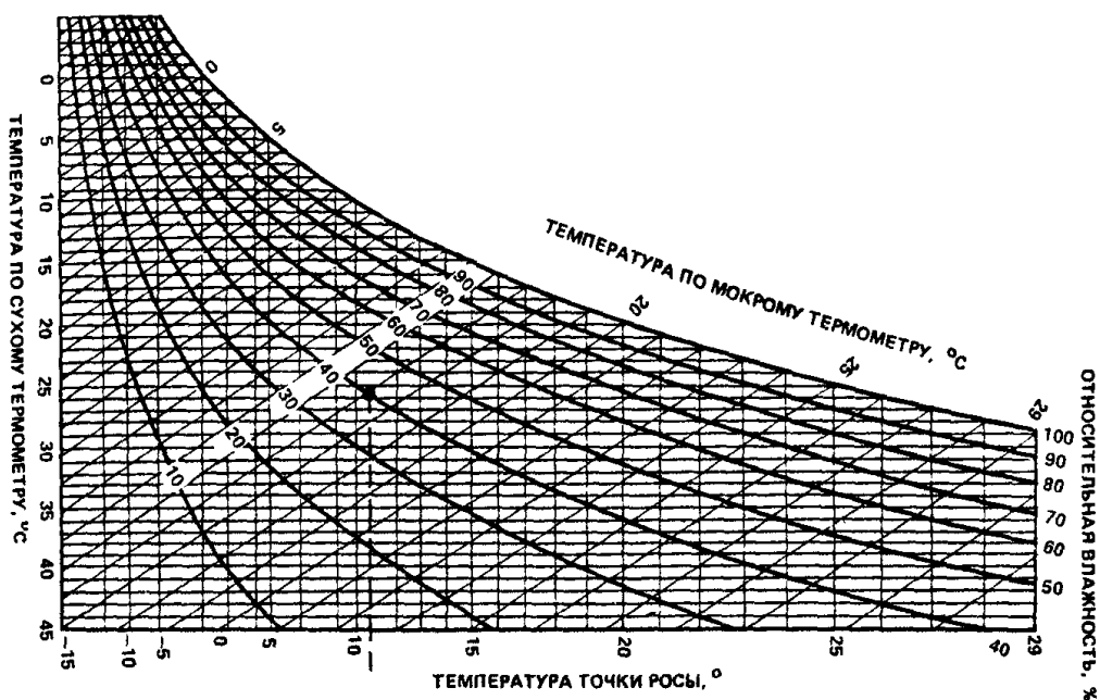
Психрометрическая диаграмма
