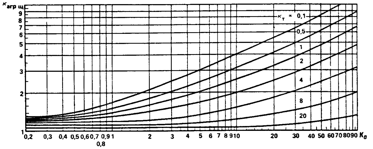
Рис. 9. Номограмма для определения коэффициента k_{agr\ \sigma}
