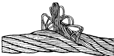
Рис. 10. Выдавливание сердечника
