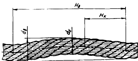
Рис. 8. Волнистость каната (объяснение в тексте)
