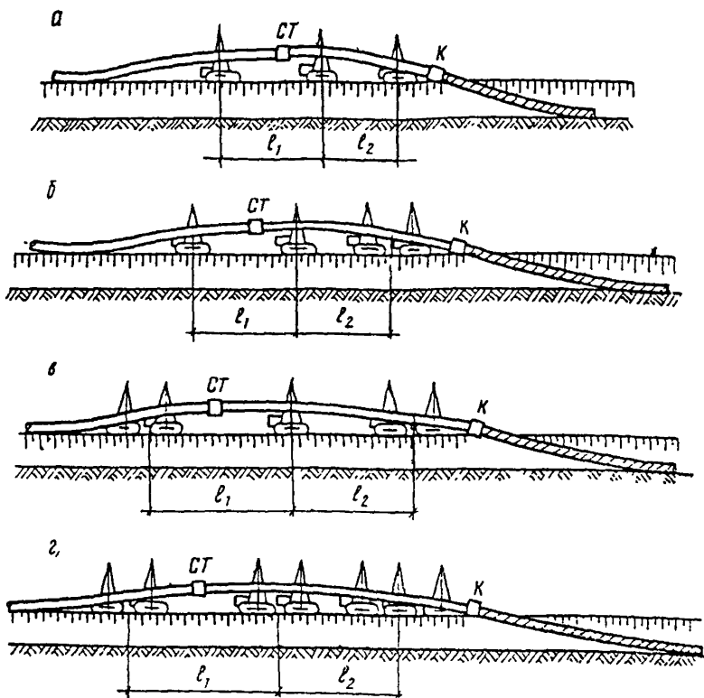
Рис.10. Схемы расстановки трубоукладчиков и машин в изоляционно-укладочной колонне при совмещенном способе производства работ для трубопроводов различных диаметров: а - 529-820 мм; б - 1020 мм; в - 1220 мм; г - 1420 мм; СТ - сушильная установка; К - комбайн для очистки и изоляции трубопровода; l_1, l_2 - расстояния между трубоукладчиками и группами трубоукладчиков
