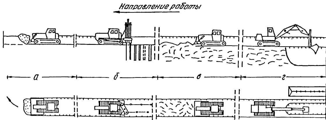
Рис.5. Схема разработки траншей в мерзлом грунте с предварительным рыхлением их буровзрывным способом: а - снятие снежного покрова; б - рыхление грунта буровзрывным способом; в - планировка разрыхленного грунта; г - разработка траншей
