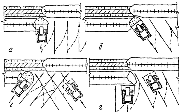
Рис.7. Схемы производства работ по засыпке уложенного трубопровода бульдозером: а-прямолинейными проходами; б-косопоперечными параллельными проходами; в-косопоперекрестными проходами; г-комбинированным способом
