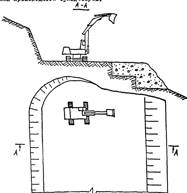
Рис.4. Схема разработки полков экскаватором
