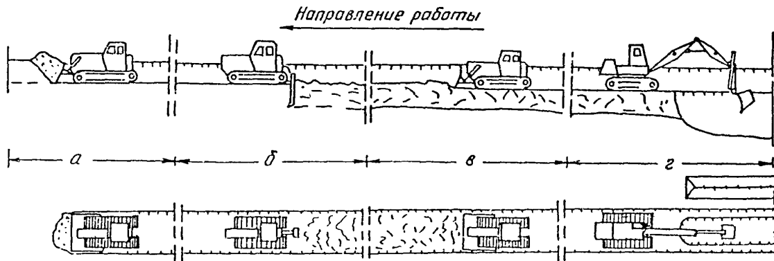
Рис.6. Схема разработки траншеи в мерзлом грунте с предварительным рыхлением его механическим рыхлителем: а - снятие снежного покрова; б - рыхление грунта механическим рыхлителем; в - планировка разрыхленного грунта; г - разработка траншеи экскаватором
