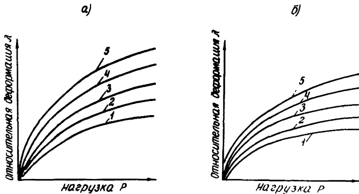
Рис.5.4. Зависимость относительной деформации образцов глинистых грунтов от нагрузки при коэффициенте увлажнения Kw_1 (а) и Kw_2 < Kw_1 (б): 1,2,3,4,5 – при коэффициентах уплотнения соответственно K_{c1} > K_{c2} > K_{c3} > K_{c4} > K_{c5}
