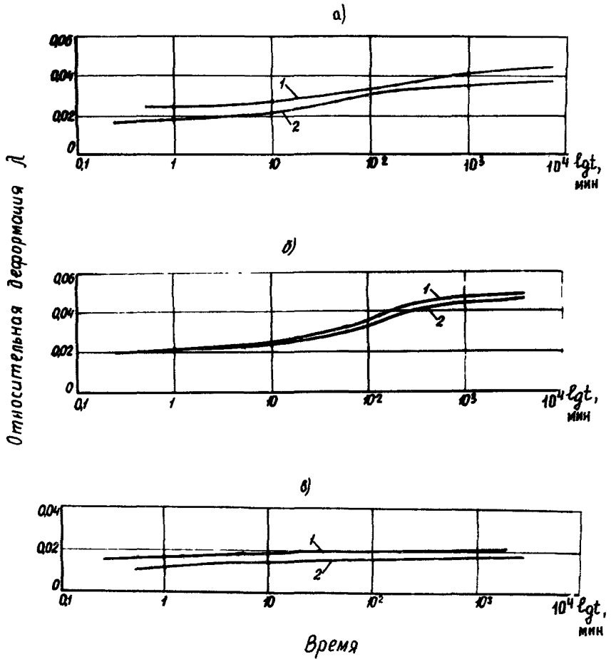
Рис.2. Зависимость относительной деформации от времени при P_{упл} = 5 \text{ МПа} : а- K_w = 1,4 ; \rho_d/\rho_{d \text{ макс}} = 0,9 ; б- K_w = 1,4 ; \rho_d/\rho_{d \text{ макс}} = 0,95 ; в- K_w = 1,2 ; \rho_d/\rho_{d \text{ макс}} = 0,9 ; 1- h_{обр} = 2 \text{ см} ; h_{ф} = 1 \text{ см} ; 2- h_{обр} = 2,5 \text{ см} ; h_{ф} = 2,5 \text{ см}
