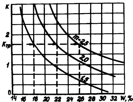
Рис.5.1. Зависимость прочностных характеристик грунта и коэффициента устойчивости откоса от влажности грунта
