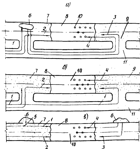
Рис.8.4. Схемы организации работ по устройству вертикальных песчаных дренай: 1-автовозка песка; 2-то же, суглинка; 3-перевозка песка со склада автомобилями, скреперами; 4-то же, транспортными тележками (для дренай); 5-дополнительная перевозка песка на склад; 6-склад песка; 7-нижний дренаирующий слой; 8-суглинок; 9-верхний дренаирующий слой; 10-вертикальные дренаи; 11-подъездный путь
