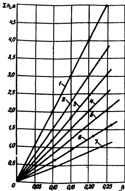
Рис.6.1. Зависимость суммарной толщины прослоек \Sigma h_i от параметра \beta для насыпей различной высоты: 1-20 м; 2-15 м; 3-12 м; 4-10 м; 5-8 м; 6-6 м; 7-4 м
