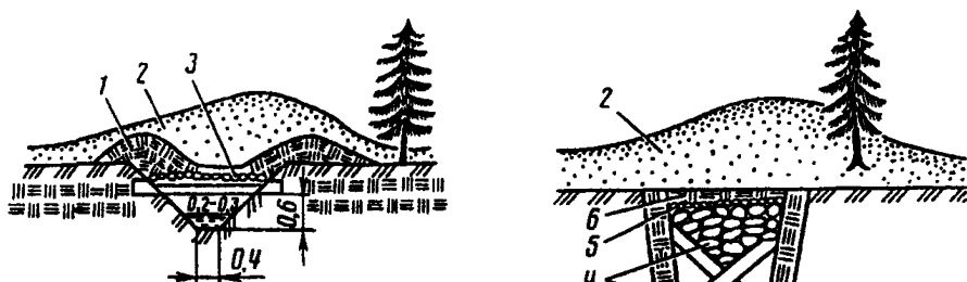
Рис. 6.14. Утепленные водоотводные канавы:
