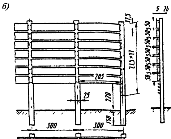
Рис 6 4 Снегопредува- ющие заборы
