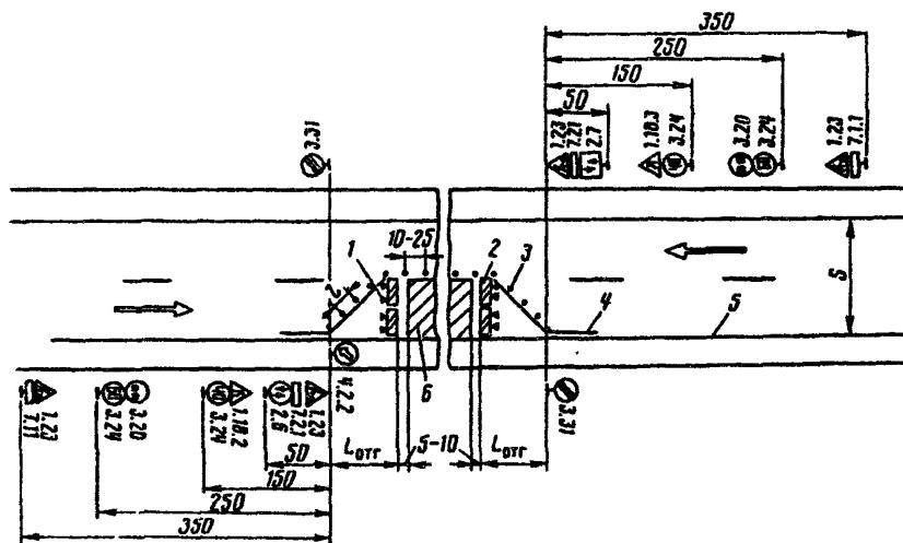
Рис. 4.5. Размещение технических средств организации движения в местах производства дорожных работ:
