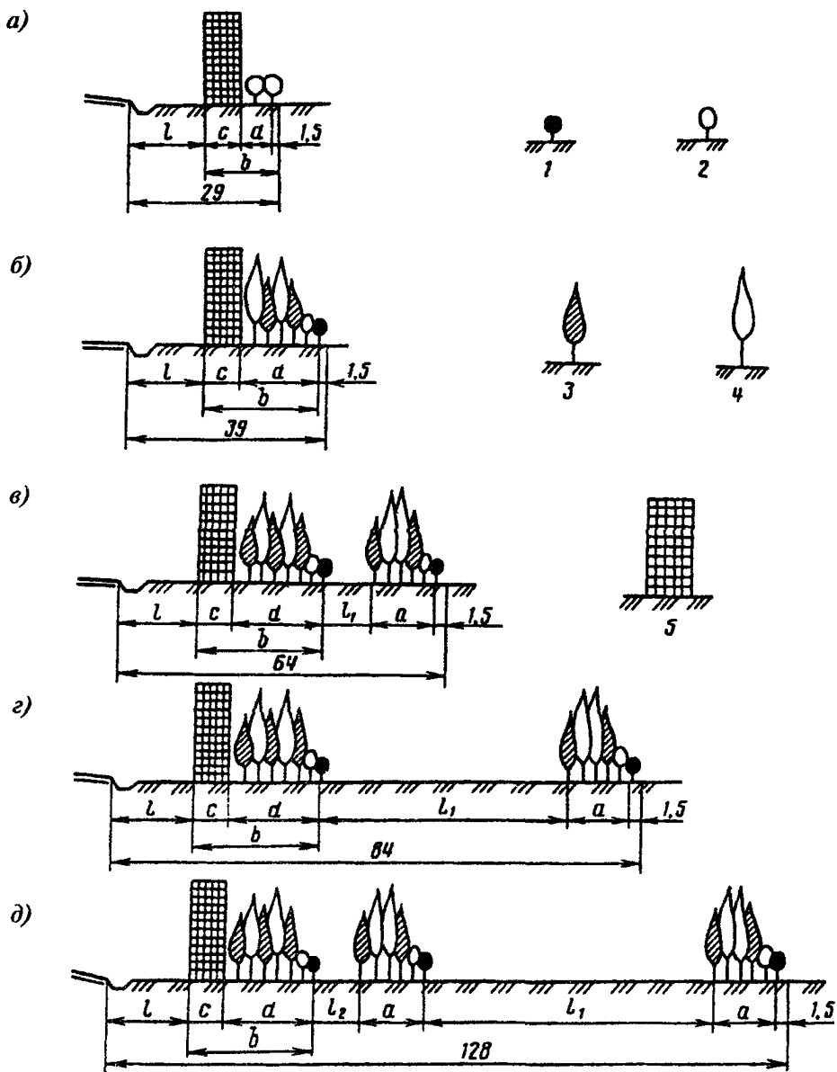
Рис. 10.2. Типовые схемы усиления существующих снегозащитных насаждений: a — при объеме снегопереноса до 25 \text{ м}^3/\text{м} ; b — до 50 \text{ м}^3/\text{м} ; в — до 100 \text{ м}^3/\text{м} ; г — до 150 \text{ м}^3/\text{м} ; д — до 250 \text{ м}^3/\text{м} ;
