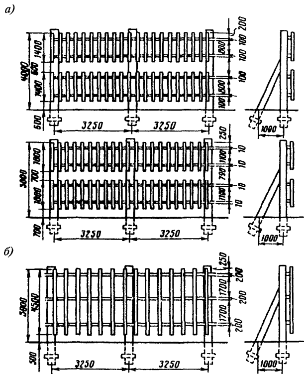
Рис. 6.3. Снегозадерживающие заборы
