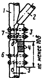
Рис. 9.11. Ремонт сопряжения подкоса со сваяей 1 — стойка или свая; 2 — подкос; 3 — подбабок; 4 — клинья; 5 — подбабок усиления; 6 — болт \varnothing 16 мм, l = 500 мм; 7 — скол
