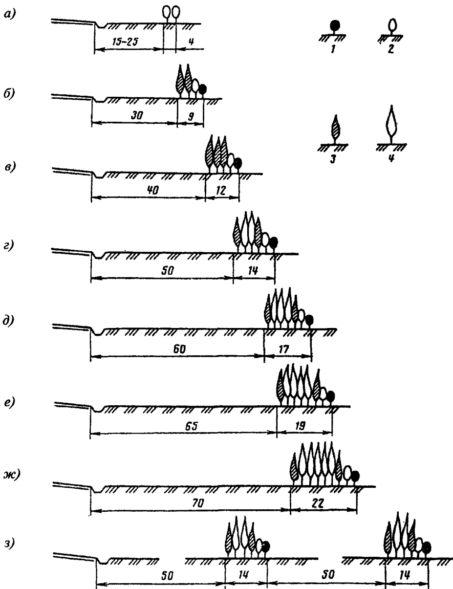
Рис. 10.1. Типовые схемы снегозащитных насаждений автомобильных дорог: а — при объеме снегопереноса до 25 \text{ м}^3/\text{м} ; б — до 50 \text{ м}^3/\text{м} ; в — до 75 \text{ м}^3/\text{м} ; г — до 100 \text{ м}^3/\text{м} ; д — до 125 \text{ м}^3/\text{м} ; е — до 150 \text{ м}^3/\text{м} ; ж — до 200 \text{ м}^3/\text{м} ; з — до 250 \text{ м}^3/\text{м} ; 1 — кустарники низкие; 2 — кустарники высокие; 3 — деревья низкокронные; 4 — деревья высококронные
