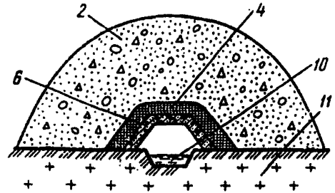
Рис. 6.16. Каптажно-дюкерное устройство:
