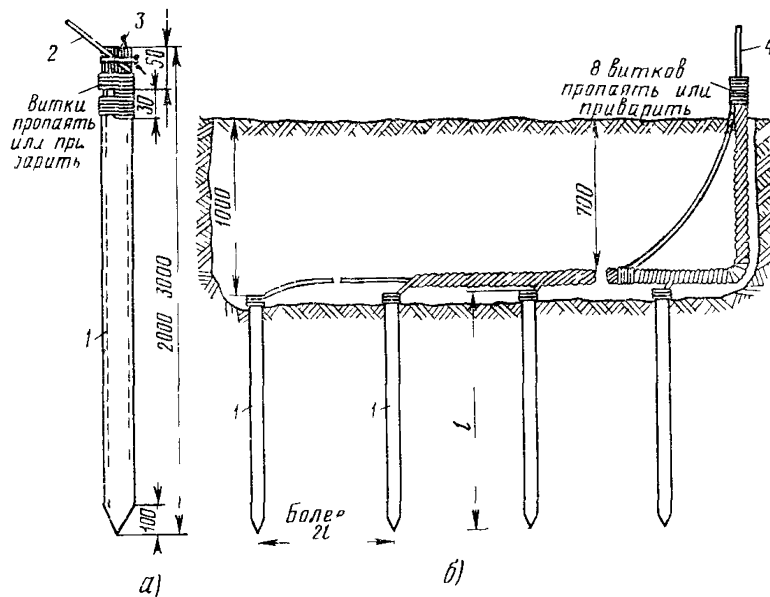
Рис 728 Устройство заземления а — одной трубой, б — несколькими трубами
