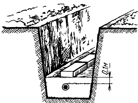
Рис 51 Дополнительная защита кабеля от возможных механических повреждений
