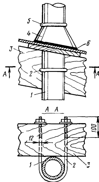
Рис 87 Крепление стойки стальным хомутом
