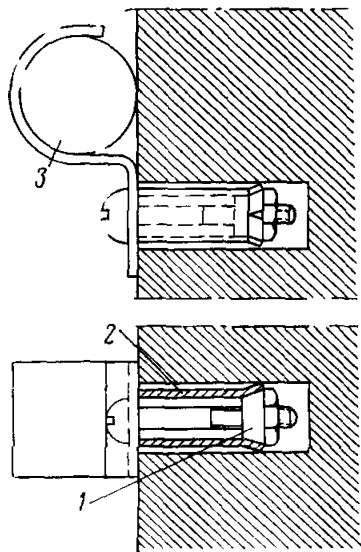
Рис 9 46 Крепление фасонных скоб винтами с распорными гайками:
