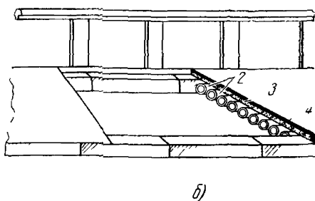
Рис 3 36 Прокладка трубопровода по мосту на деревянных колодках
