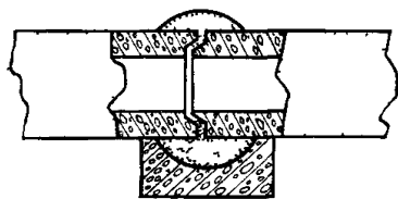
Рис 322 Заполнение массой зазоров снизу и сверху
