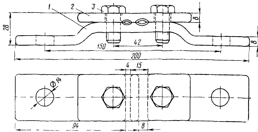
Рис. 7.40. Штампованная столбовая консоль:
