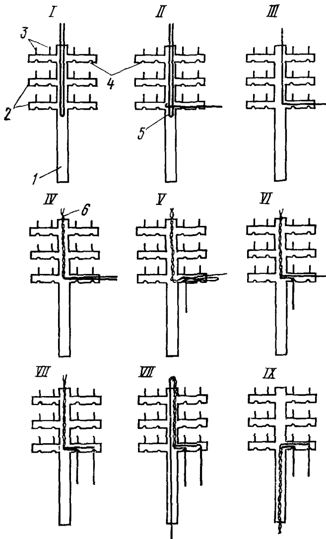
Рис 8 19 Протаскивание провода ЛТВ-В (ЛТР-В) через стойку:
