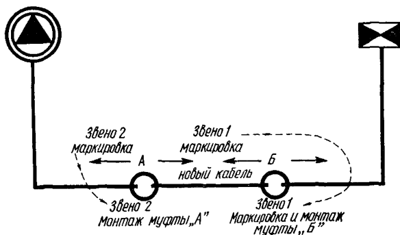
Рис. 10.55. Замена пролета двумя звеньями монтажников
