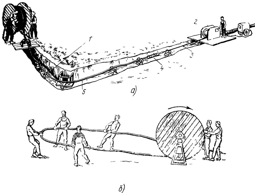
Рис. 5.4. Способы прокладки кабеля в готовую траншею а — протаскивание кабеля по роликам; б — разноска кабеля вручную вдоль траншеи напрямую или методом петли — ролик; 2 — лебедка, 3 — трос, 4 — кабельный чулок, 5 — кабель
