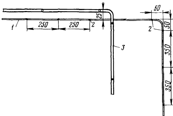
Рис. 13.2. Прокладка провода 1 \times 2 :
