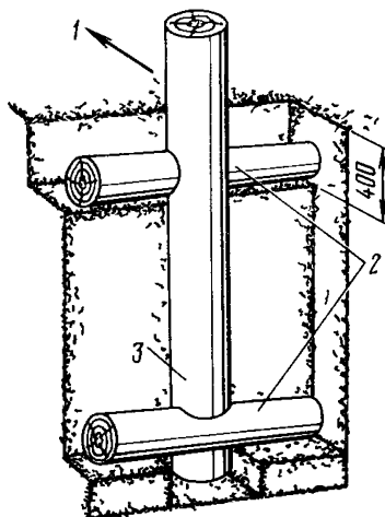
Рис 718 Укрепление опоры лежнями
