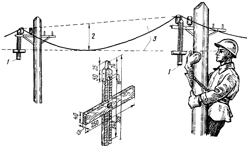
Рис. 7.32. Определение стрелы провеса провода:
