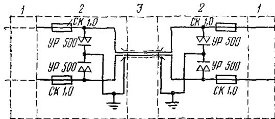
Рис. 14.34 Схема защиты кабельных вставок:
