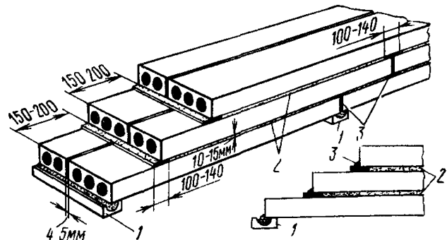
Рис 3.27. Блок из нескольких рядов бетонных труб: 1 — железобетонная подкладка; 2 — песок; 3 — цементно-песчаная масса
