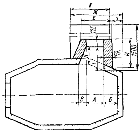
Рис 344 Типовые угловые сборные из проходных и угловых вставок железобетонные колодцы типов ККС-3, ККС-4 и ККС-5 многогранной формы (высоту вставки Л см на рис. 345)
