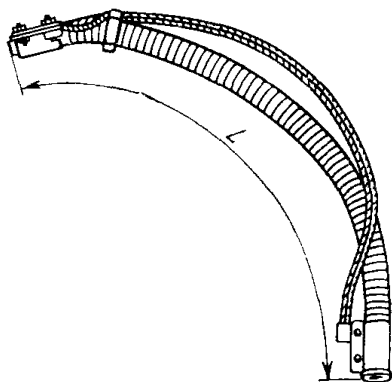
Рис. 9.27. Гибкий комплектный ввод
