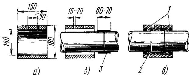
Рис. 3.17. Способ с применением асбестоцементных муфт, заливаемых битумным компаундом: а — асбестоцементная муфта; б — наложение на стык смоляной ленты; в — готовый стык
