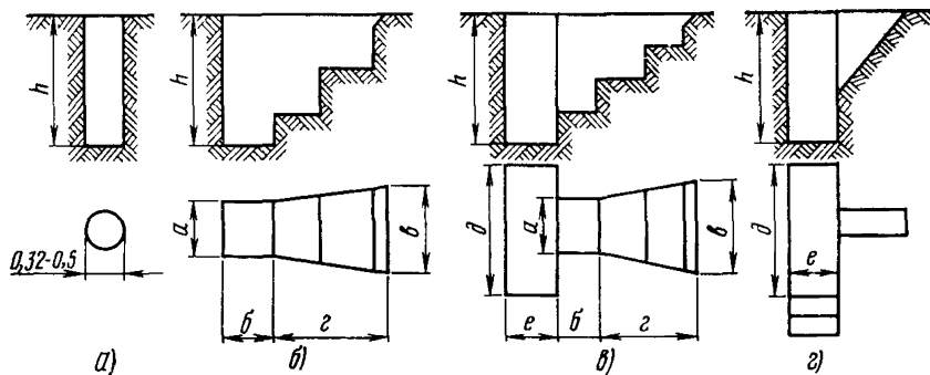
Рис. 7.12. Форма ям:
