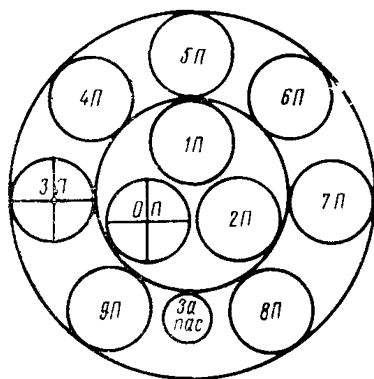
Рис 10 64 Порядок распределения жил по плинтам бокса 100x2 в кабеле пучковой скрутки
