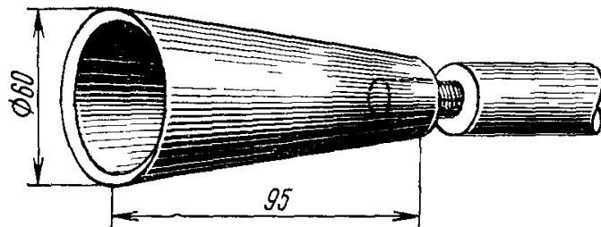
Рис 46 Воронка для извлечения палок из канала
