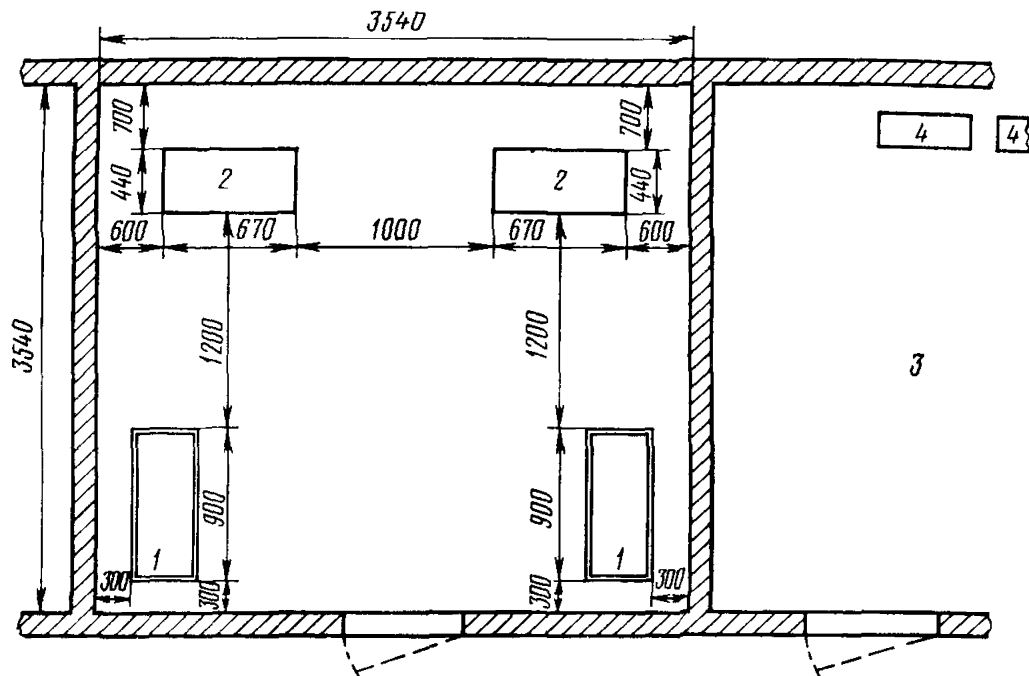
Рис. 12.3. Размещение КСУ на 30 или 60 кабелей: 1 — шахта; 2 — компрессорная группа; 3 — блок осушки и автоматики; 4 — распределительный стив
