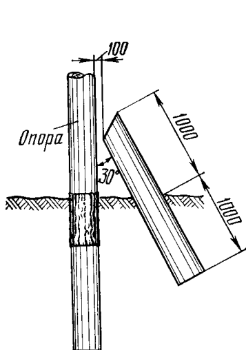
Рис 7.25. Установка отбойной тумбы
