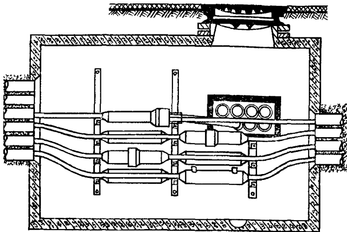
Рис 10 1 Расположение муфт в колодцах типа ККС-5
