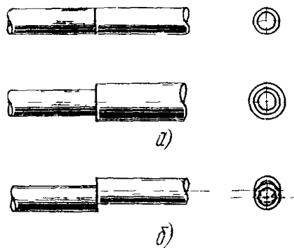
Рис 3 14 Положение стыкуемых концов труб: а — правильное; б — неправильное
