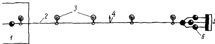
Рис. 12.25. Манометрический метод определения места негерметичности оболочки кабеля:
