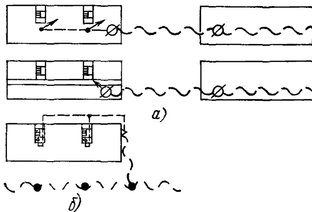
Рис 910 Варианты устройства воздушных вводов в здания а — со стоечных линий, б — со столбовых линий
