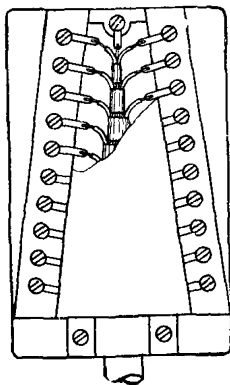
Рис 10 59 Ввод и включение кабеля в распределительную коробку типа КРО 10x2
