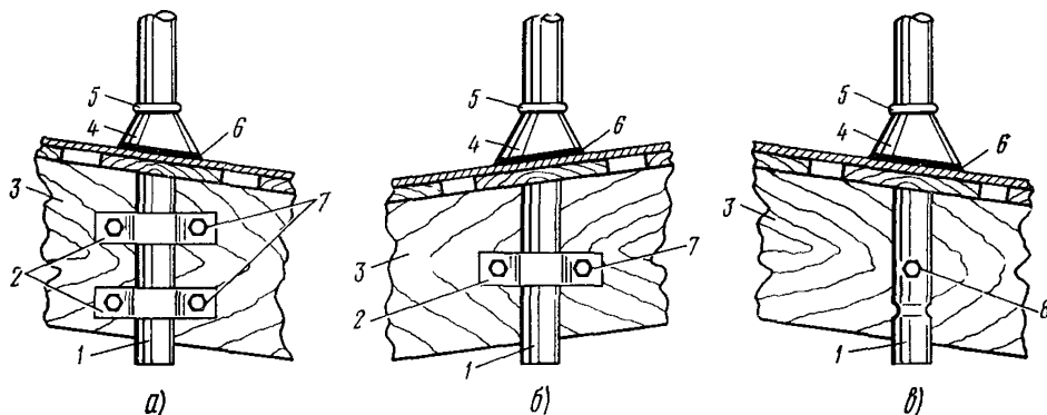
Рис. 8.5. Крепление стоек:
