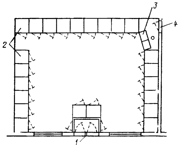
Рис. 13.9. Переговорный павильон таксофонов:
