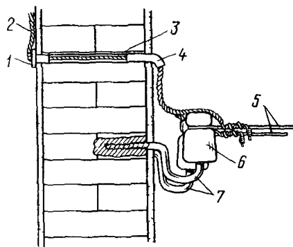
Рис. 137. Устройство ввода с крюков
