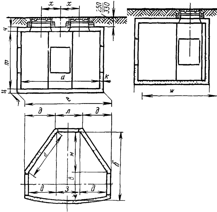
Рис 352 Монолитные железобетонные станционные колодцы для станции на 3000, 6000, 10 000 и 20 000 номеров
