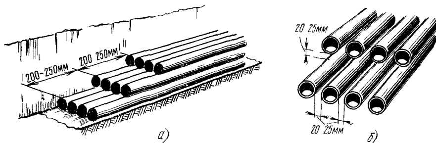
Рис 312 Положение труб в блоке a — сдвиг концов труб в каждом последующем ряду, б — расстояние между трубами в ряду и между рядами
