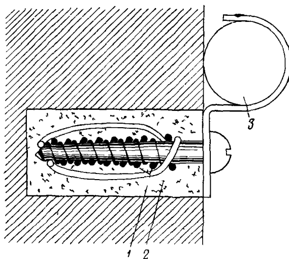
Рис 945. Крепление фасонных скреп (скоб) к кирпичным, бетонным, шлакобетонным стенам шурупами на спиралях:
