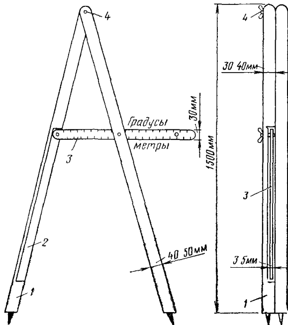
Рис 75 Угломер для определения величины угла поворота линий
