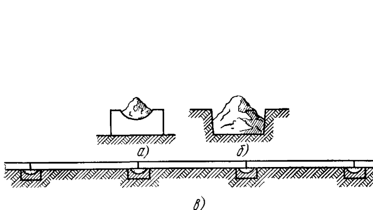
Рис 320 Заполнение подкладок или выемок цементно-песчаной массой и размещение труб а — заполнение подкладки; б — заполнение выемки; в — размещение труб над выемками или подкладками
