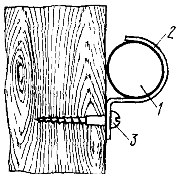
Рис 944 Крепление фигурной скрепы к деревянной стене.
