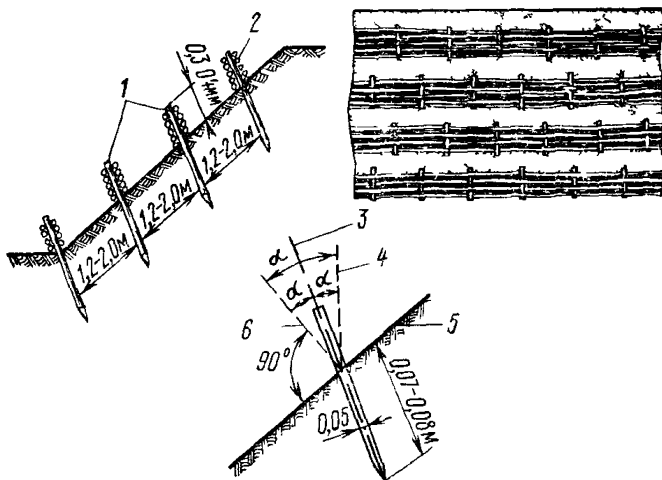
Рис 213 Схема крепления откоса плетневыми рядами
