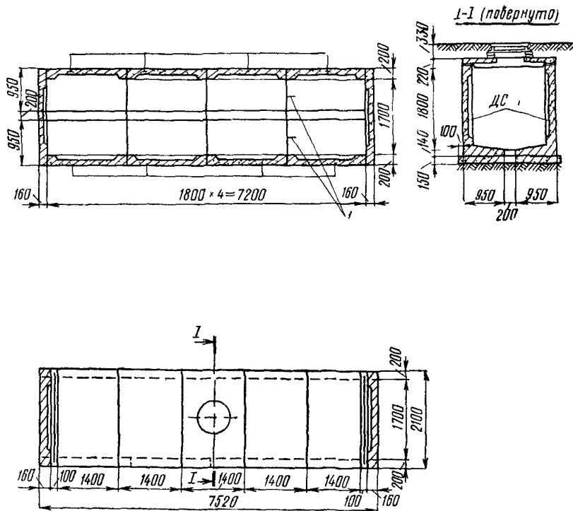
Рис 358 Эскиз сборки нетипового сборного железобетонного колодца из унифицированных (типовых) железобетонных элементами I — серги для блоков
