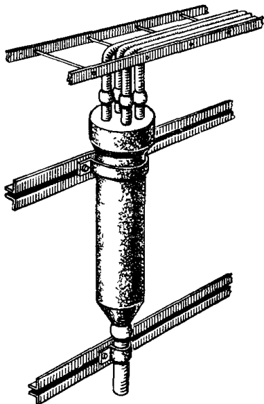
Рис. 10.2. Крепление вертикальных станционных разветвительных муфт к каркасу
