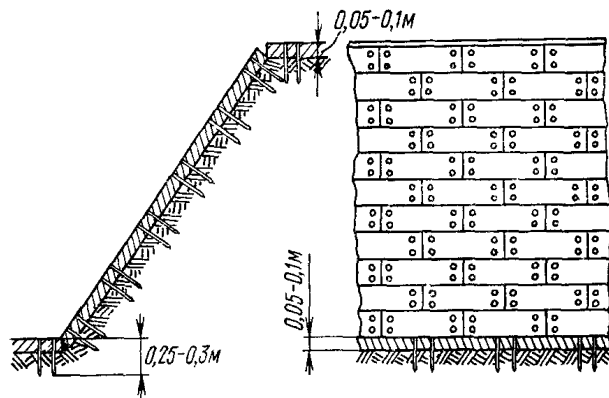
Рис 2 12 Схема крепления дерна колышками
