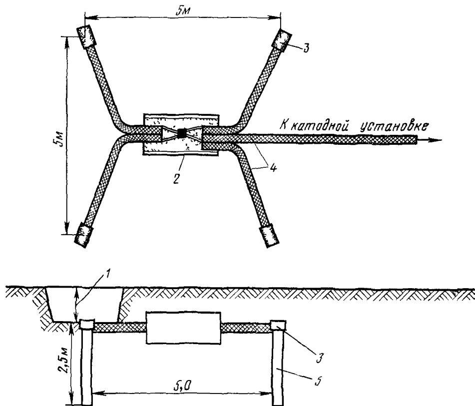
Рис. 14.22. Устройство анодного заземления для катодной защиты:
