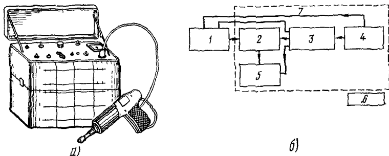
Рис. 12.21. Батарейный галлоидный теческатель типа БГТИ-5: а — общий вид; б — структурная схема:
