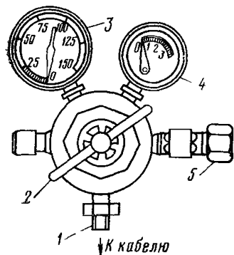
Рис. 12.13. Редуктор:
