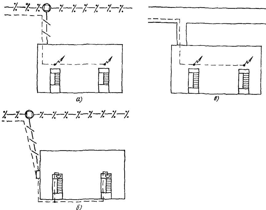
Рис. 91 Варианты устройства подземных вводов в здания
