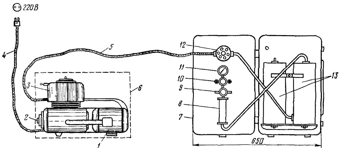
Рис. 12.8. Компрессорная установка переносного типа КМ-77:
