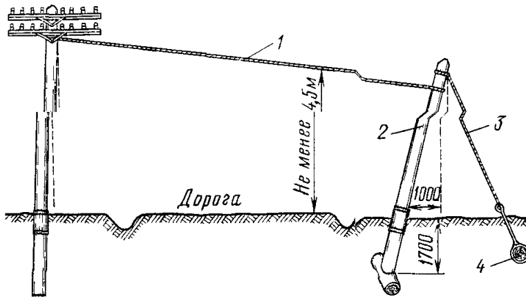
Рис. 7 23 Устройство оттяжного столба. 1 — оттяжка, 2 — оттяжной столб; 3 — контроттяжка, 4 — якорь
