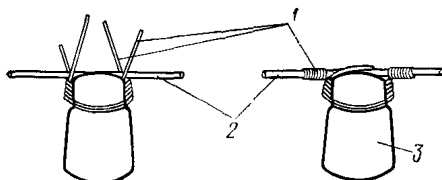
Рис. 7.33. Вязка проводов на изоляторах промежуточных опор: 1 — вязочная проволока; 2 — линейный провод; 3 — изолятор
