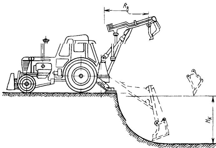
Рис. 15.2. Экскаватор Э-153А
