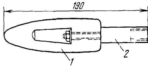
Рис 44 Наконечник для винтовых палок 1 — дерево или сталь 2 — стальная труба
