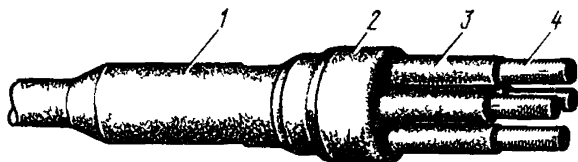
Рис 1048 Стационарная разветвительная свинцовая муфта
