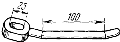
Рис 45 Ключ палочный
