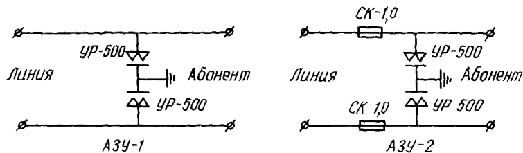
Рис 14 32 Принципиальные схемы абонентских защитных устройств
