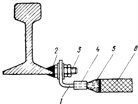
Рис 1418 Подключение дренажного кабеля к рельсу трамвая
