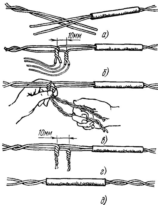
Рис. 10.19. Процесс парной скрутки жил с изолированием общей гильзой: а — надевание гильзы; б — одновременная скрутка обеих жил в изоляции и удаление последней с концов жил; в — одновременная скрутка оголенных концов жил; г — обрезка излишних концов жил; д — продвижение общей гильзы
