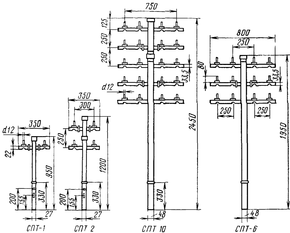
Рис. 8.1. Стоечные опоры
