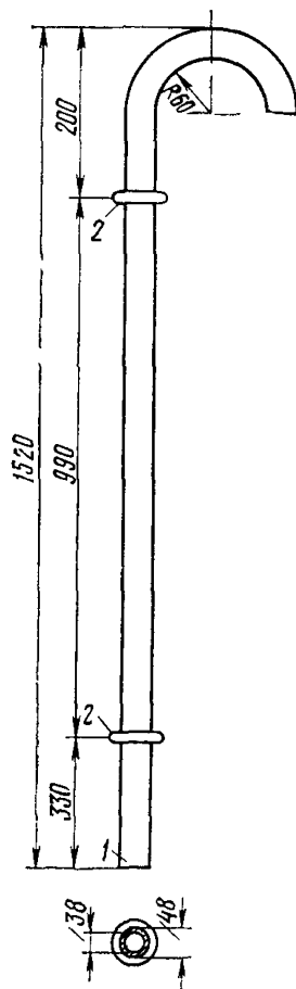
Рис. 8.3. Выводная труба:
