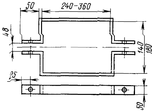
Рис. 7 19 Двухушковый хомут
