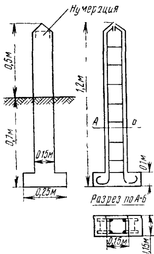
Рис 56 Железобетонный замерный столбик
