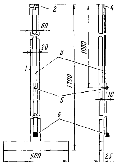
Рис. 36. Уклономер для кабельной канализации
