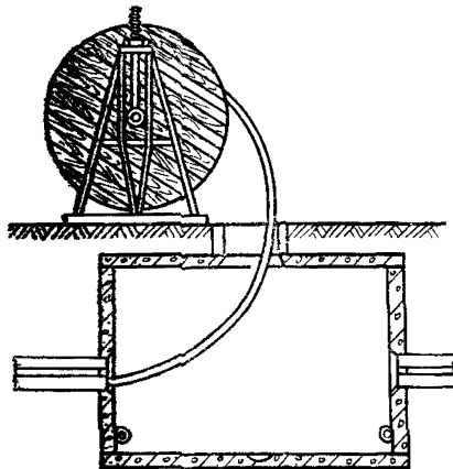
Рис. 4.11. Подача кабеля в смотровое устройство
