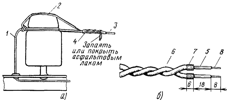
Рис. 7.29. Соединение клемм кабельного ящика с линейными проводами:
