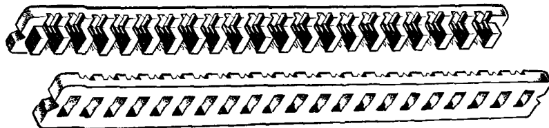
Рис. 10.29. Групповой десятипарный соединитель (модуль) СМЖ-10
