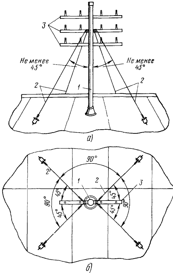
Рис. 8.8. Расположение оттяжек стойки: а — вид спереди: 1 — вертикальная труба стойки, 2 — оттяжки; 3 — траверсы. б — вид сверху
