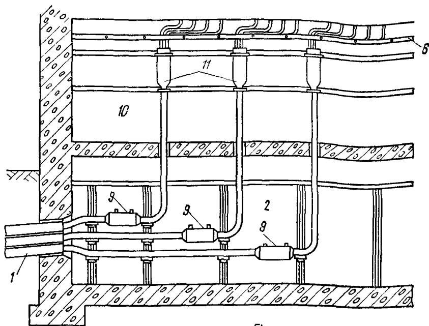
Рис. 371. Кабельные шахты:
