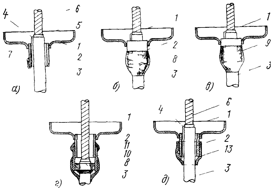
Рис 10 58 Ввод кабеля в распределительную коробку 10×2
