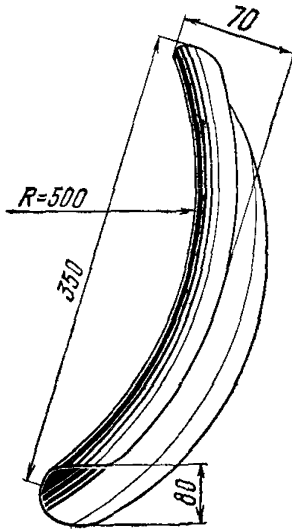
Рис. 4.15. Колено стальное кабельное
