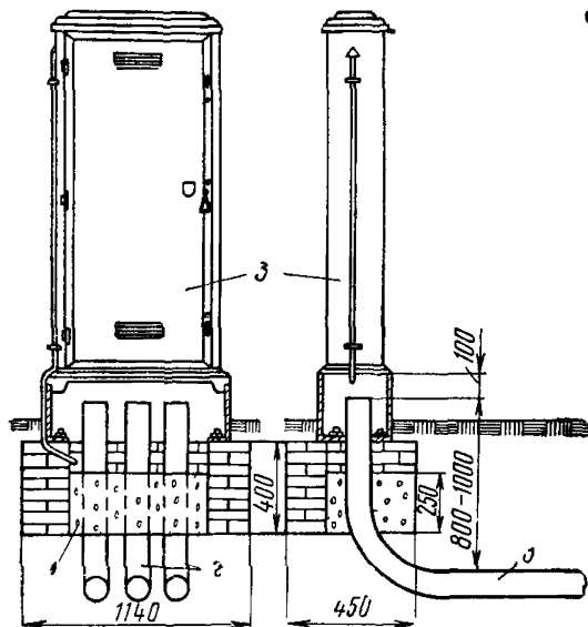
Рис 377. Установка распределительного шкафа на выложенном на месте фундаменте 1 — фундамент; 2 — изогнутые трубы; 3 — шкаф
