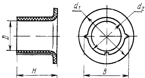
Рис. 9 21 Оконцеватель пластмассовый для труб (втулка полиэтиленовая)
