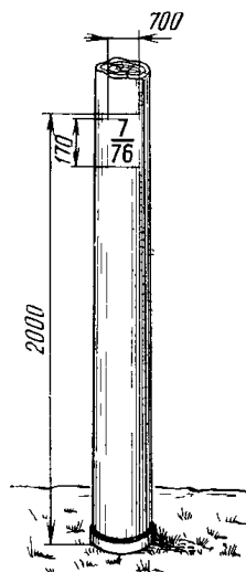
Рис. 7.26. Нумерация опор
