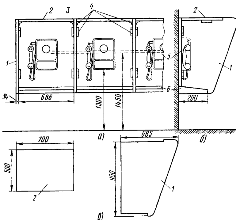
Рис. 13.10. Установка таксофонов на стенах вестибюлей:
