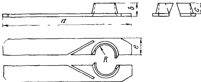
Рис. 10 36. Медные вкладыши для сварки поливинилхлорида
