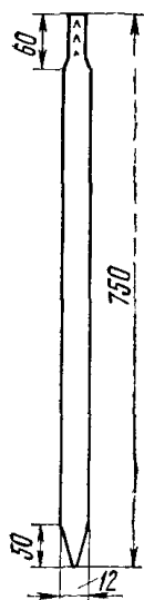
Рис. 8.2. Стальной штырь
