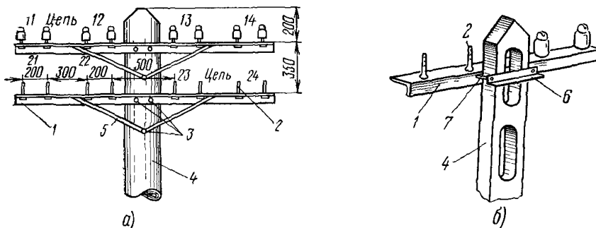
Рис. 7.9. Оснастка опор траверсами: а — деревянных; б — железобетонных:
