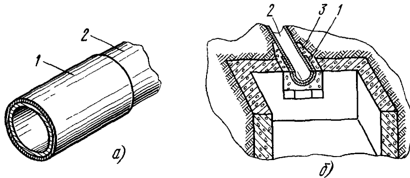
Рис. 332. Ввод полиэтиленовых труб в колодец а — подготовка конца трубы; б — заделка концов труб на вводе в колодец 1 — пять-шесть слоев битуминизированной ленты, 2 — полиэтиленовая труба, 3 — раствор цемента со щебенкой
