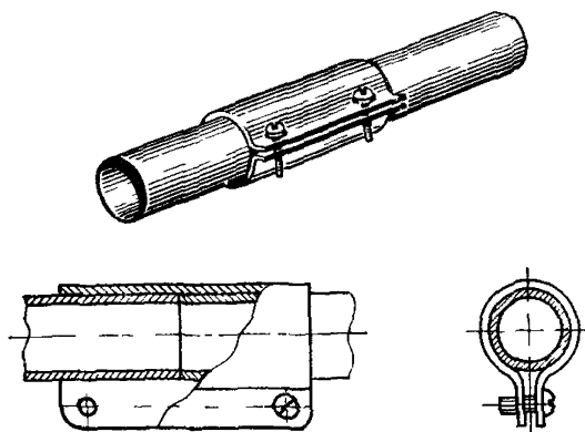
Рис. 9 23 Соединение тонкостенных стальных труб манжетой зажимаемой винтами
