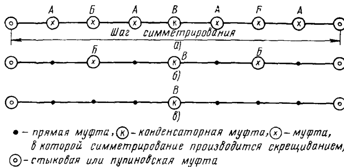
Рис. 11.1. Схемы симметрирования внутри шага
