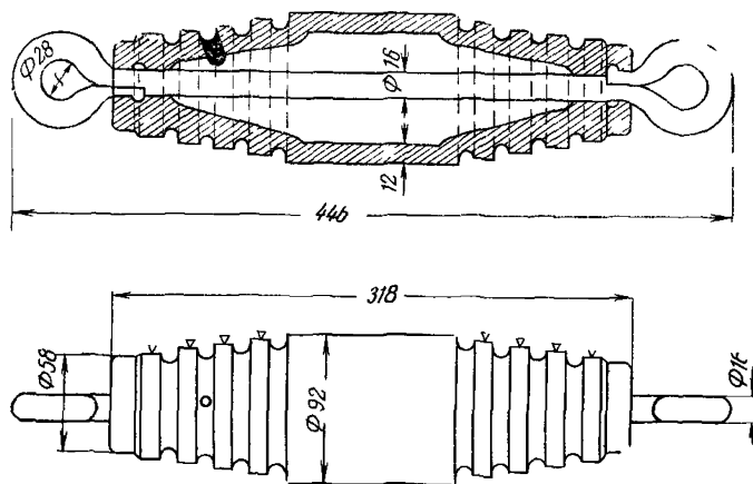
Рис 48 Цилиндр пробный
