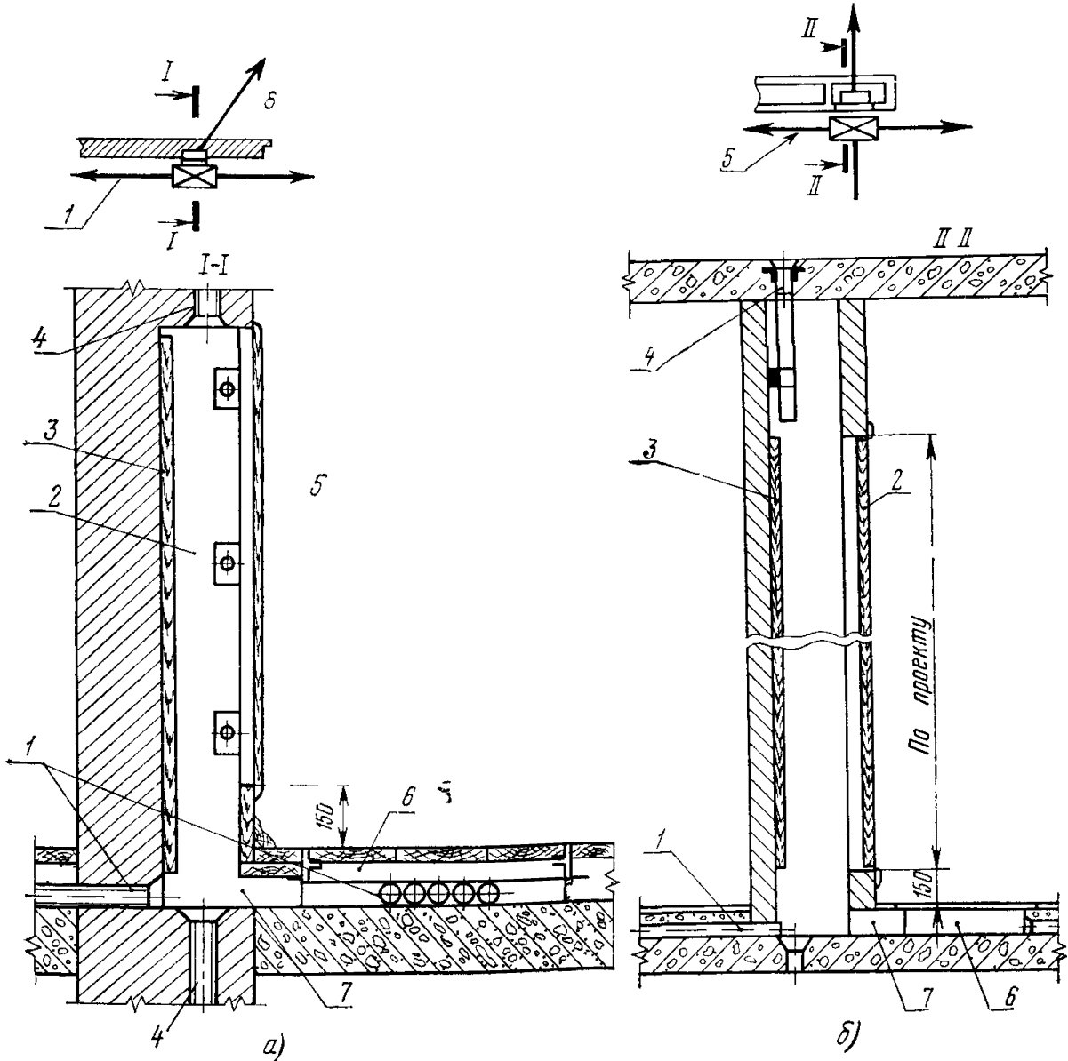
Рис. 9 36 Узел вертикального стояка
