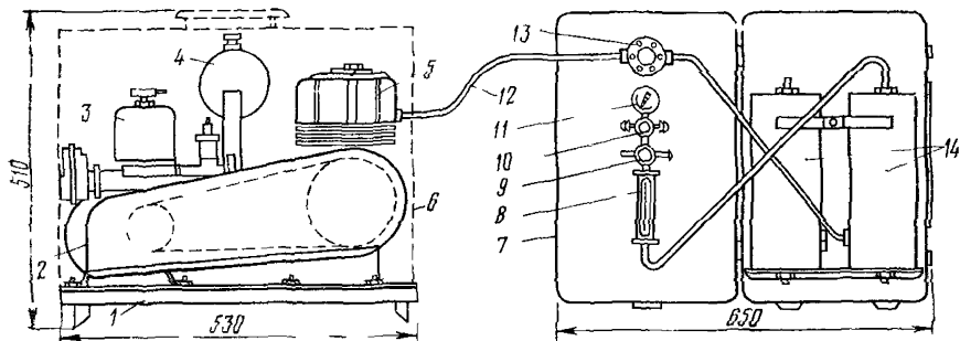
Рис. 12 11. Полевая нагнетательно осушительная установка типа ПНОУ-3
