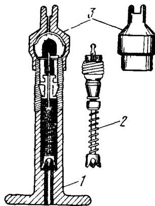
Рис. 12.14. Вентиль автомобильный типа Р:
