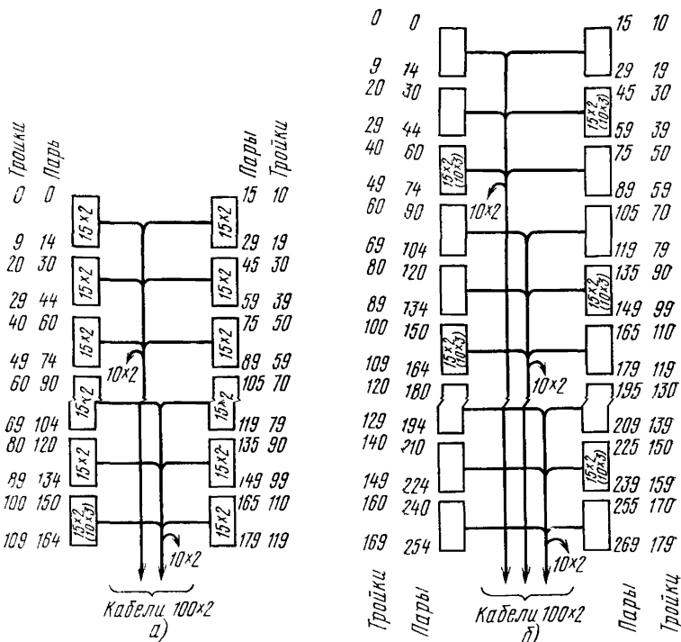
Рис. 1071. Схемы расшивки кабелей 100 \times 2 на рамки 15 \times 2 ( 10 \times 3 ) креста соединительных линий: а — на кроссе полуторной высоты; б — на кроссе двойной высоты
