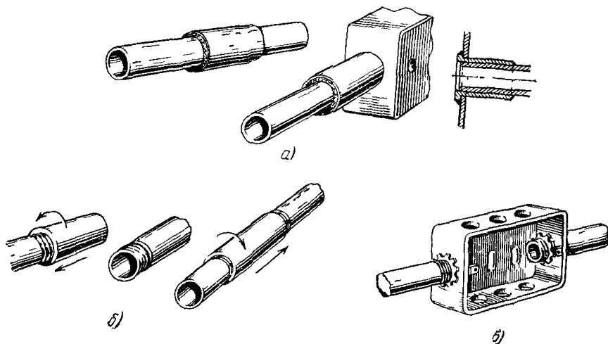
Рис. 9.24 Соединение тонкостенных стальных труб а — сваркой, б — резьбой; в — при помощи цапающих гаек
