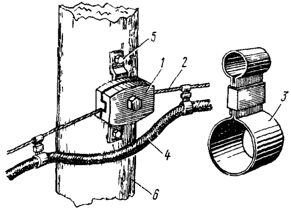
Рис. 7.39. Чугунная столбовая консоль и стальная подвеса для подвески кабеля:
