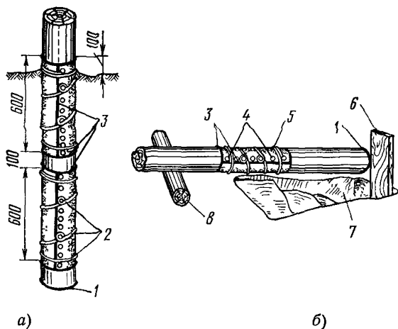
Рис. 7.14. Пропитка опор бандажным способом:
