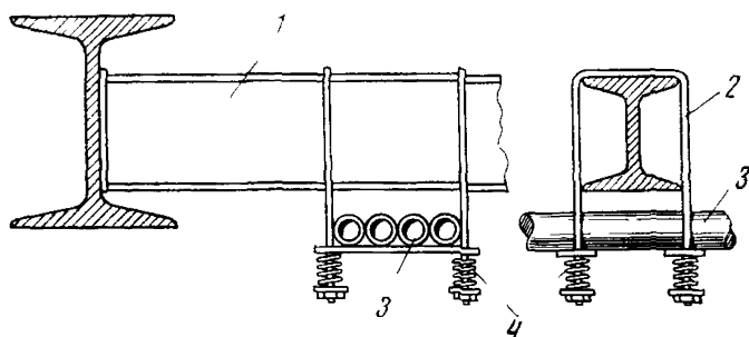
Рис 3 35. Прокладка трубопровода по мосту на пружинных амортизаторах:
