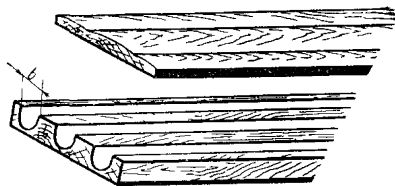
Рис. 9.17. Багет 3×6
