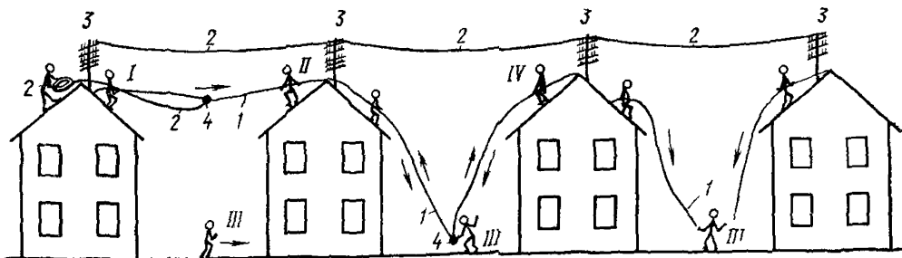
Рис. 8.16. Подвеска проводов на стоечных линиях:
