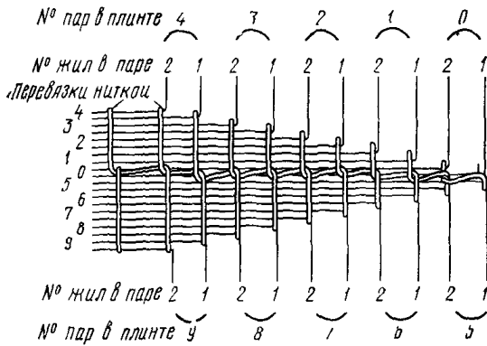
Рис. 10.67. Схема расшивки жил на плинт бокса
