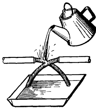
Рис. 10.14. Прощпарка сердечника кабеля
