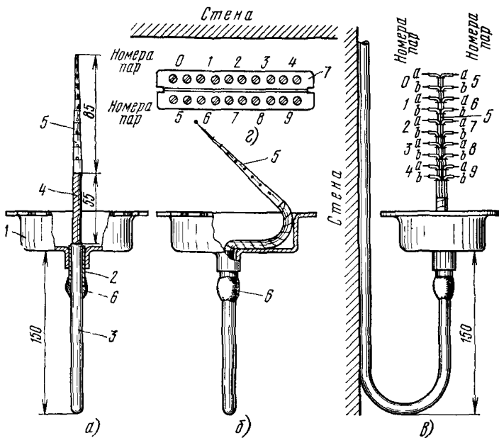
Рис 10 61 Примерные размеры разделки кабеля и порядок включения жил в штифты плинта распределительной коробки 10x2 КРТ, КРТП
