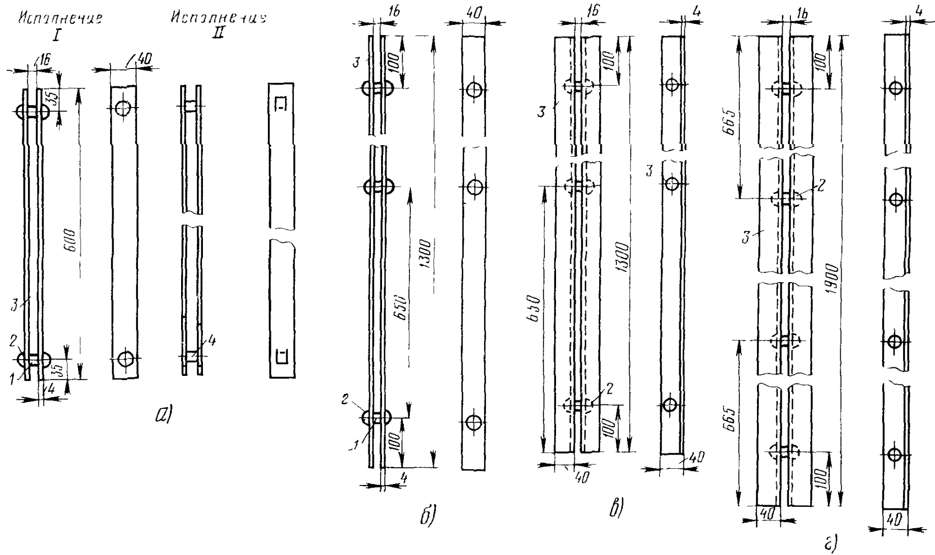
Рис 363. Кронштейны для кабельных консолей:
