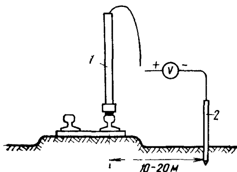
Рис. 14.11. Схема измерения потенциалов рельс электрифицированного транспорта относительно земли: 1 — деревянная штанга со стальным накопителем, 2 — стальной электрод
