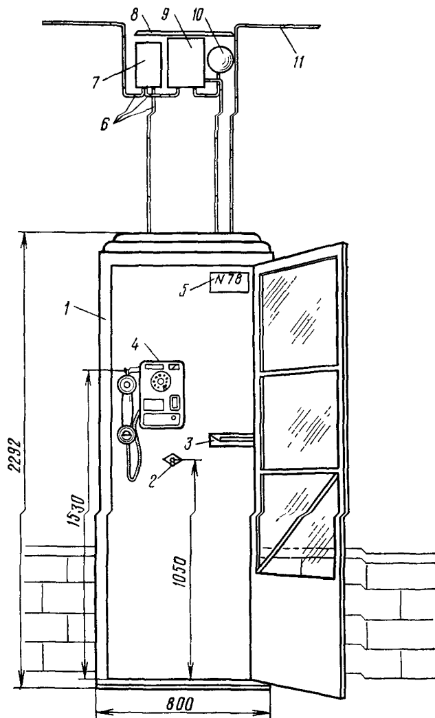
Рис. 138. Оборудование пункта таксофона в уличной кабине:
