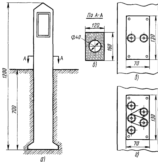
Рис. 14.1. Контрольно-измерительный пункт (КИП)
