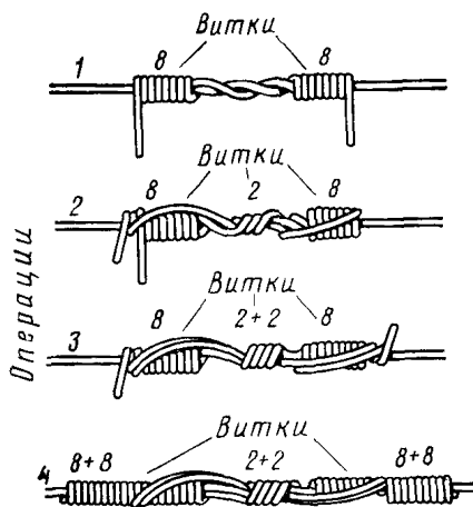
Рис. 7.35 Сращивание проводов двойной скруткой
