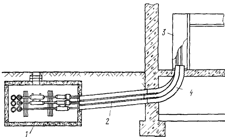
Рис. 373. Ввод кабелей с распайкой в стационарном колодце:
