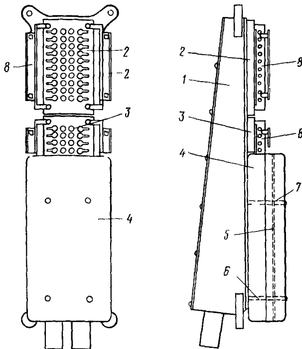
Рис. 11.5. Бокс БМ-2-3 с симметрирующей панелью:
