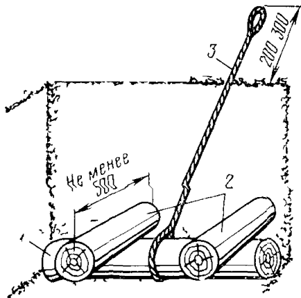
Рис 7 21. Крепление якоря двумя лежнями
