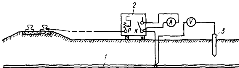
Рис. 14.14. Схема пробного включения дренажа на бронированном кабеле:
