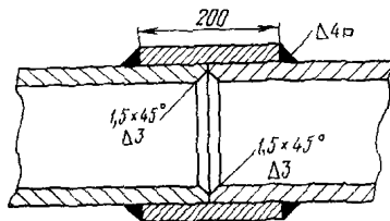
Рис. 6.3. Соединение стальных труб сваркой
