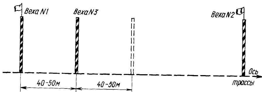
Рис. 2.2. Разбивка трассы с помощью вех
