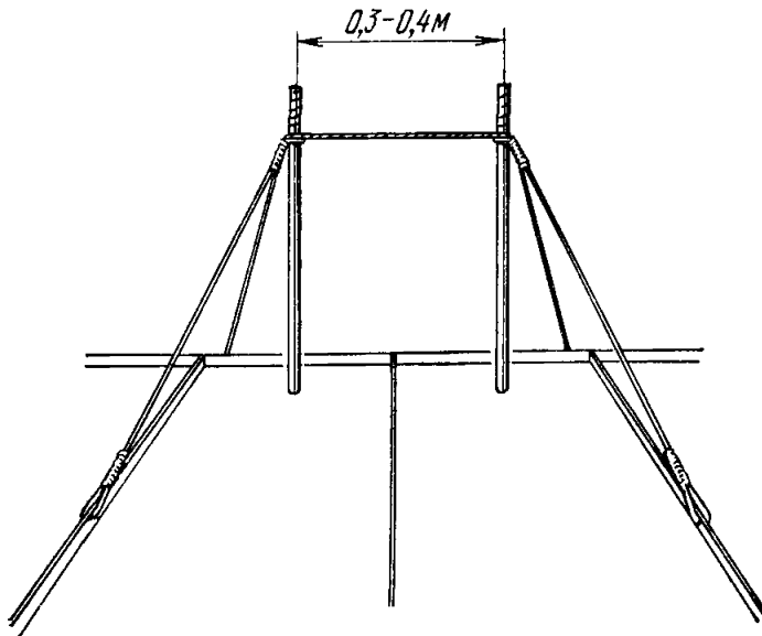
Рис. 8.10. Установка пары штырей
