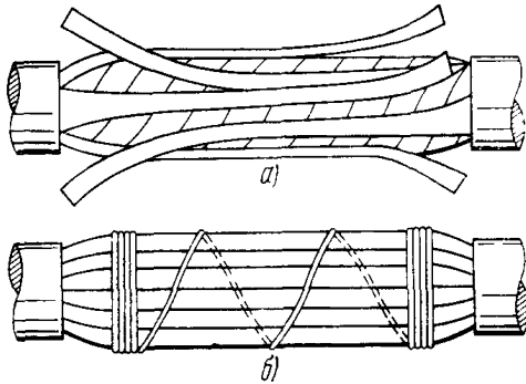
Рис. 10.31. Восстановление продольного экрана:
