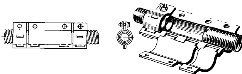
Рис. 9.33 Муфты-коробки типа КБ
