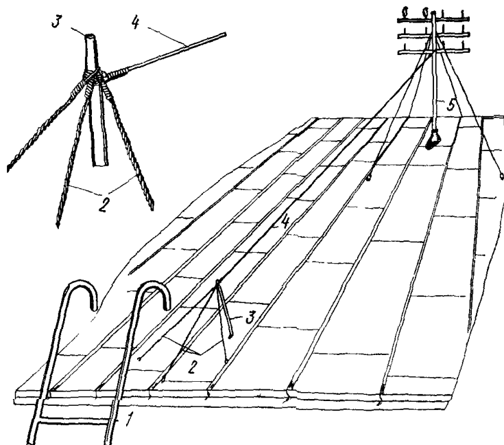
Рис. 8.15. Крепление предохранительной проволоки за стальной штырь:
