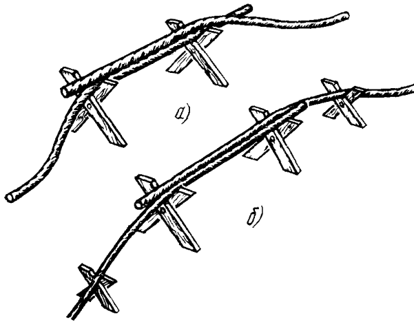
Рис 107 Укладка бронированных кабелей на козлы для монтажа муфт а — укладка кабелей с ленточной броней на одинарные козлы; б — укладка кабелей с проволочной броней на двоянные козлы
