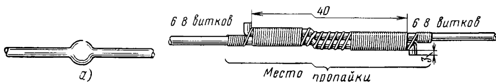
Рис. 736 Сращивание стальных проводов диаметром 3 мм: а — сваркой термитным патроном, б — спаянной проволокой с пропайкой
