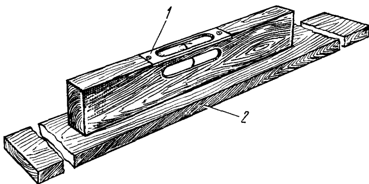
Рис 35. Рейка с уровнем для определения уклона трубопровода.
