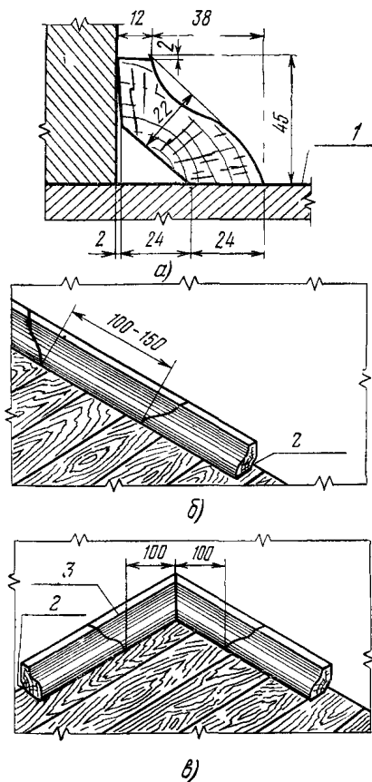
Рис. 9.15. Галтель с каналами скрытой проводки:
