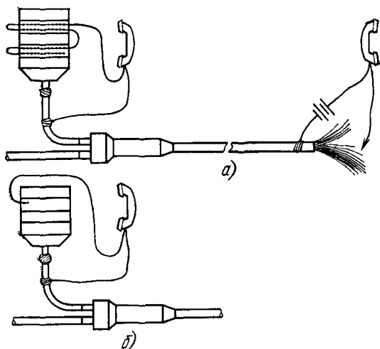
Рис. 10.52. Схема прозвонки кабеля в сборной муфте:
