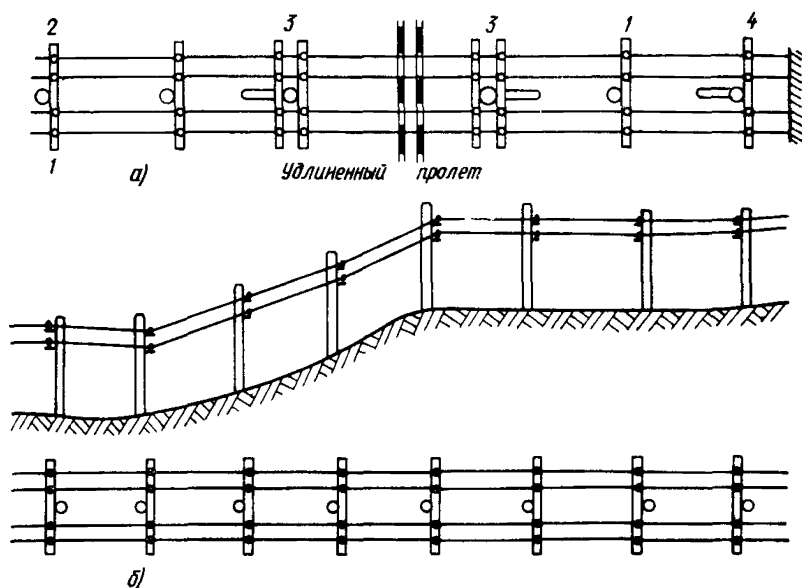
Рис. 7.10 Расположение траверс на опорах:
