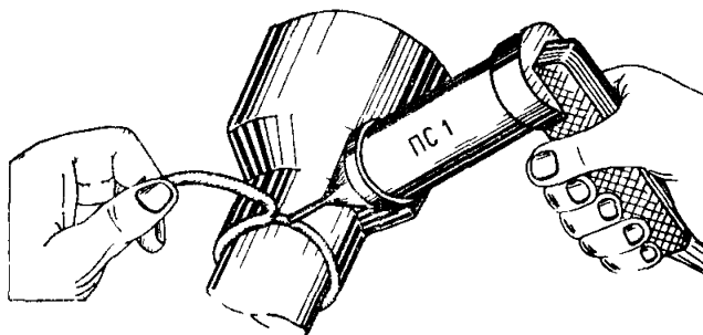
Рис 10.37 Сварка пластмассовых муфт при садочным пластмассовым прутком
