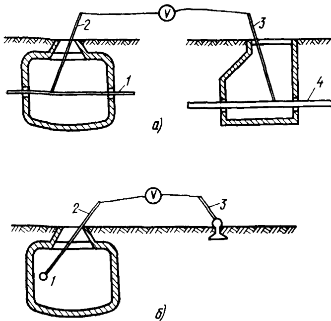
Рис. 14.10. Схема измерения разности потенциалов: а — между кабелем и трубопроводом в колодцах; б — между оболочкой кабеля и рельсами электрифицированного транспорта: 1 — кабель; 2 — штанга со свинцовым электродом; 3 — штанга со стальным электродом, 4 — трубопровод
