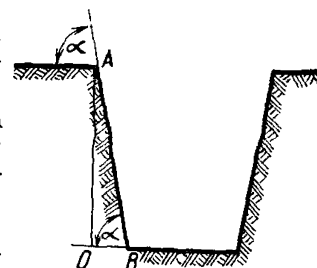
Рис. 29. Крутизна от-косов: \alpha — угол отко-са; \text{tg } \alpha = \frac{OB}{QA} — кру-тизна откоса
