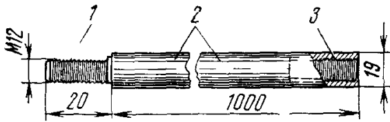
Рис 43 Палка винтовая 1 — резьбовой наконечник 2 — труба 3 — резьбовая втулка
