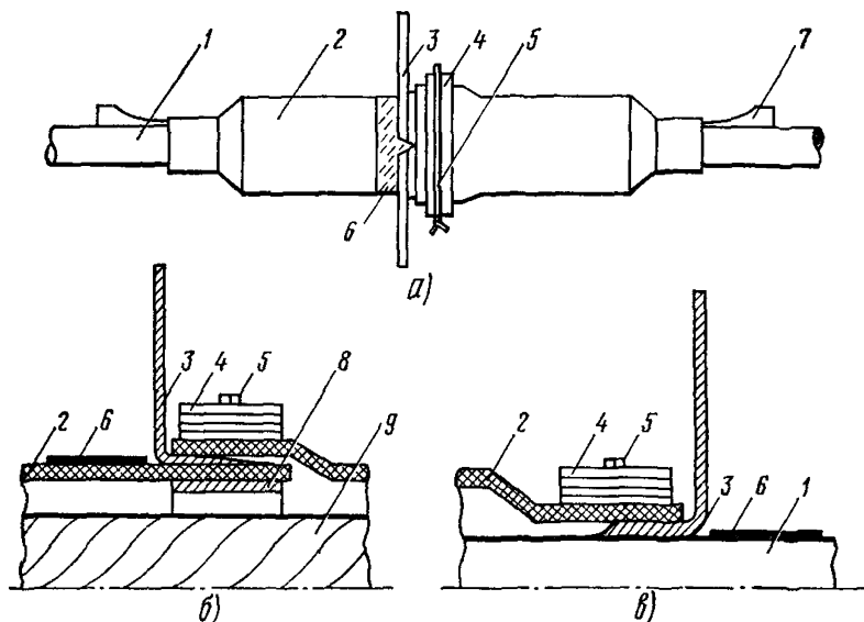
Рис. 10.34. Сварка полиэтиленовых муфт при помощи медных вкладышей:
