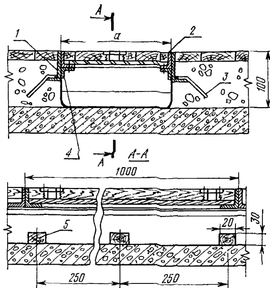
Рис 9 40 Подпольные каналы из металлических коробов со съёмными крышками
