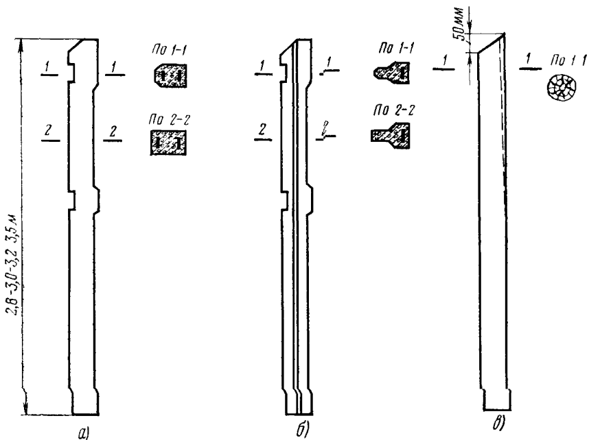
Рис 7.2. Приставки: а, б — железобетонные типов [Р и ТН; в — деревянная
