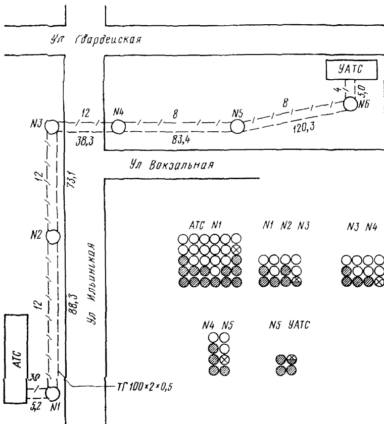
Рис 41 Рабочий чертеж на прокладку кабеля в канализации
