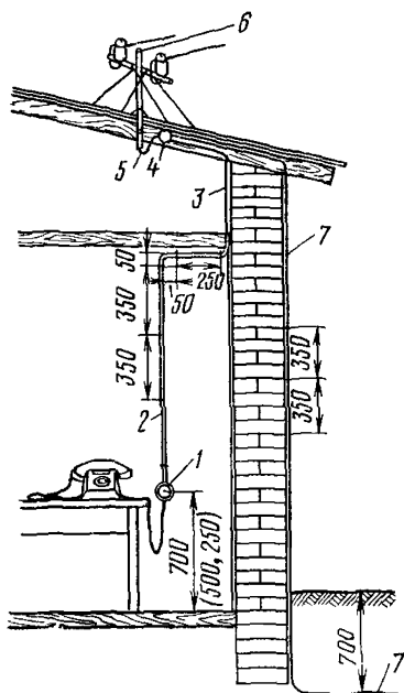
Рис. 136. Абонентский пункт с воздушным вводом:
