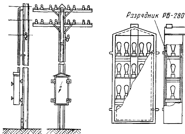
Рис. 14 30. Установка разрядников на опоре в специальных ящиках
