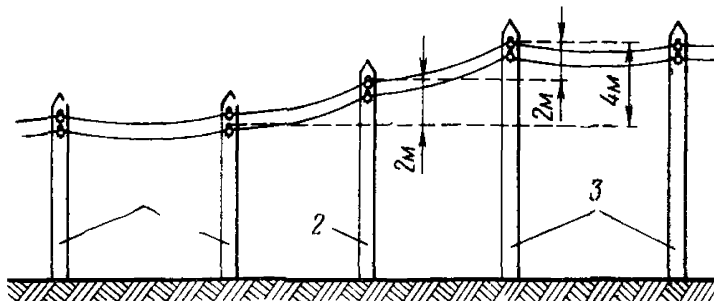
Рис. 7.3 Переход линии с нормальных на высокие опоры:
