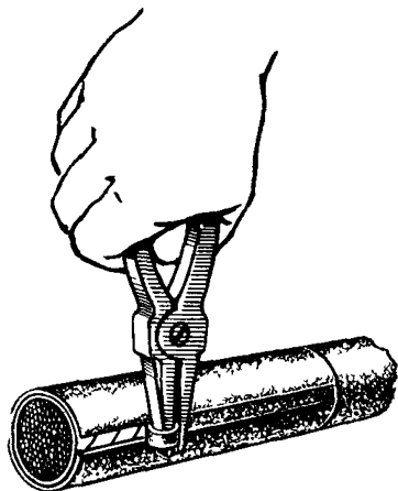
Рис. 10.10. Удаление полоски между надрезами
