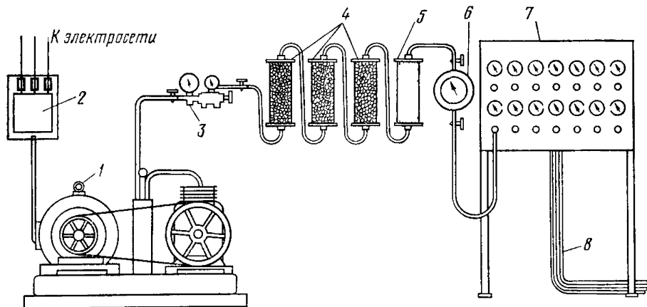
Рис. 12.10. Стационарная компрессорная установка:
