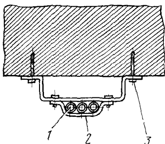
Рис 9 37 Узел крепления пакета труб
