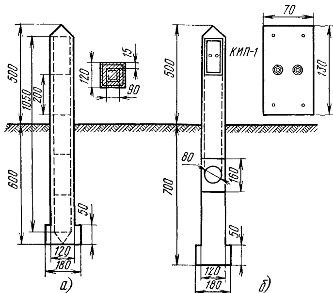
Рис. 10.42 Замерные железобетонные столбики: а — замерный столбик; б — замерный столбик, совмещенный с КИП
