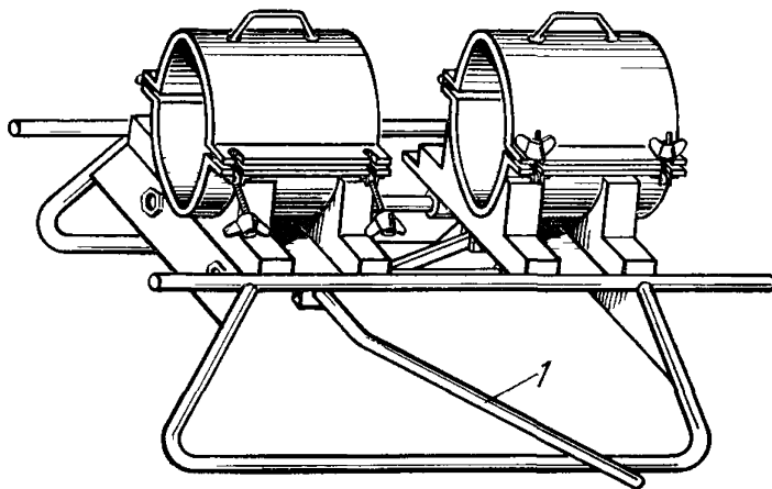
Рис 328 Станок для закрепления концов свариваемых труб 1 — рычаг
