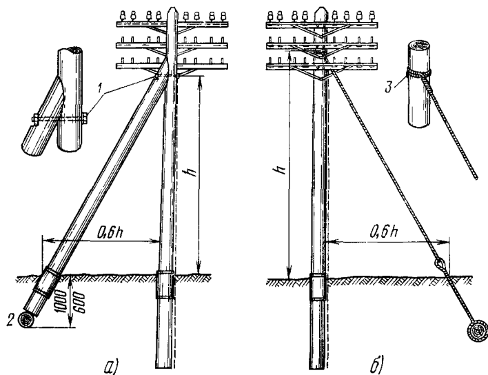
Рис 7.16 Укрепление опор: а — подпорой, б — оттяжкой:
