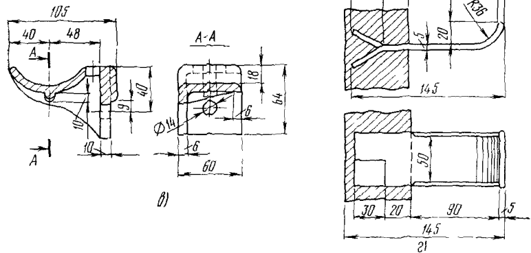
Рис. 362 Консоли кабельные и консольные крючья для смотровых устройств кабельной канализации. а — консоль кабельная чугунная трехместная; б — то же, двухместная; в — то же, одноместная; г — крюк консольный
