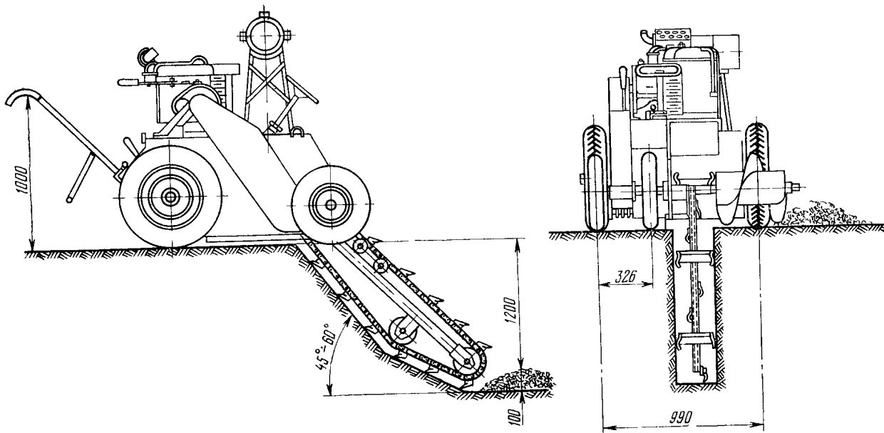
Рис. 15 4. Траншейный экскаватор ТК-2
