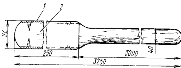
Рис 323 Контрольная штанга 1 — кровельная сталь, 2 — дерево
