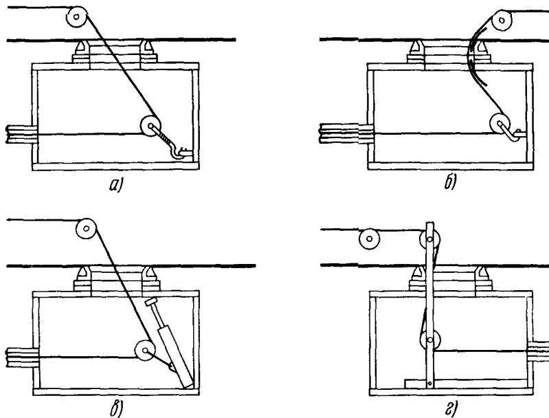
Рис 4.14. Приспособление для подтягивания троса из канала: а — серьга и блок; б — серьга, блок, колена и ролики; в — телескопическая стойка и блок; г — вертикальная блочная стойка
