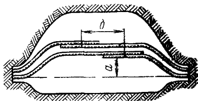
Рис 55 Выкладка концов кабелей в котловане
