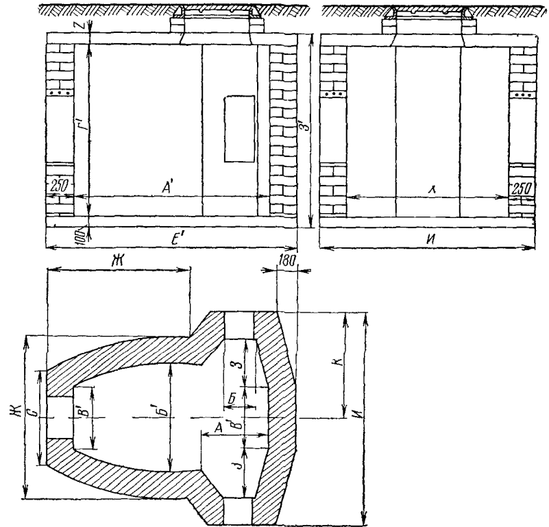
Рис 356 Разветвительные кирпичные колодцы типов ККСр 3, ККСр 4, ККСр 5
