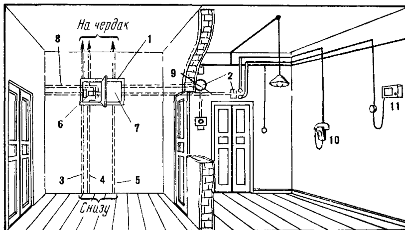
Рис. 9.14. Устройство телефонной сети в жилом доме способом смешанной проводки:
