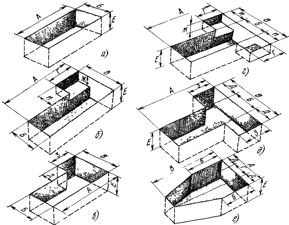
Рис 338 Примерные формы и размеры котлованов для основных типов колодцев кабельной канализации а — под проходные колодцы; б — под угловые колодцы, составленные из проходных и угловых вставок; в — под специально угловые колодцы, г — под разветвительные колодцы, составленные из проходных и угловых вставок, д — под специально разветвительные колодцы, е — под станционные колодцы
