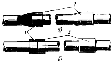
Рис. 3.34. Клеевые соединения поливинилхлоридных труб: а — раструбные; б — муфтовые; 1 — клей; 2 — раструбы; 3 — муфты
