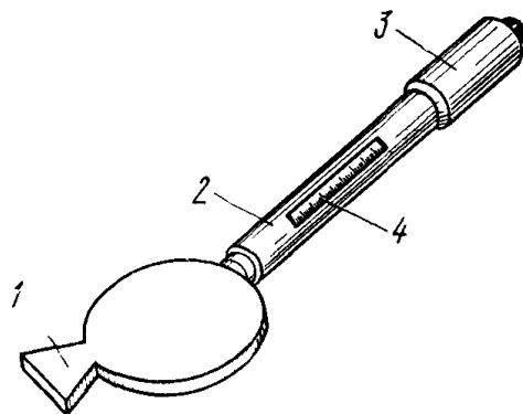
Рис. 330 Нагревательный диск 1 — выступ для нагрева диска пламенем паяльной лампы или газовой горелки, 2 — дюралевая трубка 3 — деревянная или пластмассовая рукоятка, 4 — электроконтактный термометр или термодатчик
