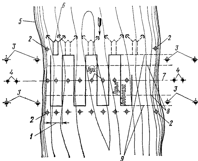
Рис. 65 Обследование и разбивка трассы подводного перехода:
