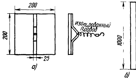
Рис. 14.5. Свинцовые электроды: а — пластинчатый; б — трубчатый
