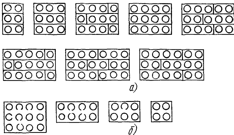
Рис. 3 25. Некоторые варианты компоновки блоков из бетонных труб:
