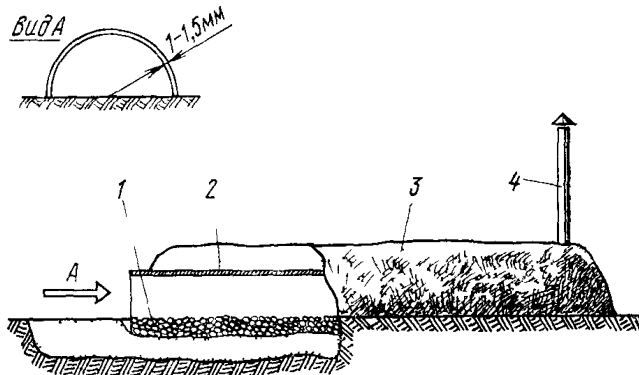
Рис 210 Схема установки коробов для отогрева грунта
