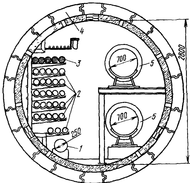
Рис 367 Поперечное сечение круглого коллектора диаметром 2800 мм
