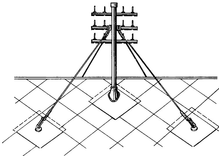
Рис. 8.12. Установка стоечных опор на неметаллических крышах
