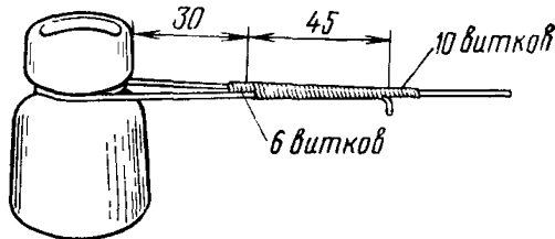
Рис. 7.31. Оконечная заделка стальных проводов диаметром 3 мм
