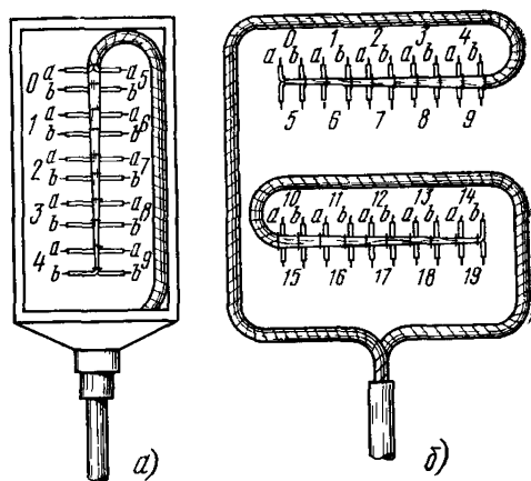
Рис. 10 62. Расшивка кабеля и порядок включения жил на плинты кабельных ящиков: а — 10×2; б — 20×2
