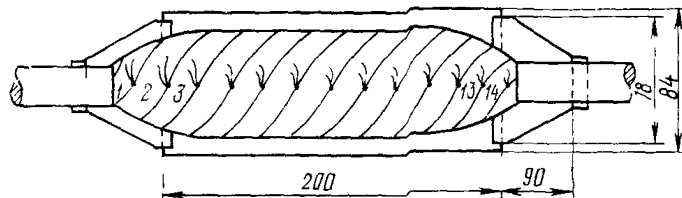
Рис. 112. Схема симметрирующей муфты (размеры даны для кабеля 7×4×1,2)
