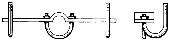
Рис. 8.18. Отходная планка
