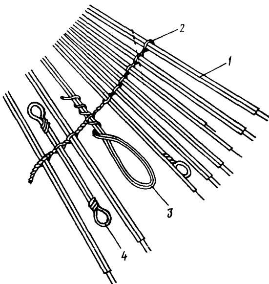
Рис 10.53 Перевязка отобранных (занумерованных) пар в косоплетке:
