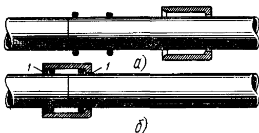
Рис. 3.18. Способ с применением специальных асбестоцементных муфт и резиновых колец: а — надвигание специальной асбестоцементной муфты и резиновых колец; б — готовый стык:
