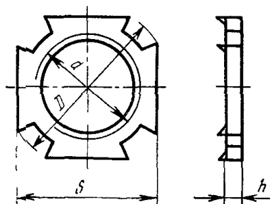
Рис. 9.26. Гайка установочная заземляющая (царапающая)
