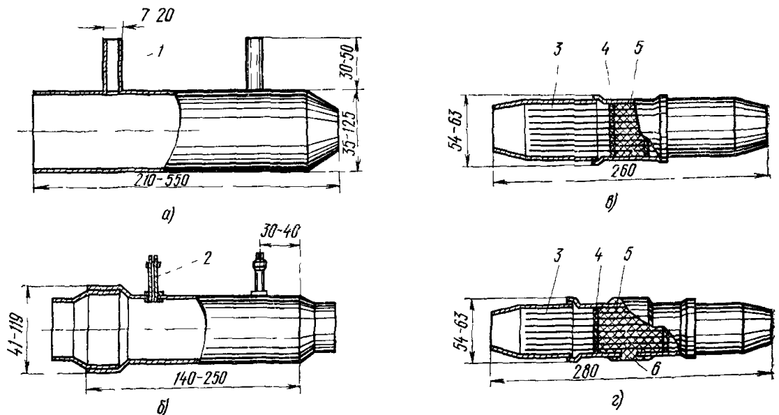
Рис. 12.17. Газонепроницаемые муфты: а — свинцовая типа МГ; б — полиэтиленовая; в — свинцовая типа ГМС; г — свинцовая типа ГМСИ: 1 — патрубок (трубка); 2 — вентиль; 3 — медные жилы; 4 — эбонитовая шайба; 5 — эпоксидный компаунд; б — кольцевой вырез
