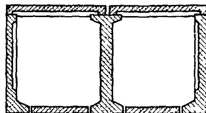
Рис 368 Схематическое изображение поперечного сечения двухсекционного коллектора
