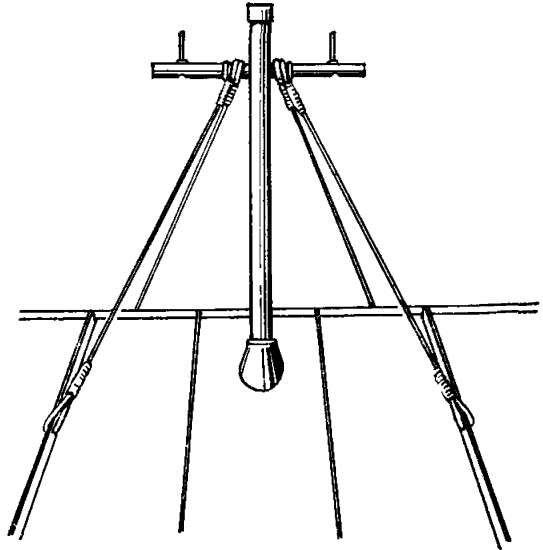
Рис. 8.9. Установка стойки типа СПТ-1
