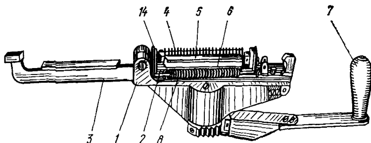
Рис. 10.30 Ручная пресс-техника ПСМЖ-200 для соединителей типа СМЖ-10:
