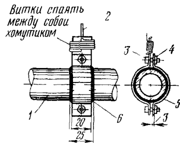
Рис 14 36 Подключение заземляющего провода к водопроводной трубе:
