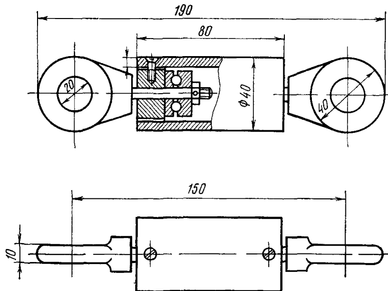
Рис 4 13 Компенсатор кручения
