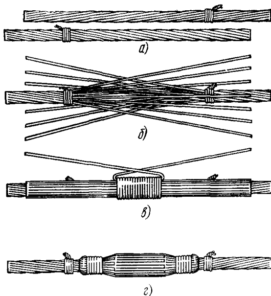
Рис. 10.47. Соединение стального каната бандажным способом:
