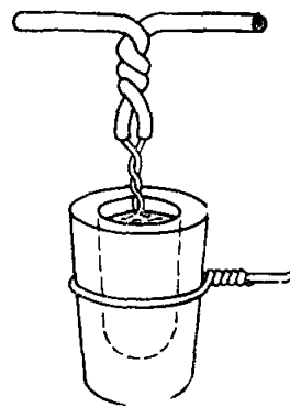
Рис. 10.22. Пропайка скрутки жил в стаканчиковом паяльнике
