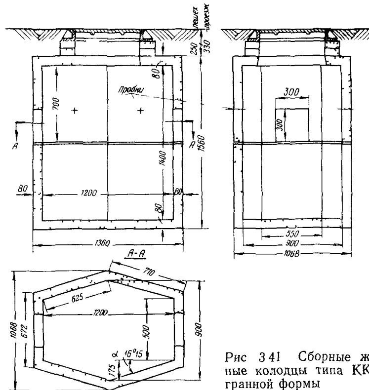
Рис 340 Сборные железобетонные колодцы типа ККС-1
