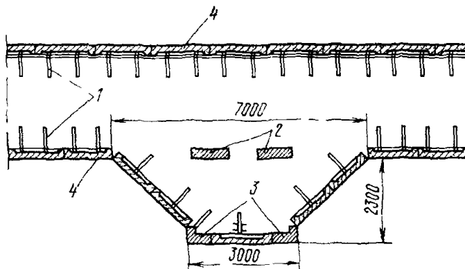
Рис. 370. Камера для ввода коммуникаций в коллектор
