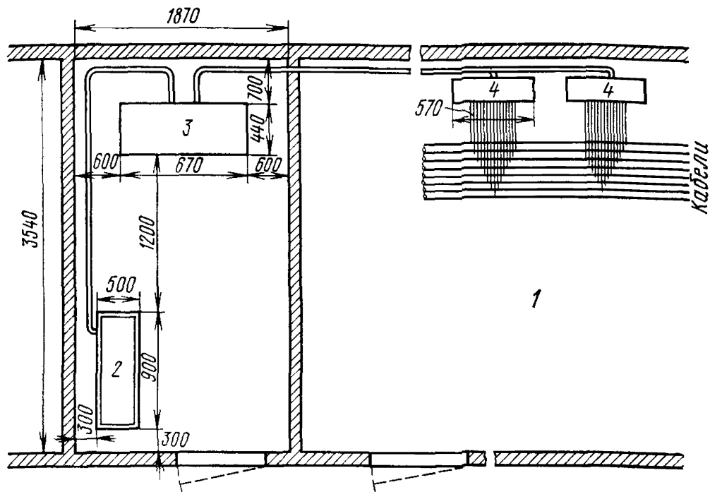
Рис. 12.3. Размещение КСУ на 30 или 60 кабелей: 1 — шахта; 2 — компрессорная группа; 3 — блок осушки и автоматики; 4 — распределительный стив
