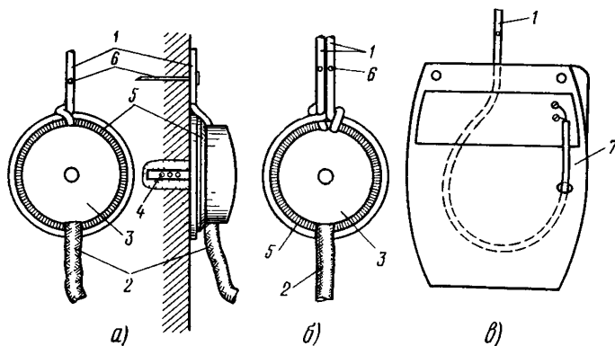
Рис. 13.3. Включение провода 1 \times 2 :
