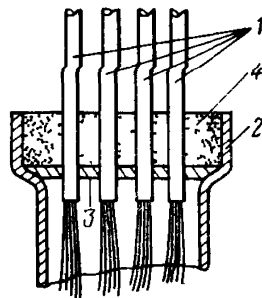
Рис 1049 Разветвительная стационарная муфта без патрубков
