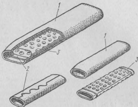
Рис. 10.23. Индивидуальный сжимаемый соединитель трубчатого тупикового типа:
