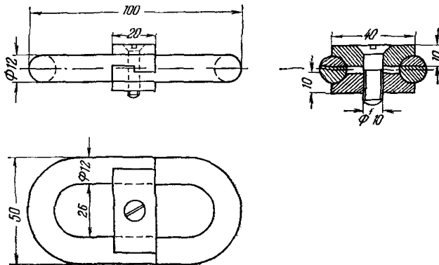
Рис. 4.10. Карабин
