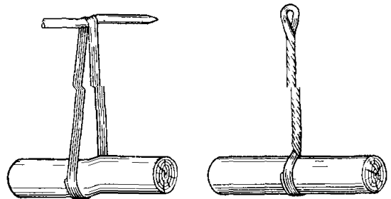
Рис. 7 22. Заделка якорного жгута
