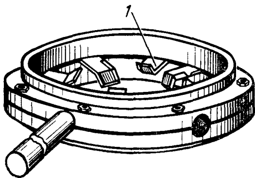
Рис. 329 Фреза с комбинированными резаками для торцовки и снятия фаски 1 — комбинированные резы
