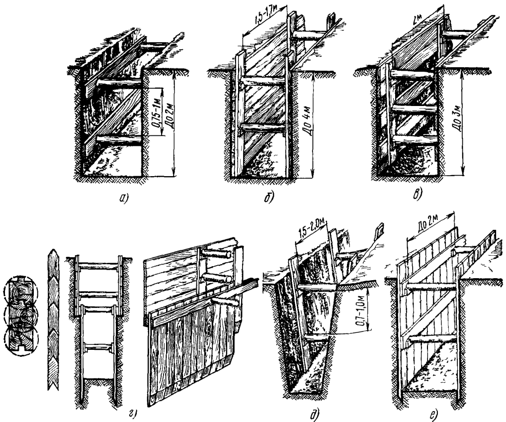
Рис. 2.11. Способы крепления стенок траншей и котлованов: а — горизонтально-рамный; б — горизонтально-сплошной; в — горизонтальный с прозорами; г — смешанный горизонтально-сплошной со шпунтом; д — вертикально-рамный; е — вертикально-сплошной
