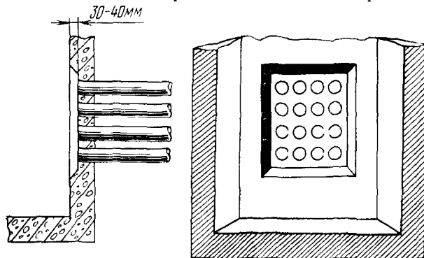
Рис. 3.10 Ввод труб в смотровые устройства
