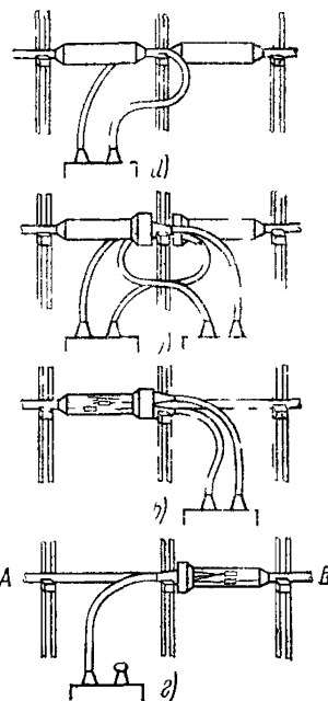
Рис. 10 51 Соединение пупиновских ящиков с линейными кабелями: а — соединительными муфтами; б — разветвительными муфтами с двумя патрубками (пальцами) каждая; в — разветвительной муфтой с тремя патрубками (пальцами); г — одним общим стабкабелем
