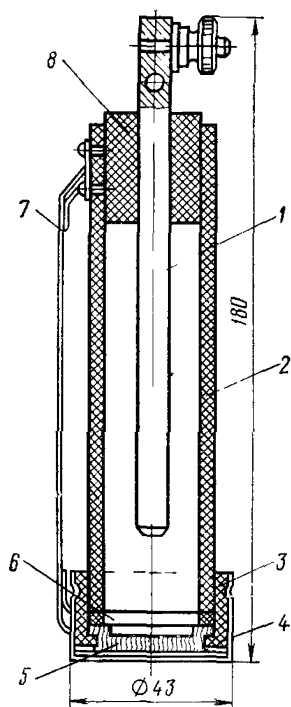
Рис 148 Медносульфатный неполяризующийся электрод:
