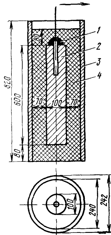
Рис 14 27. Неупакованный протектор МГА-5 из сплава МЛ-5
