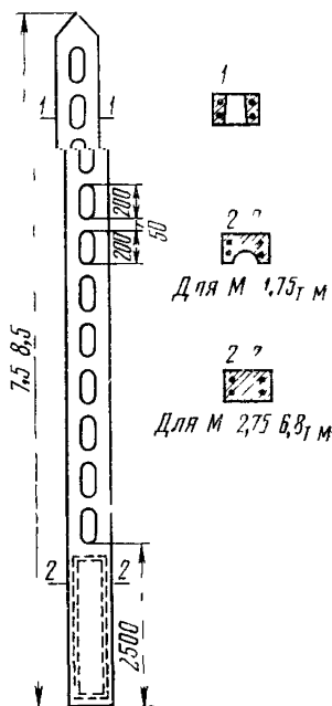
Рис 71 Железобетонная опора
