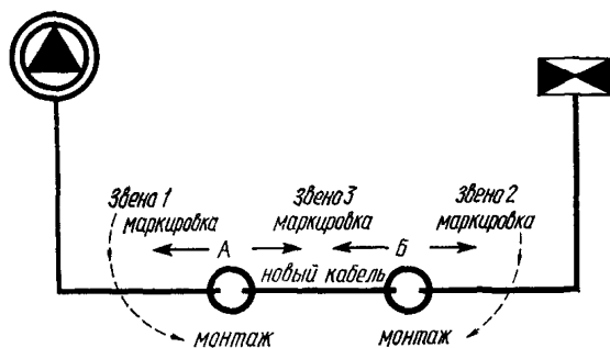
Рис. 10.54. Замена пролета тремя звеньями монтажников
