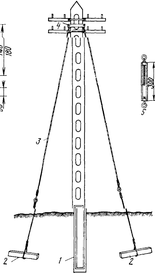
Рис. 7 20 Укрепление оконечной железобетонной опоры двумя оттяжками
