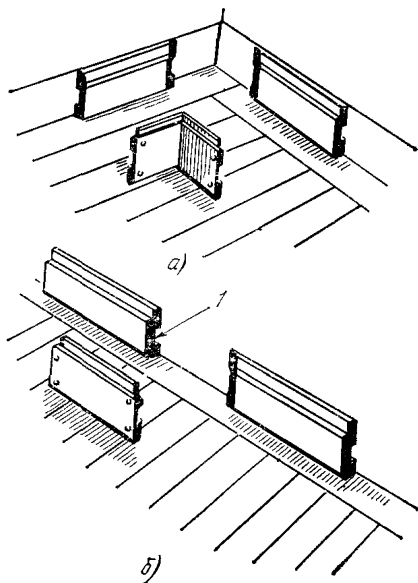
Рис. 9.16. Багет с каналом скрытой проводки:
