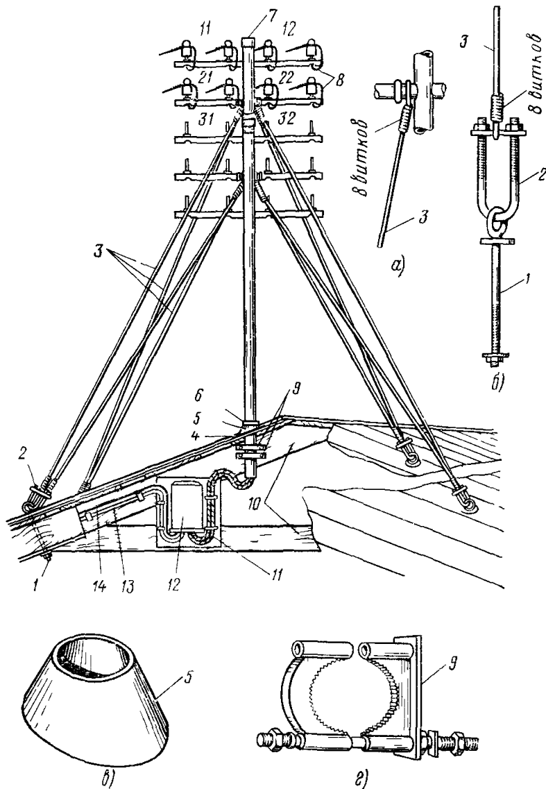
Рис. 84. Установка стойки 10×2 и детали ее крепления:
