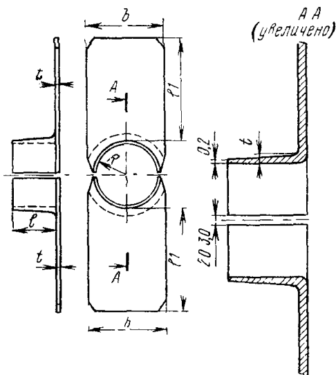
Рис. 10 33. Конструкция медных вкладышей для сварки полиэтилена
