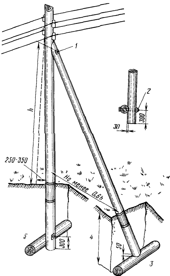
Рис. 7.17. Угловая опора, укрепленная подпорой и лежнем:
