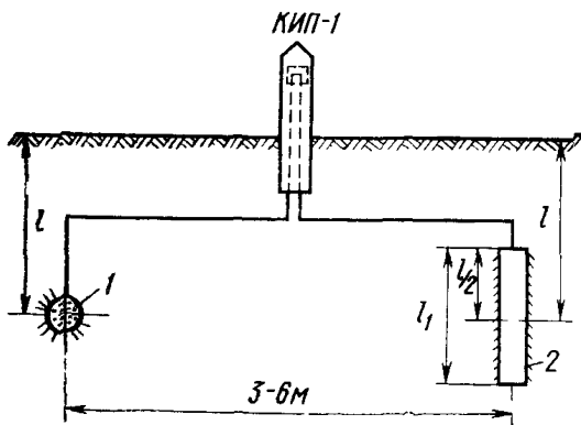
Рис. 14.28. Схема протекторной установки в грунте высокой влажности:
