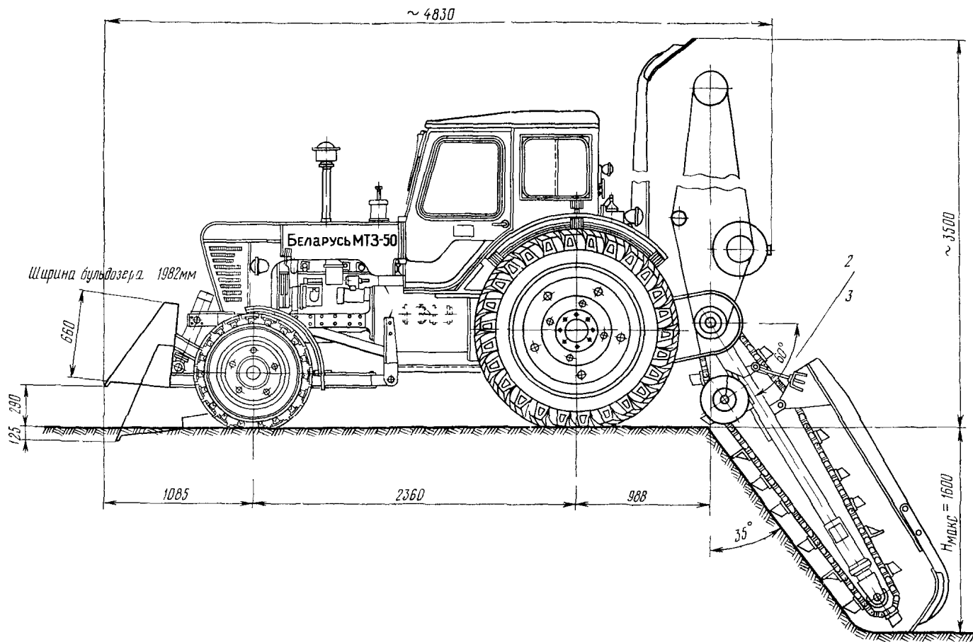
Рис 153 Цепной граншейный экскаватор ЭТЦ-161
