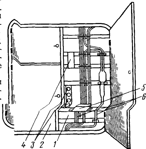
Рис. 9.41. Крепление кабелей к металлоконструкциям шкафов и ниш:
