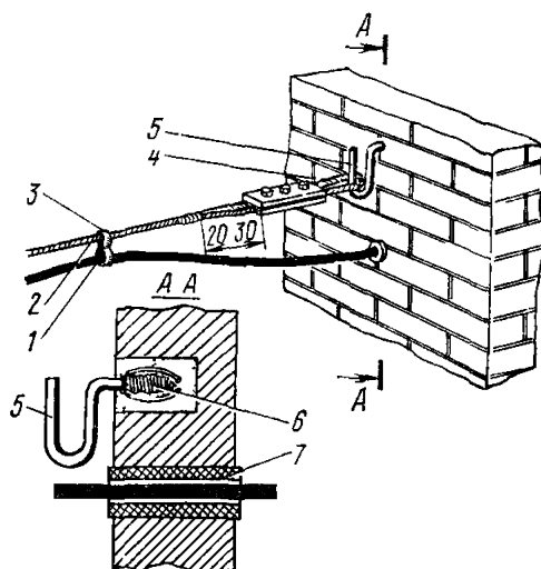
Рис 911 Ввод подвешеного кабеля в здание
