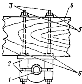
Рис 86 Крепление чугунного хомута
