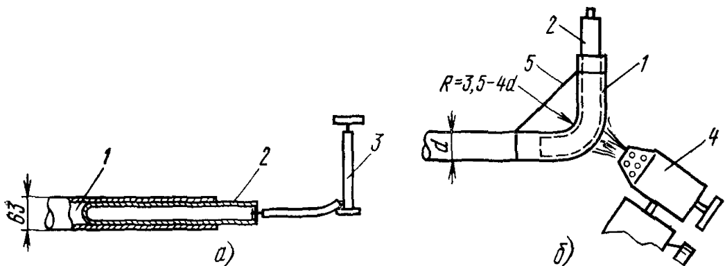
Рис 333 Изгибание полиэтиленовой трубы диаметром 63 мм для вывода на стены зданий а — раздув резинового шланга, б — разогрев изгибаемой трубы. 1 — полиэтиленовая труба, 2 — резиновый шланг, 3 — воздушный насос, 4 — паяльная лампа, 5 — вязка
