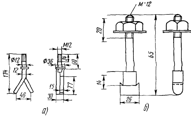
Рис 364 Детали крепления кронштейнов и консолей а — болт фундаментный (е р ш); б — болт консольный
