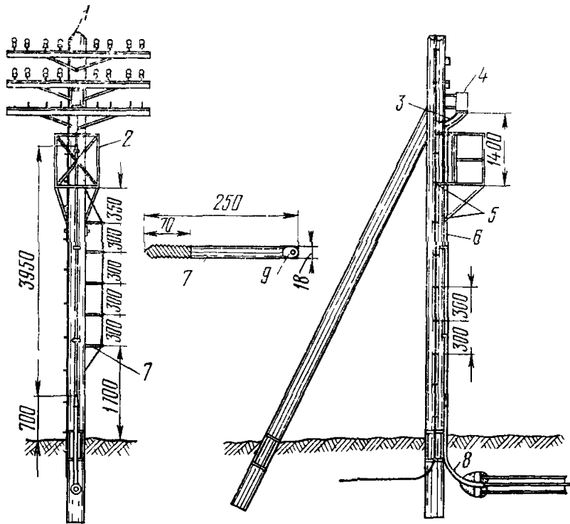
Рис. 7 27. Кабельная опора:
