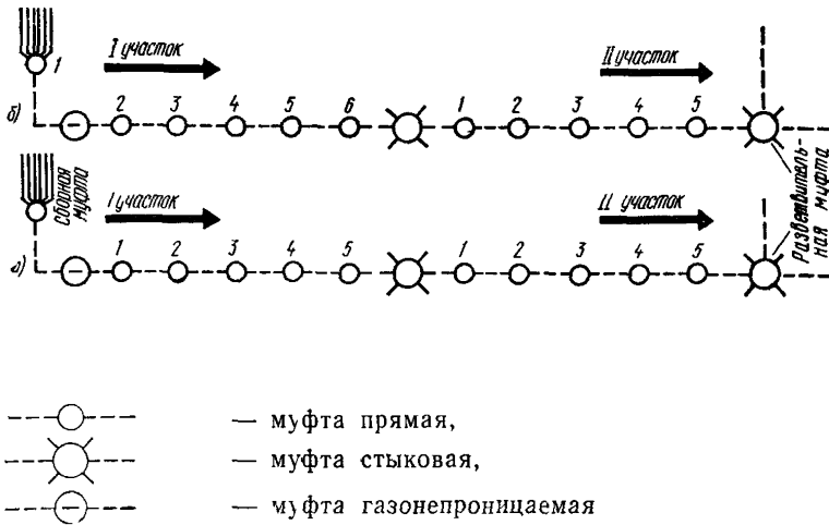
Рис 10.5 Последовательность монтажа муфт кабельных линий ГТС
