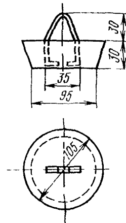
Рис. 3.7. Пробка для закупорки каналов кабельной канализации
