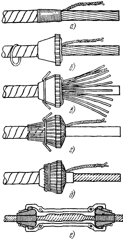
Рис. 10.44. Соединение круглых проволок брони при помощи стяжной муфты с грушевидными вкладышами а — припайка жгута из медных проволок; б — надвигание стального кольца и посадка вкладыша; в — фиксация вкладыша двумя проволоками брони; г — укладка всех проволок брони на вкладыше; д — огибание концами бронепроволок стального кольца и наложение бандаж из линейной проволоки диаметром 3 мм; е — установка корпуса муфты
