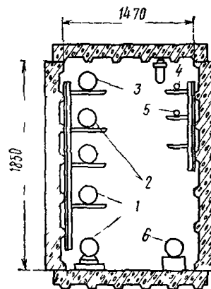
Рис 369 Поперечное сечение коллектора малого типа (сцепка)
