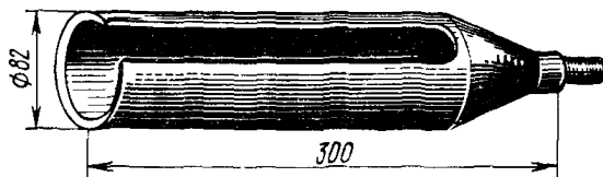
Рис 47 Совок для очистки засоренных каналов
