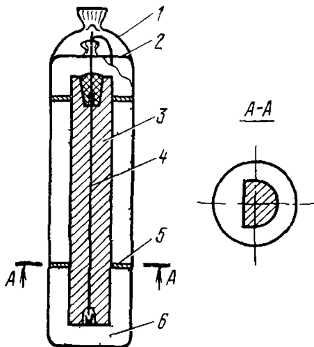
Рис 14 26 Протектор ПМ 10 У/2 МЛ16 в заводской упаковке
