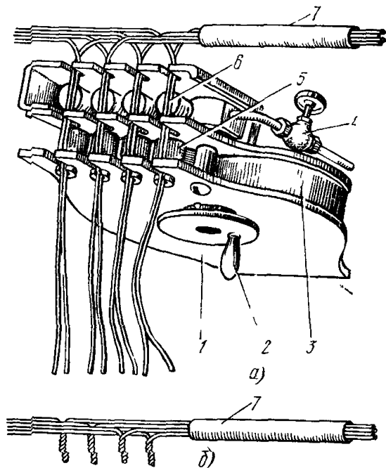
Рис. 10.20. Механизированная скрутка четверки жил с помощью приспособления ПСЖ-4: а — сращивание жил; б — готовые скрутки: 1 — корпус; 2 — рукоятка; 3 — большая шестерня; 4 — газовый кран; 5 — малые шестерни; 6 — место нагрева и скрутки жил; 7 — общая гильза
