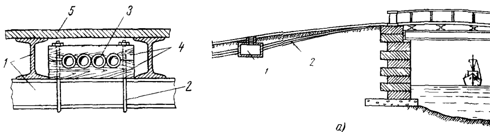
Рис 3 36 Прокладка трубопровода по мосту на деревянных колодках
