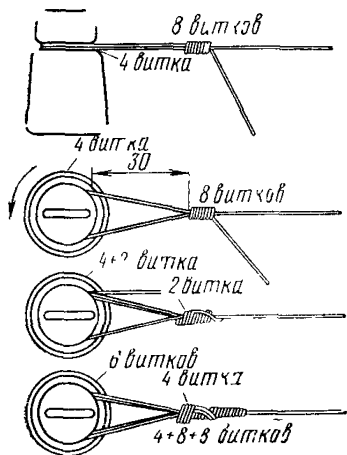
Рис. 7.30. Оконечная заделка провода диаметром 1,2—2 мм
