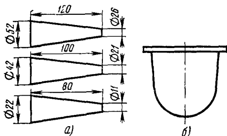
Рис. 9 19 Пробки для закупорки каналов
