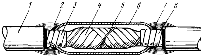
Рис. 1038. Восстановление стальной гофрированной оболочки свинцовой муфтой:
