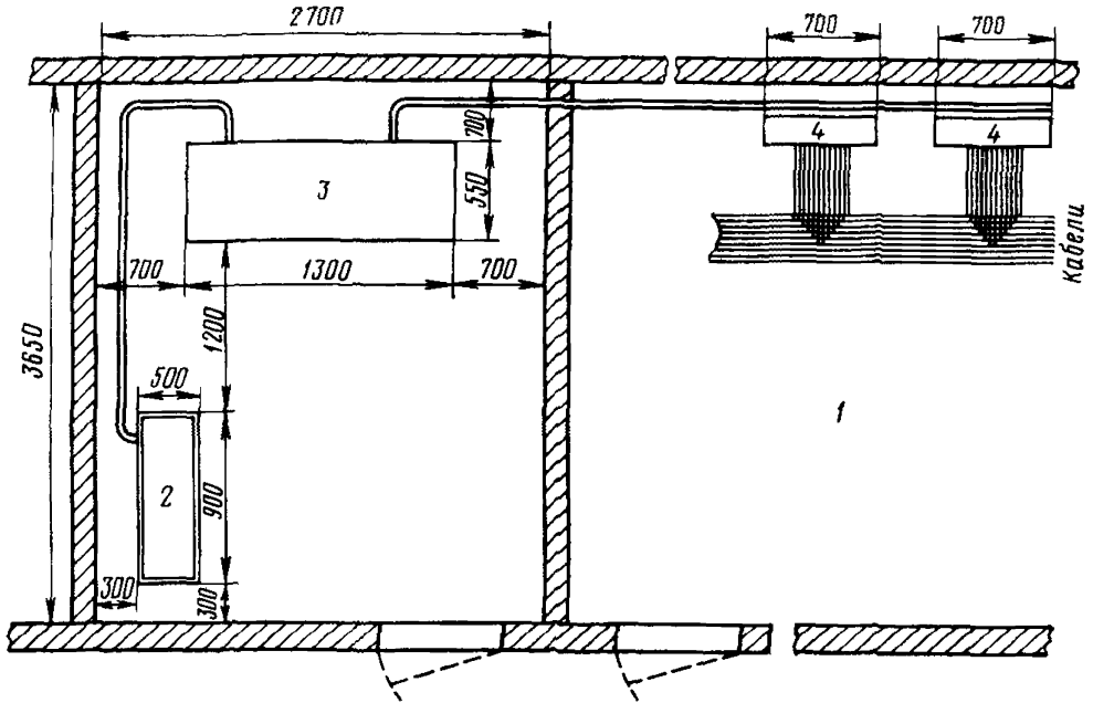
Рис. 12.7. Размещение КДВ-10 на 100 кабелей:
