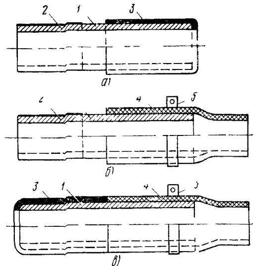
Рис. 1039. Конструкции переходных манжет:
