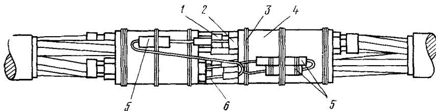
Рис 114. Сросток симметрирующей муфты кабеля 7×4
