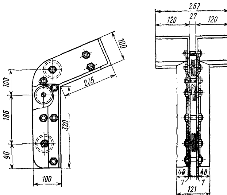
Рис. 4.16. Колено блочное
