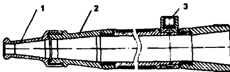
Рис. 2.1. Ствол-водомер:
