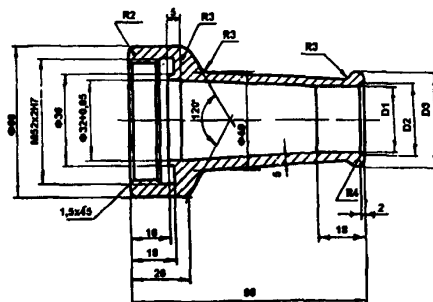
Рис. 2.1. Ствол-водомер:
