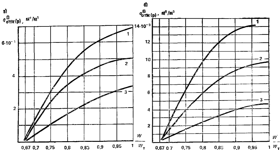
Рис. 15. Графики для определения объема воды, отжимаемой из супеси (а), суглилков и глин (б) под действием динамической нагрузки от автомобилей
