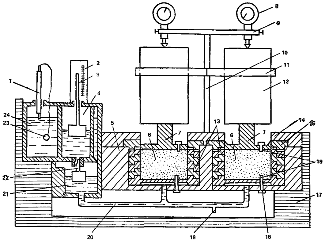
Рис. 1. Прибор для определения пучения и осадки грунта
