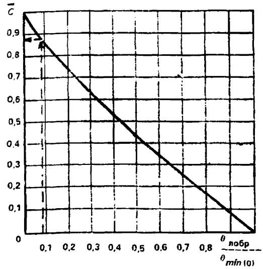
Рис. 8. Номограмма для определения параметра C , входящего в расчет глубины промерзания
