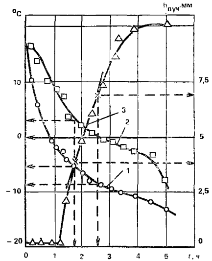
Рис. 2. Кривые пучения и температуры легкой пылевой супеси, полученные с помощью прибора
