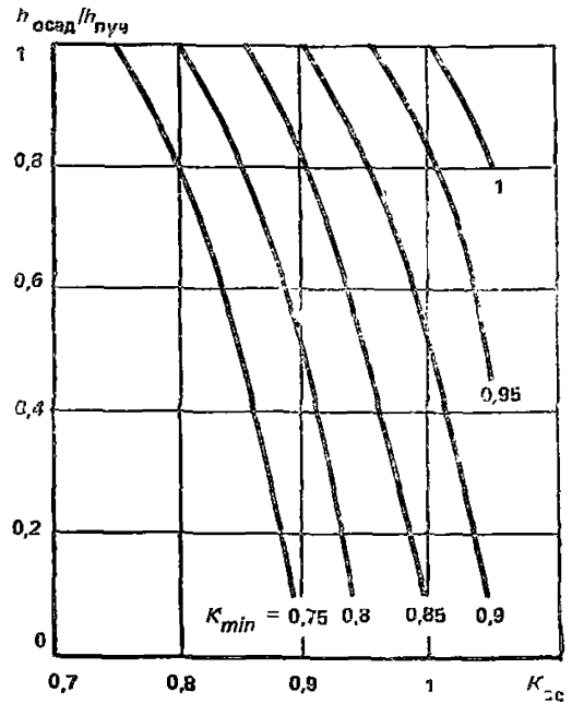
Рис. 12. Графики для определения минимального значения коэффициента уплотнения грунта после осадки
