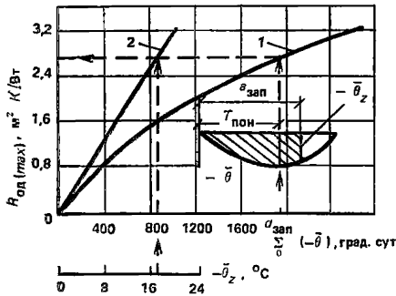
Рис. 1. График для определения параметров R_{\text{од(мак)}} и a_{\text{зап}} .
