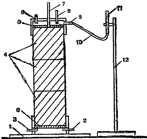
Рис. 1. Схема прибора для определения показателей капиллярных свойств грунта 1 — поддон; 2 — отверстие в поддоне; 3 — дырчатая пластина; 4 — разъемные кольца для заполнения грунтом; 5 — оголовок; 6 — пробка в крышке оголовка; 7 — арретирный винт; 8 — термометр; 9 — отверстие в оголовке; 10 — водоподводящая трубка; 11 — стеклянная градуированная трубка; 12 — держатель
