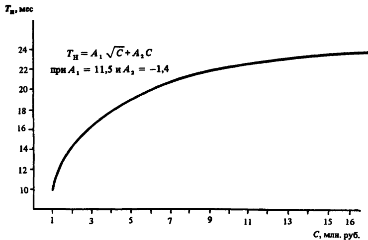
Черт. 22. Определение T н отдельных цехов, корпусов и зданий при C = 1–16 млн. руб.
