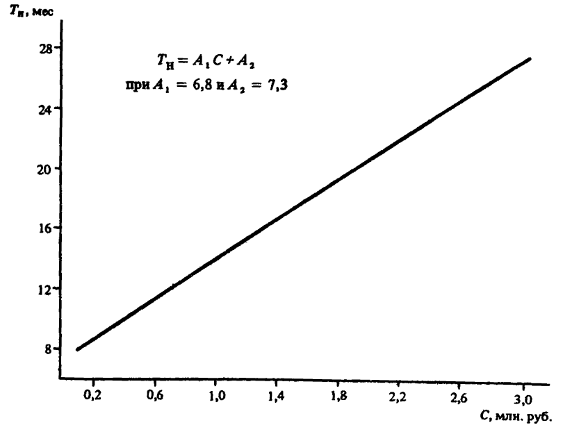
Черт. 48. Определение T_{\text{н}} предприятий по ремонту и обслуживанию сельхозтехники при C = 0,1 - 3,0 млн. руб.
