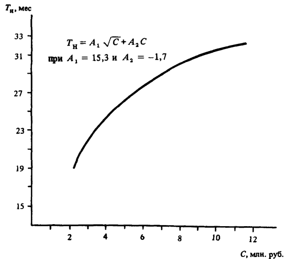
Черт. 4. Определение T_H электростанций при C = 2,2 - 12,0 млн. руб.
