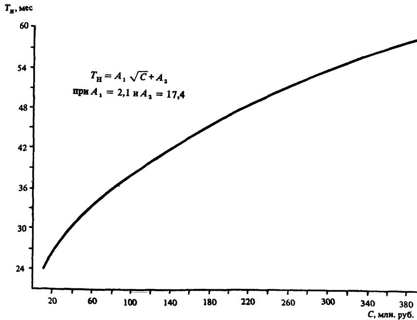
Черт. 24. Определение T_H различных объектов при C = 10-400 млн. руб.
