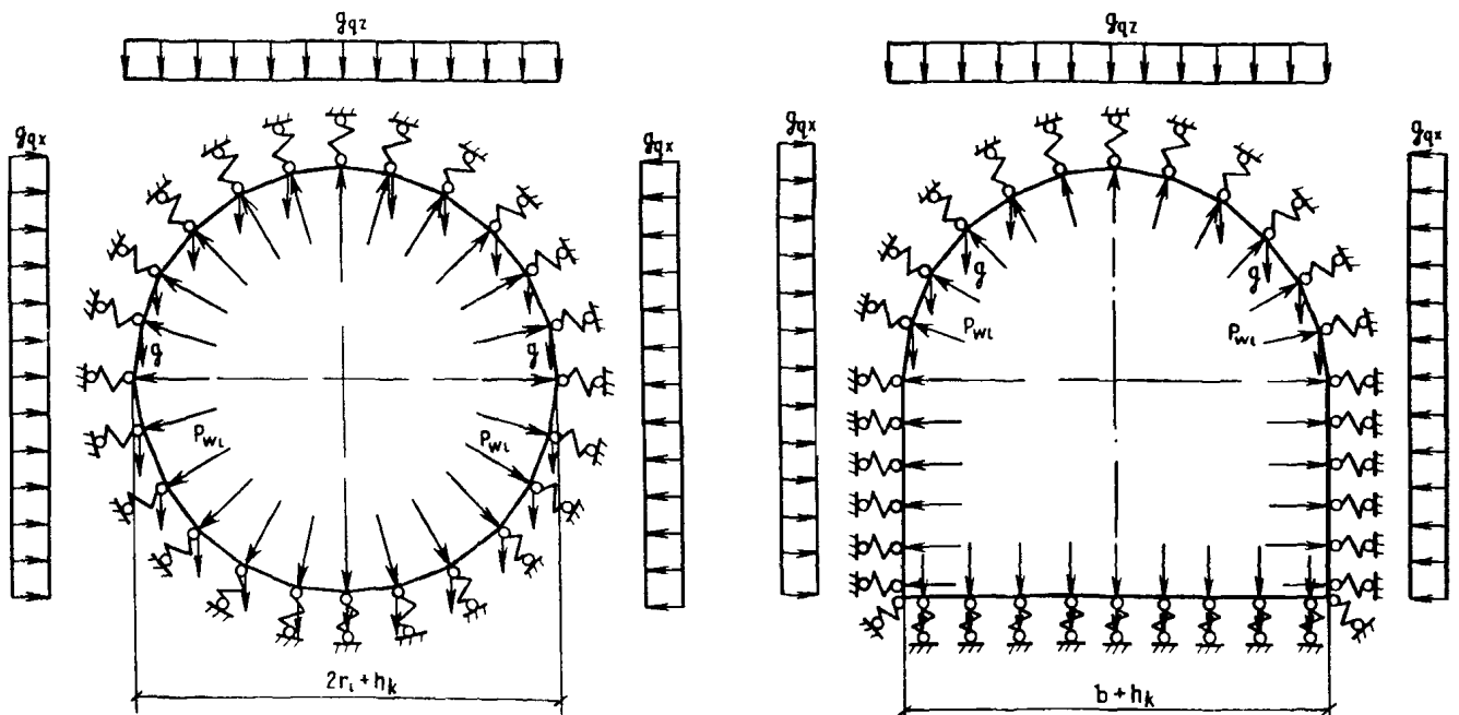
Черт. 1. Расчетные схемы обделок туннелей
