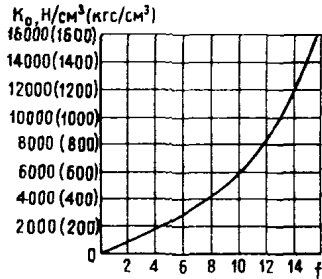
Черт. 2. График зависимости коэффициента удельного отпора K_0 от коэффициента крепости грунта f для трещиноватых грунтов
