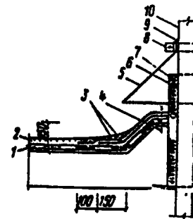
Рис 3. Пример решения пропуска труб
