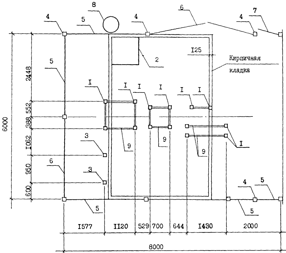
Схема расположения сборных железобетонных элементов фундаментов установки КТПМН 6-10/0,4-0,69 кВ.
