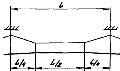
ПРОЛЕТ ПОДВЕСКИ
