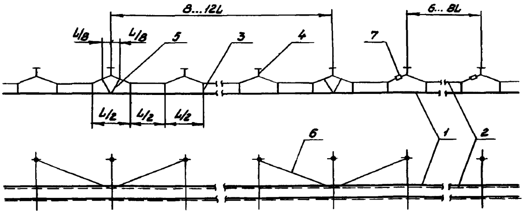
ПРОЛЕТ ПОДВЕСКИ
