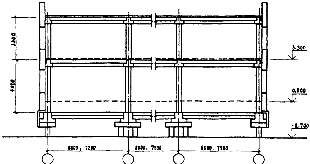
ПОПЕРЕЧНЫЙ РАЗРЕЗ ПО ЗДАНИЮ С ТЕХНИЧЕСКИМ ПОДПОЛЬЕМ НАД ХОЛОДНЫМ ПОДПОЛЬЕМ (ЗДАНИЕ ТИПА 3Т)
