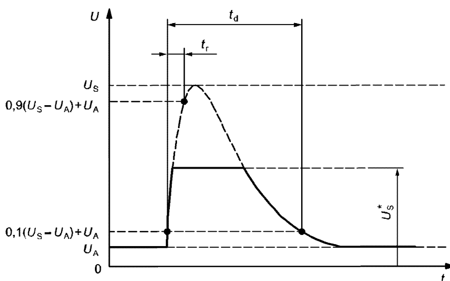
t — время; U — напряжение испытаний; t_d — длительность импульса; t_r — длительность увеличения напряжения импульса; U_A — напряжение питания от работающего генератора; U_S — напряжение питания; U_S^* — напряжение питания при подавлении сброса нагрузки
