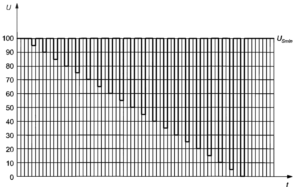
Рисунок 6 — Профиль напряжения питания для испытания на перезагрузку
