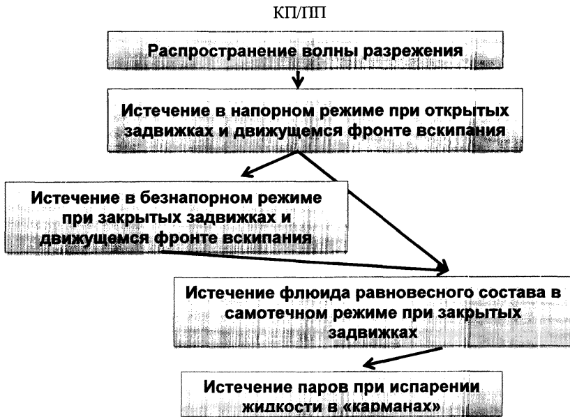
Рисунок 2 – Стадии истечения нестабильной жидкости при гильотинном разрыве КП/ПП
