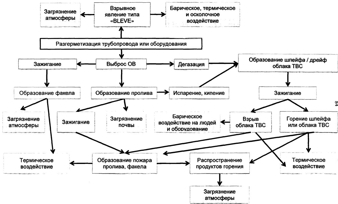
Рисунок 1 – Укрупненная схема развития аварии с выбросом ОВ при авариях на трубопроводах и оборудовании КПП/ПП.
