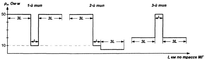
Рисунок 1 - Типы чередования грунтов с различными удельными сопротивлениями
