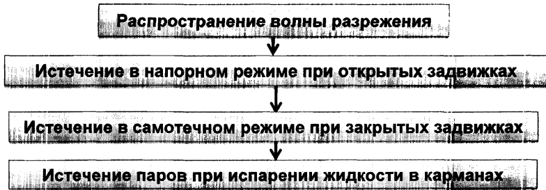
Рисунок 1 – Стадии истечения стабильной жидкости при гильотинном разрыве
