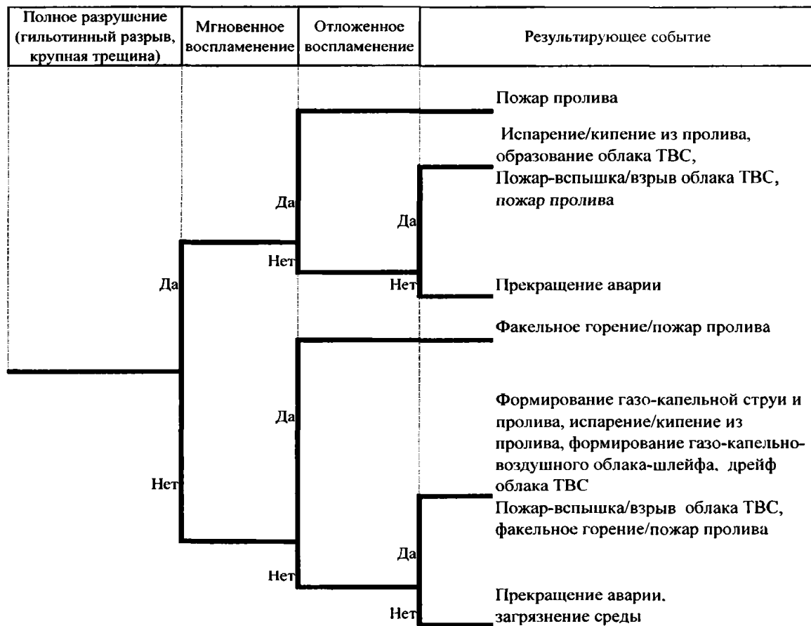
Рисунок 3 – Дерево событий развития аварии с образованием трещины на линейной части трубопровода ШФЛУ
