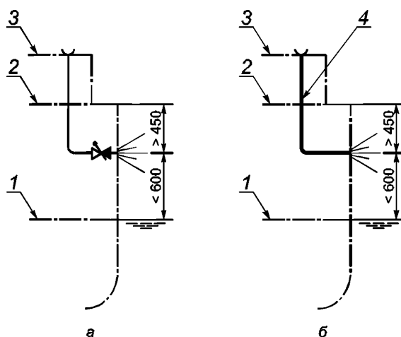
1 — летняя грузовая ватерлиния; 2 — палуба надводного борта; 3 — палуба надстройки; 4 — толстостенный трубопровод
