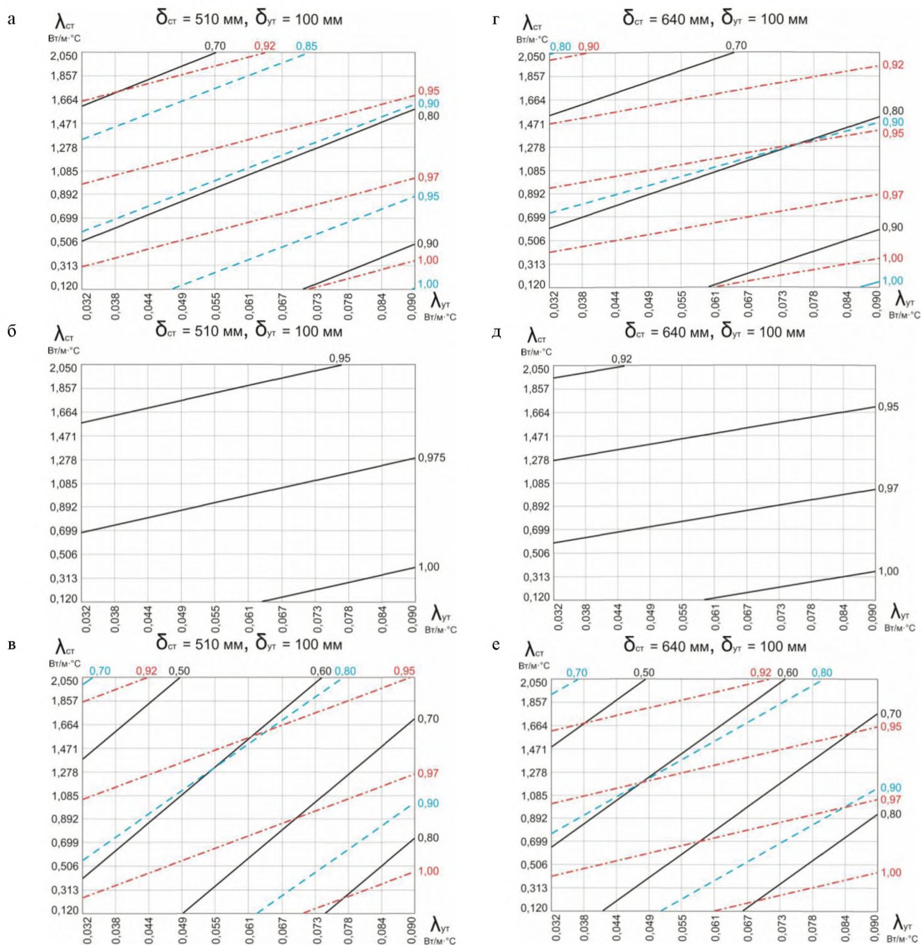
Рис. 7.1-5. Зависимость коэффициента влияния дефектов теплозащиты k от коэффициента теплопроводности утеплителя \lambda_{ут} и коэффициента теплопроводности основания \lambda_{ст} при заданных значениях толщин основания и утеплителя: а, г – зазор в стыке плит утеплителя; б, д – зазор в стыке кронштейна и плит утеплителя; в, е – отслоение плит утеплителя от основания;
