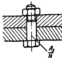
Черт. 10. Посадка чистого ббата в отверстие из-под развертки
