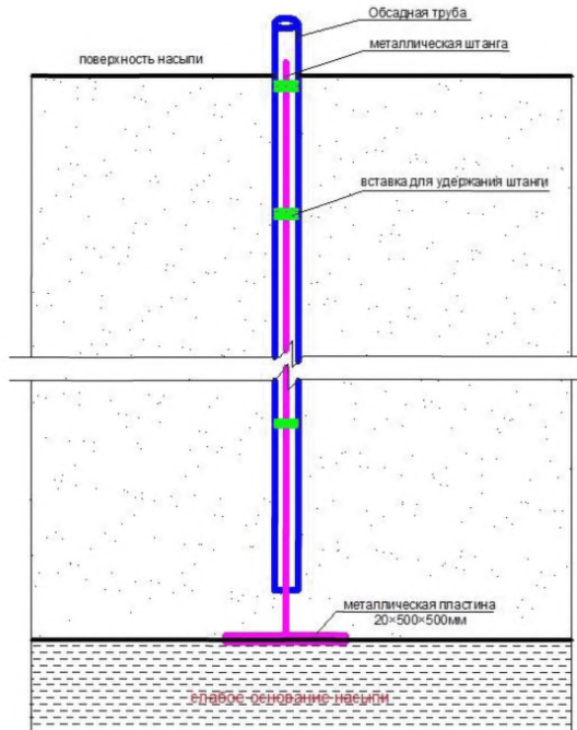
Рисунок 1 - Осадочная марка
