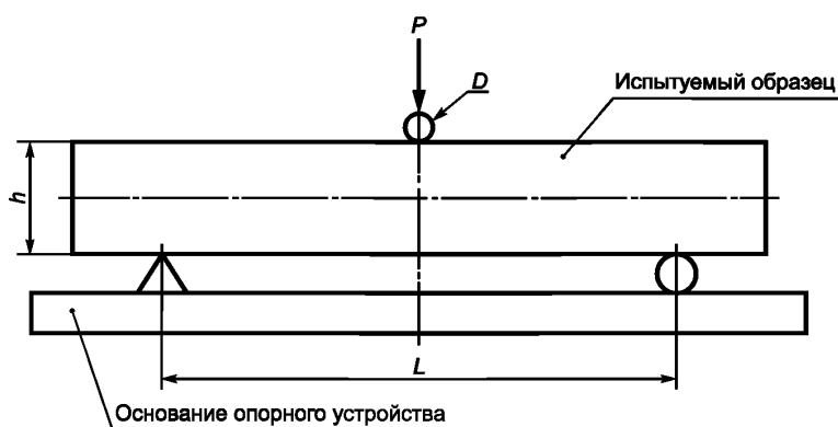
Рисунок 1 — Схема опорного устройства
