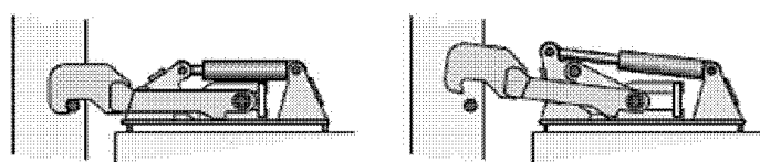
Рис. 15 Стопорный гак 1
