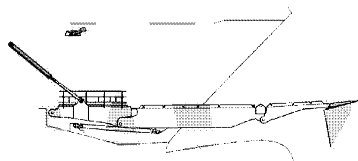
Рис. 4 Носовая грузовая аппарель – аппарель частично выдвинута
