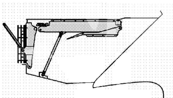
Рис. 2 Носовая грузовая аппарель – положение «по-походному», кормовая часть (внутренняя дверь) отсоединена
