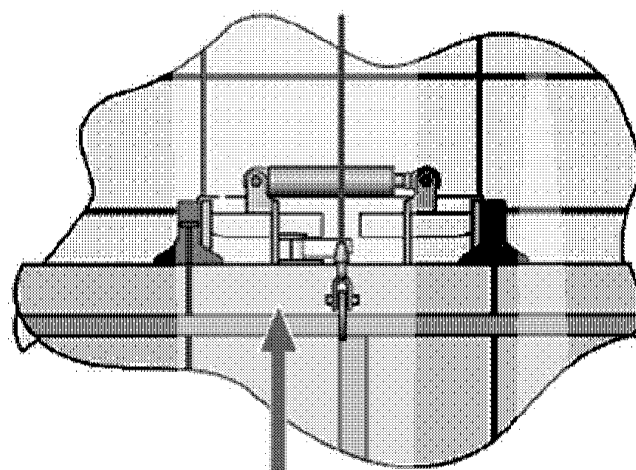
Рис. 30 Грузовая дверь – верхнее боковое гидравлическое задраивающее устройство не задраено
