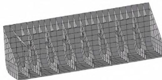
Рис. 2.2.3-2 Скуловые танки
