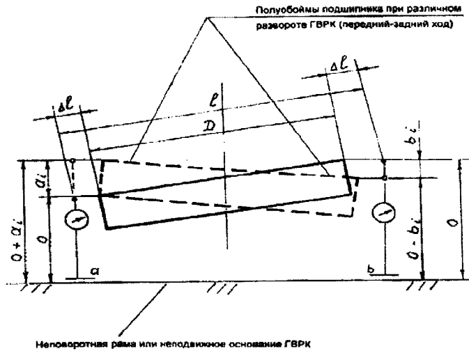
Рис. 2 Схема измерений линейных перемещений полуобоймы подшипника поворота ГВРК
