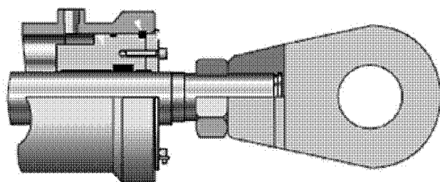
Рис. 19 Гидравлический привод 2
