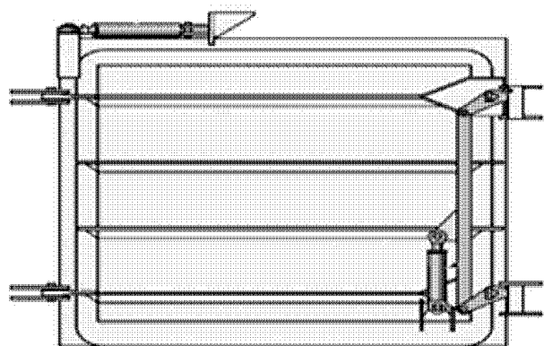
Рис. 26 Бункерный люцпорт – тип 2, в закрытом положении, вид изнутри
