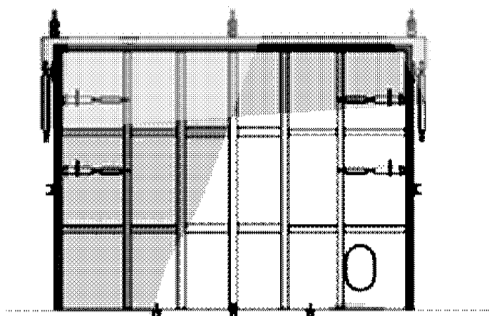
Рис. 2 Носовая грузовая аппарель – положение «по-походному», кормовая часть (внутренняя дверь) отсоединена
