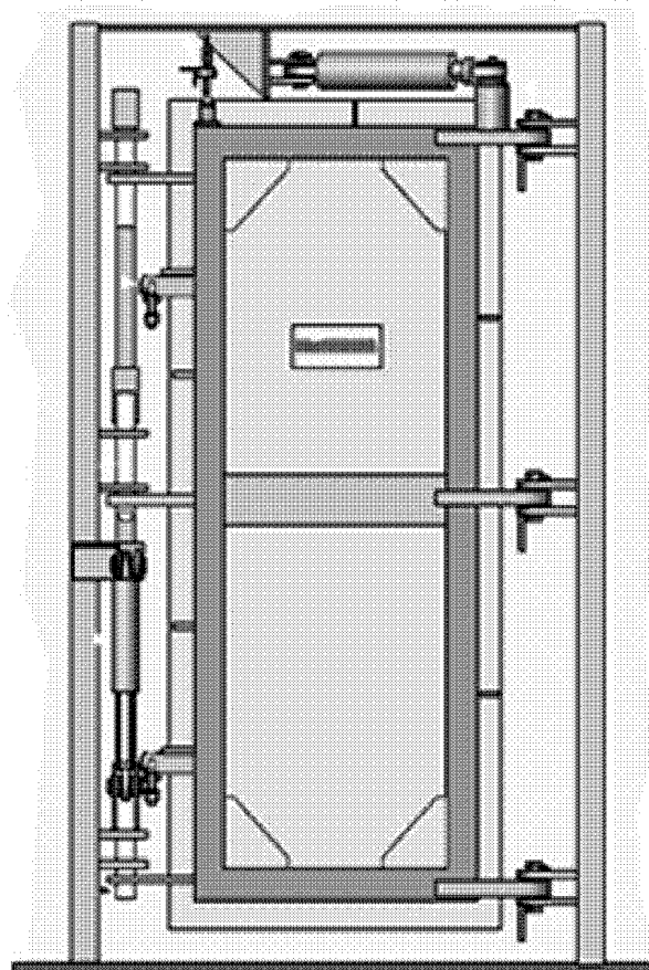
Рис. 23 Внутренняя дверь в закрытом положении
