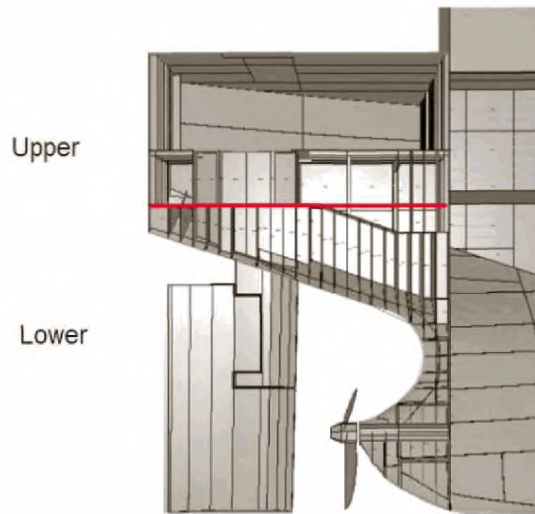
Рис. 2.2-3 «Типового района», указанного для танка ахтерпика 3
