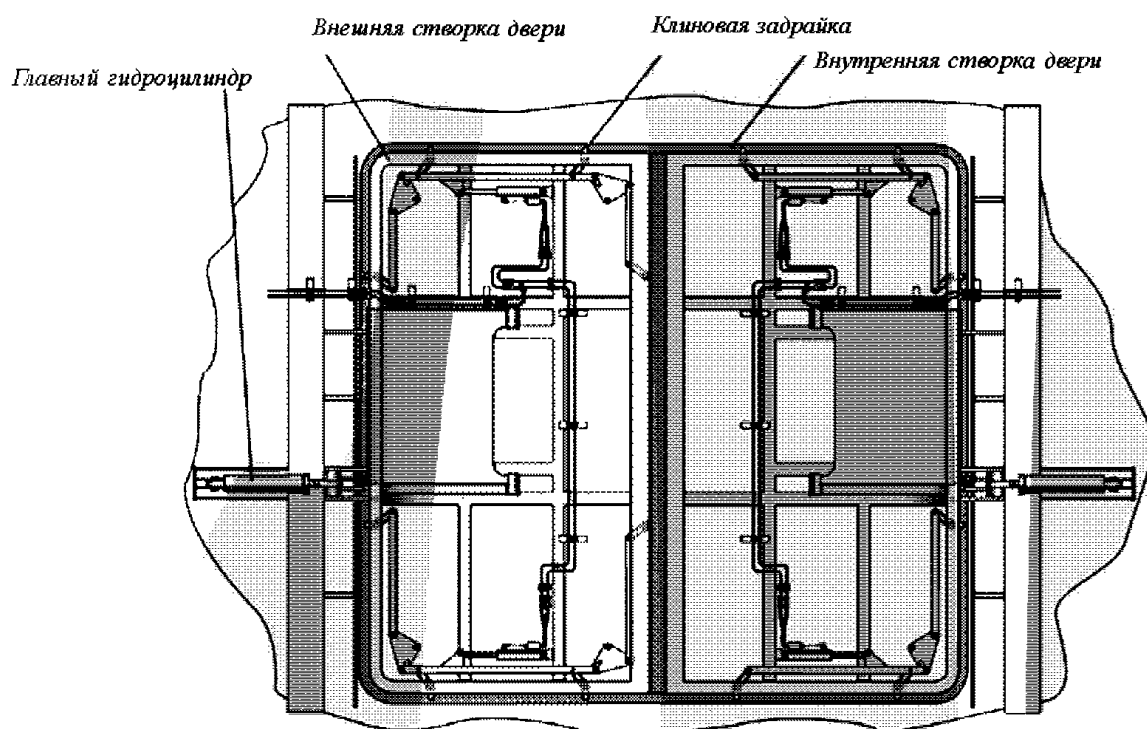
Рис. 32 Бортовая дверь – двухстворчатая, закрытое положение, вид изнутри
