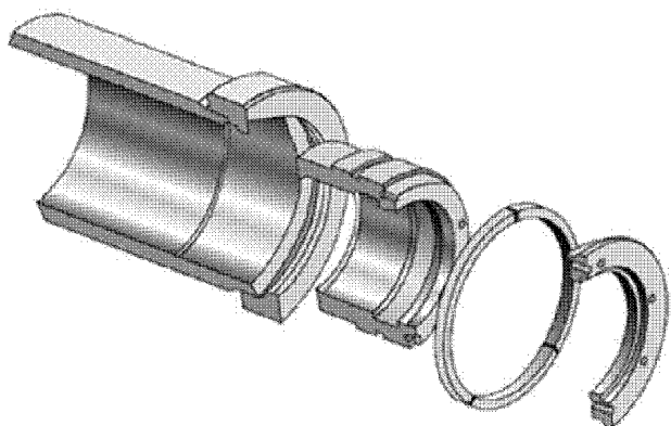
Рис. 18 Гидравлический привод 1
