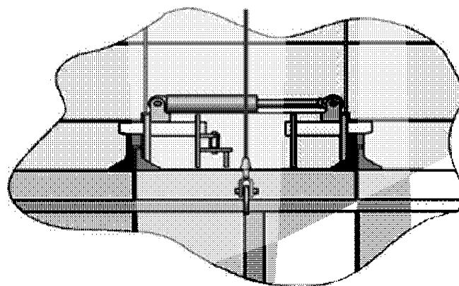
Рис. 31 Грузовая дверь – верхнее боковое гидравлическое задраивающее устройство задраено
