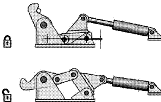
Рис. 16 Стопорный гак 2
