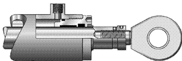
Рис. 21 Гидравлический привод 4
