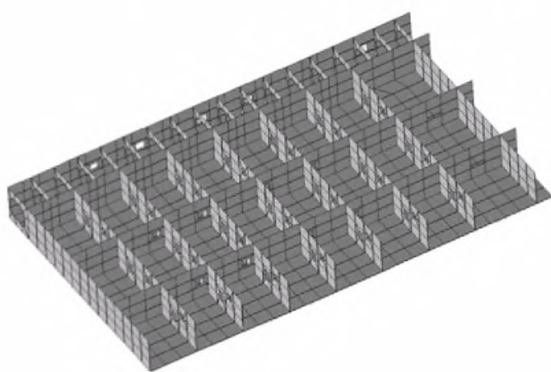
Рис. 2.2.3-3 Междудонные танки
