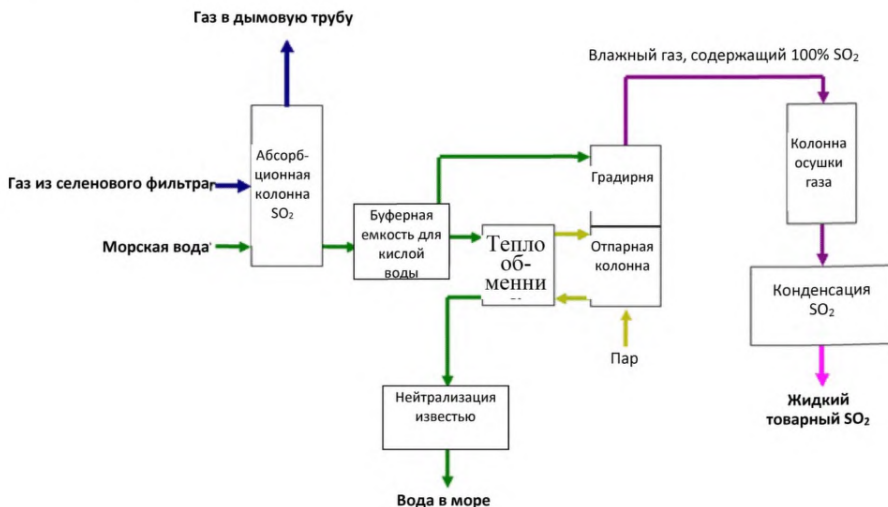
Рисунок А.31 – Схема процесса производства жидкого диоксида серы
