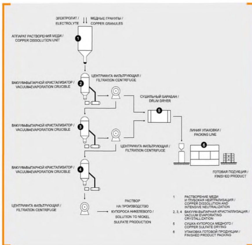
Рисунок А.21 – Технологический процесс производства медного купороса
