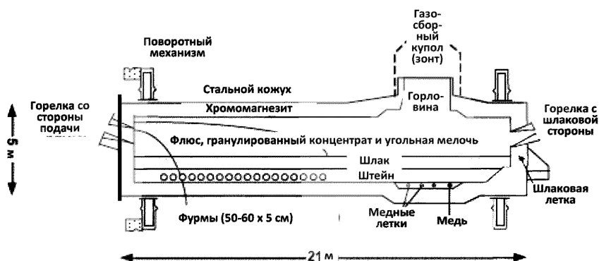
Рисунок А.8 – Реактор Noranda
