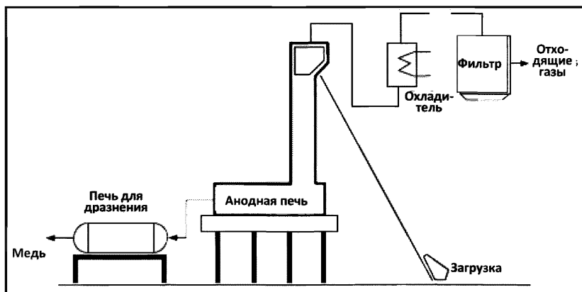
Рисунок А.128 – Технология Contimelt [26]
