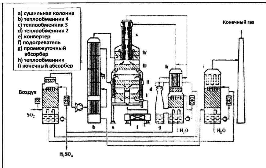
Рисунок А.30 – Типичная сернокислотная установка двойной абсорбции
