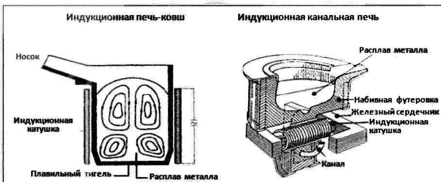
Рисунок А.117 – Индукционные печи
