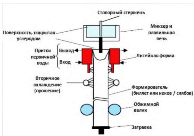
Рисунок 2.7 – Принципиальная схема непрерывного и циклического литья [26]
