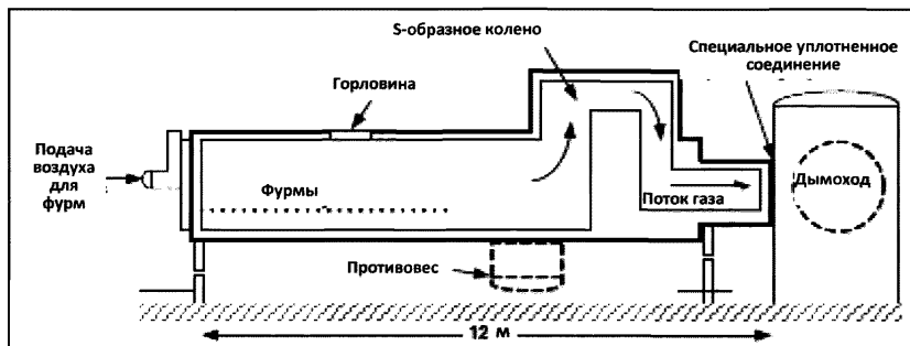
Рисунок А.106 – Конвертер Хобокен
