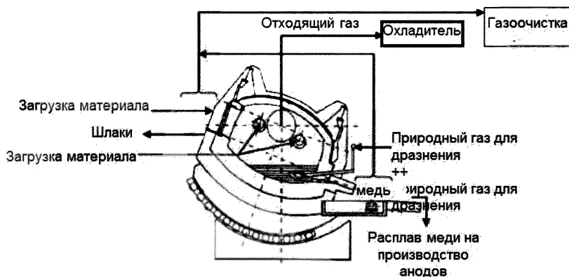
Рисунок А.2 – Устройство наклоняемой отражательной подовой печи для плавки вторичной меди
