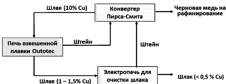
Рисунок 2.12 – Переработка медного шлака в электродуговой печи
