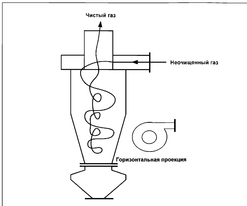
Рисунок А. 24 – Схема устройства циклона
