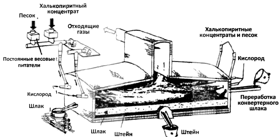
Рисунок А.73 – Печь INCO
