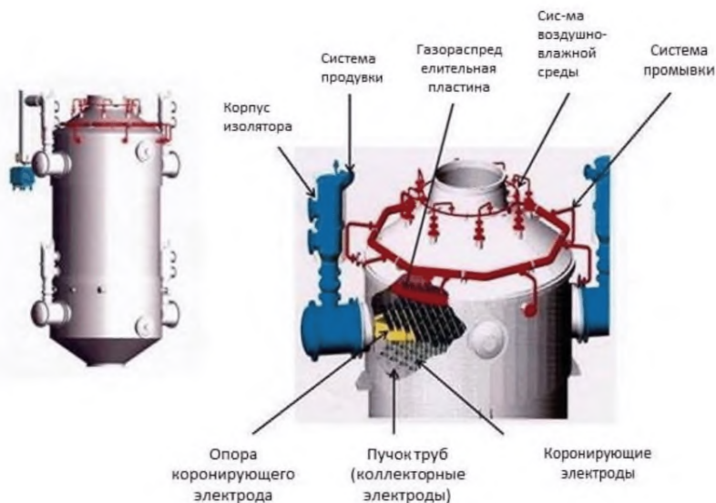
Рисунок А.2314 – Схема устройства мокрого электрофильтра
