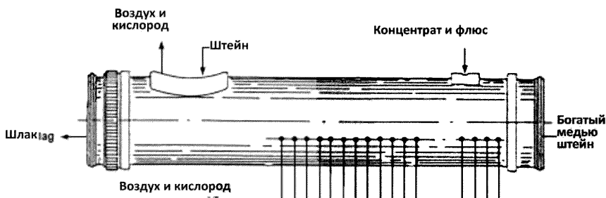
Рисунок А.9 – Реактор El Teniente
