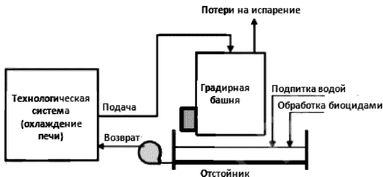
Рисунок А.32 – Пример рециркуляции охлаждающей воды
