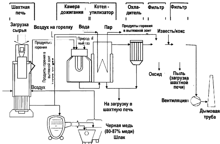
Рисунок А.4 – Шахтная печь для выплавки вторичной меди [33]
