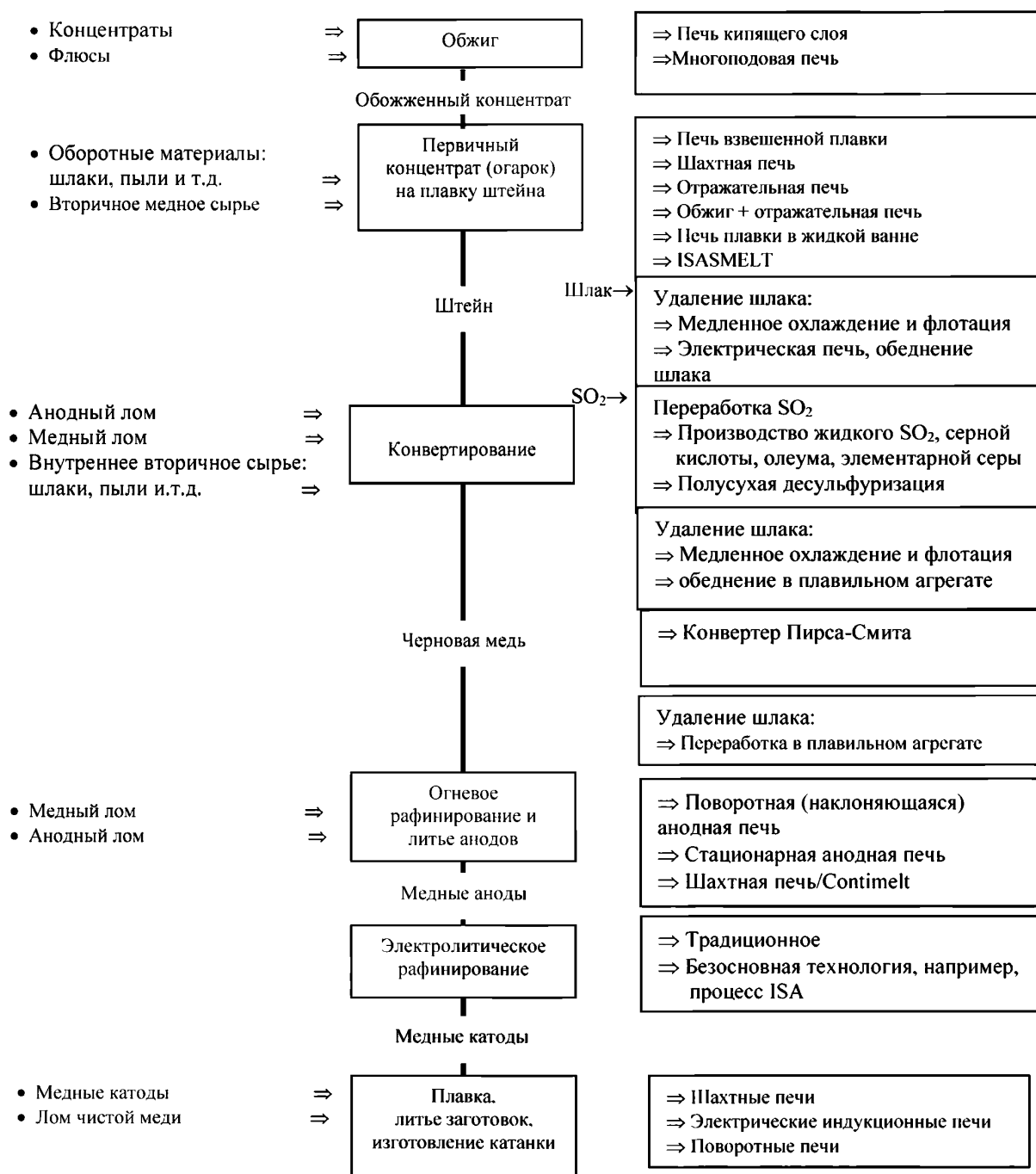
Рисунок 2.1 – Схема процесса производства меди
