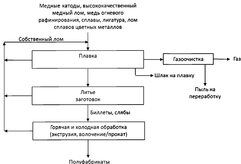
Рисунок 2.6 – Общая схема процесса производства полуфабрикатов [26]
