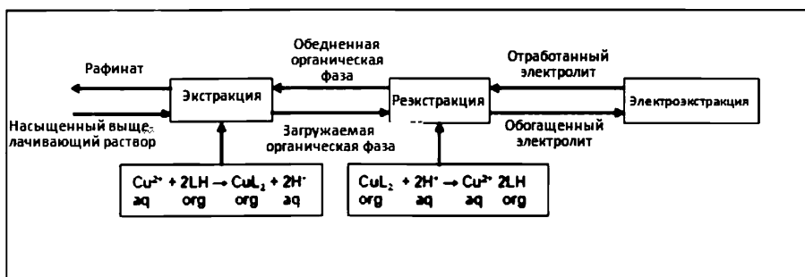
Рисунок А.139 – Этапы экстракции растворителем
