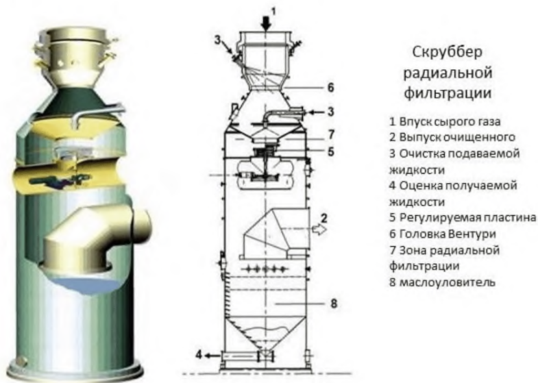
Рисунок А.28 – Радиальный мокрый скруббер
