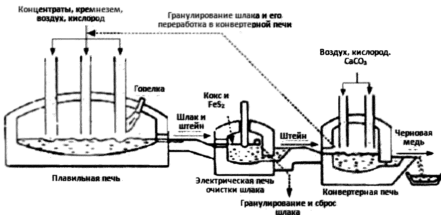
Рисунок А.10 – Технология Mitsubishi
