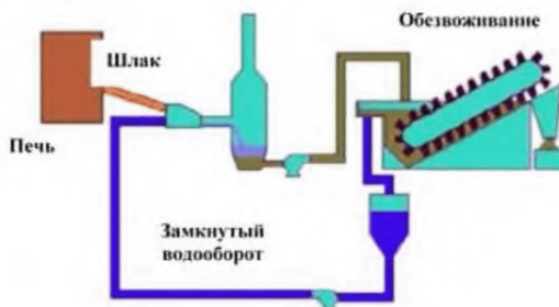
Рисунок 2.11 – Замкнутый цикл водооборота
