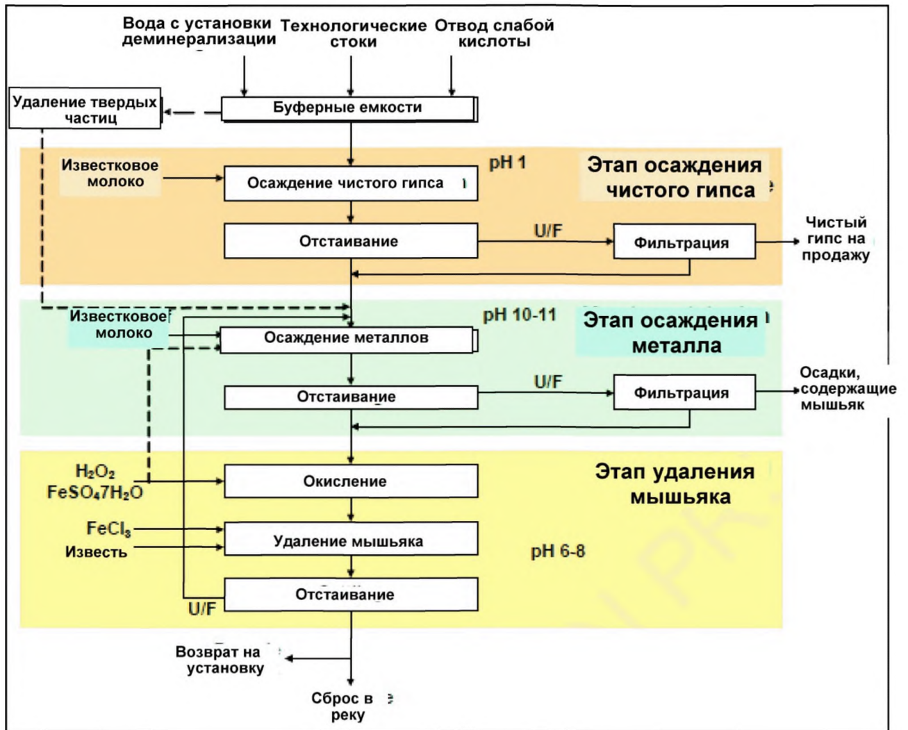
Рисунок А.33 – Схема процесса очистки слабокислых стоков
