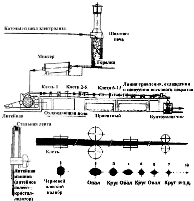
Рисунок 2.4 – Примерная схема процесса Southwire [26]
