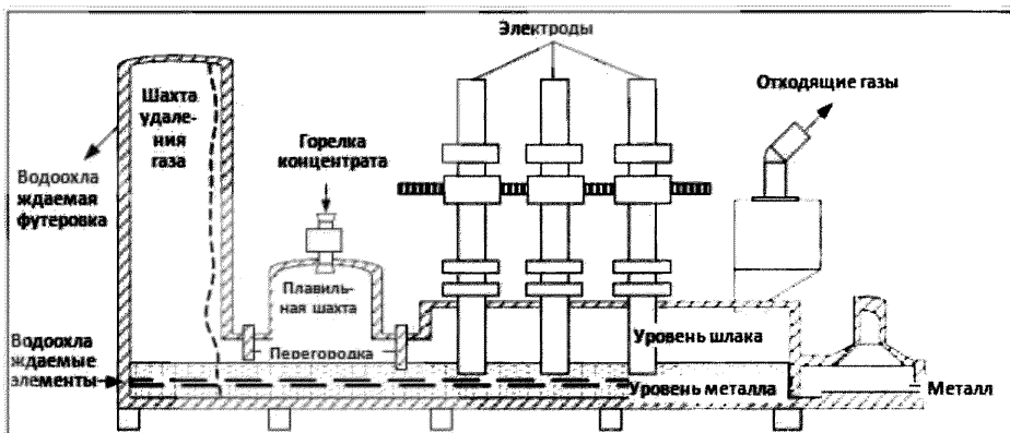
Рисунок А.84 – Печь Кивцет
