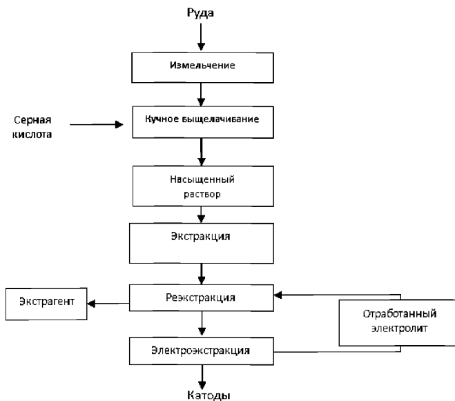
Рисунок 2.2 – Обобщенная технологическая схема гидromеталлургического процесса [29]
