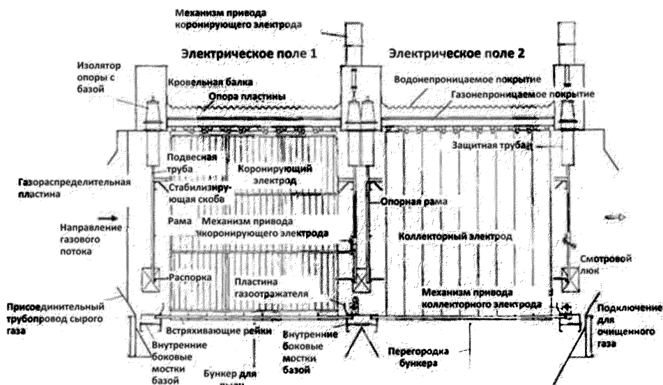
Рисунок А.22 – Схема устройства электрофильтра (показаны только две зоны)
