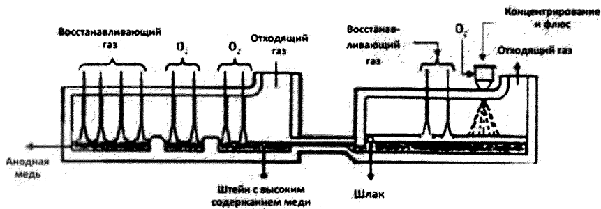
Рисунок А.51 – Схема процесса Contop
