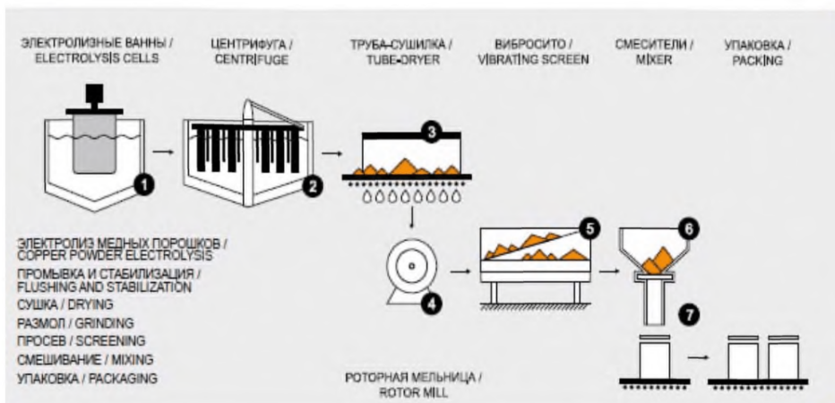
Рисунок А.20 – Технологический процесс производства порошков
