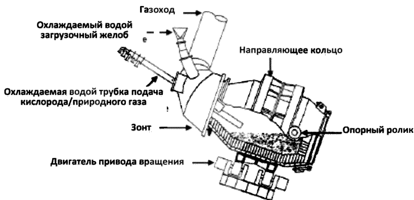
Рисунок А.7 – Поворотный конвертер с верхним дутьем и наклонная вращающаяся кислородно-топливная печь
