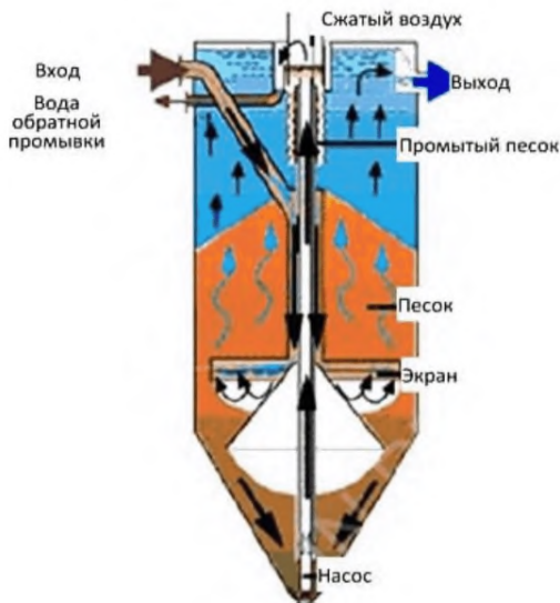
Рисунок А.34 – Схема песчаного фильтра
