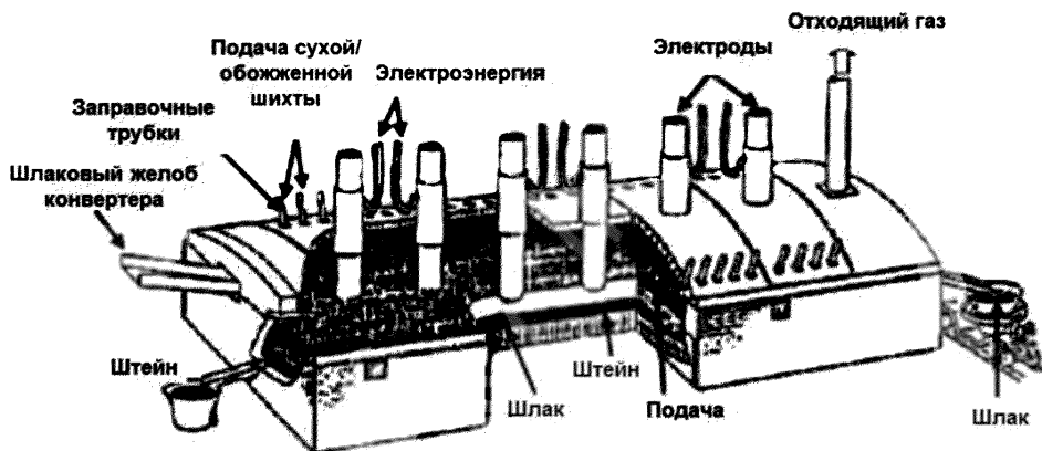
Рисунок А.5 – Электрическая печь для плавки концентрата и обожженного материала
