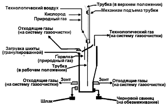
Рисунок А.6 – Технология Ausmelt (Sirosmelt)/ISASMELT [26]
