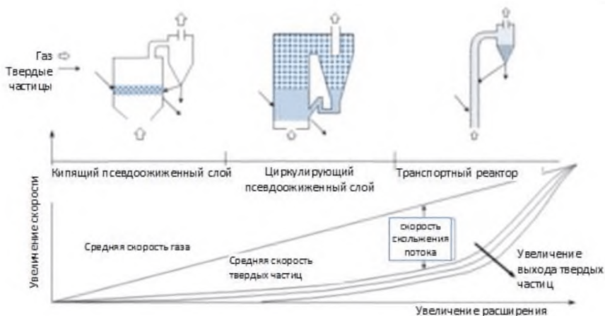
Рисунок А.1 – Реакторы для плавки в псевдоожженном слое
