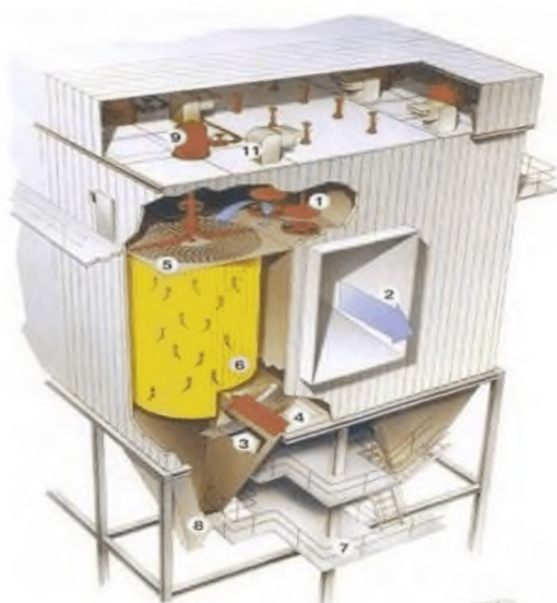
Рисунок А.27 – Система очистки воздухом низкого давления
