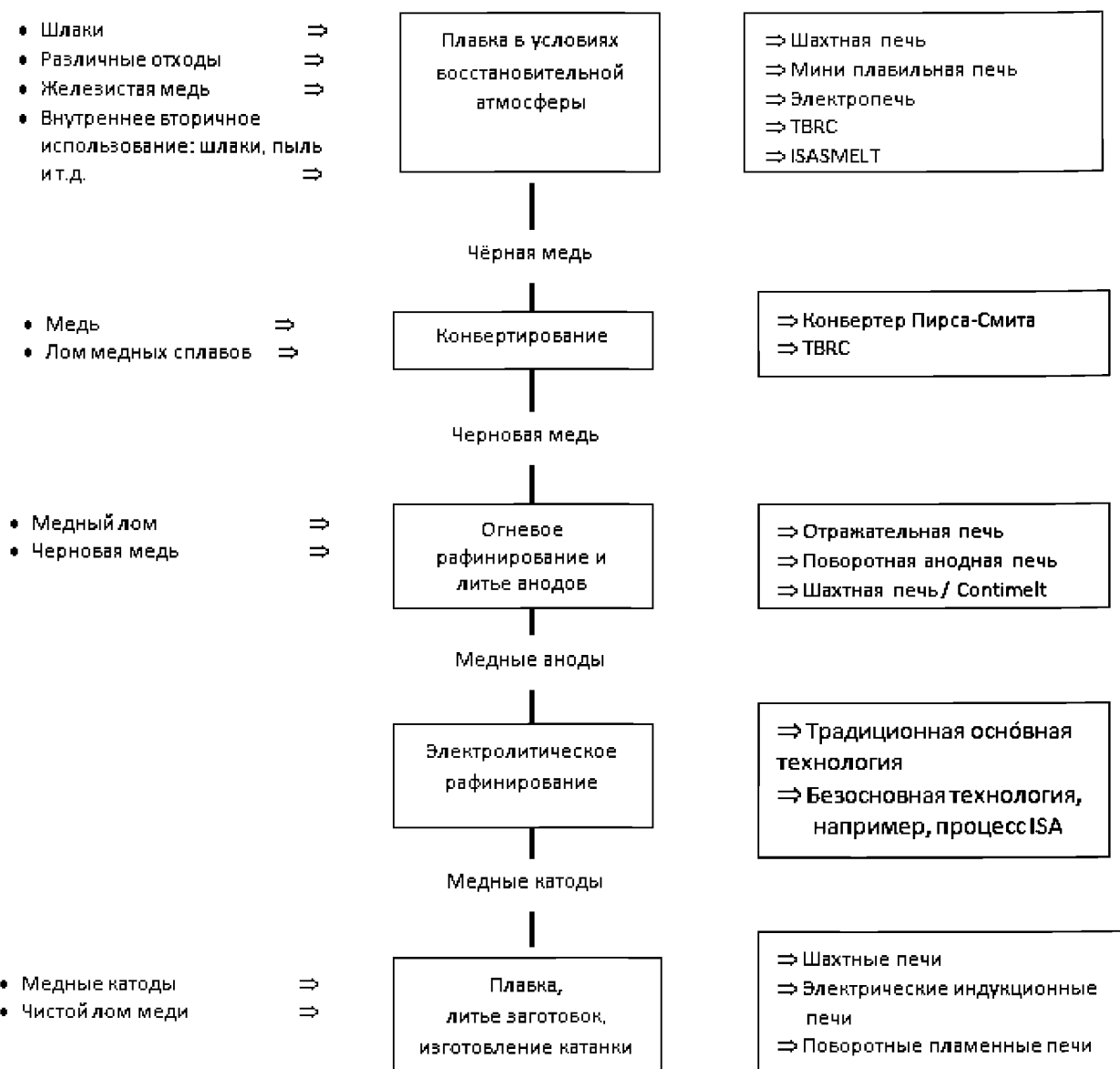
Рисунок 2.3 – Общая технологическая схема производства меди [19]
