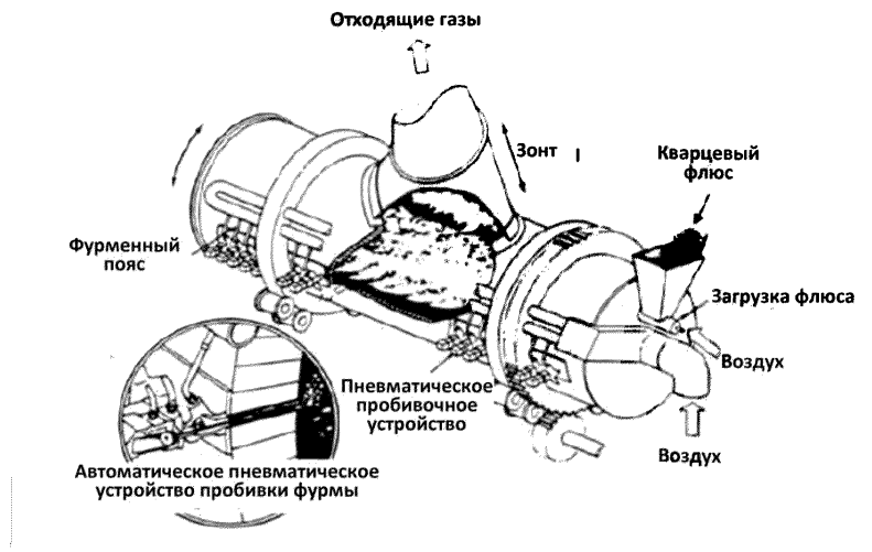
Рисунок А.95 – Конвертер Пирса – Смита
