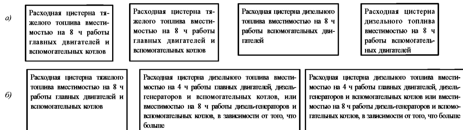
Рис. 13.8.1-2 Расходные цистерны, используемые для подвода топлива к главным двигателям и вспомогательным котлам, работающим на тяжелом топливе, и вспомогательным двигателям, работающим на дизельном топливе:
