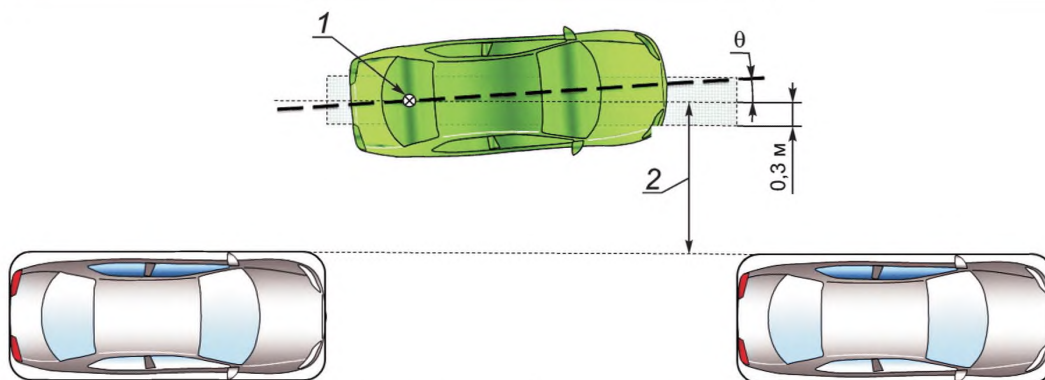
1 — контрольная точка; 2 — d_{lcd} + 1/2 ширины транспортного средства
