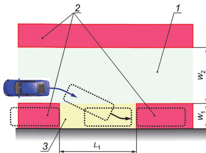
1 — область, где разрешено управление APS; 2 — области ограниченного движения; 3 — целевое парковочное место; L_1 = 1,4L_v м, L_v — длина транспортного средства; W_1 = 2,5 м; W_2 = 4,5 м или более
