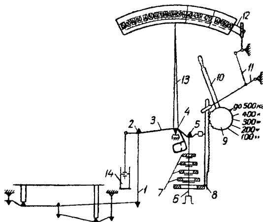
Рис. 12. Схема платформенных циферблатных весов (з-да «Мосмет»).
