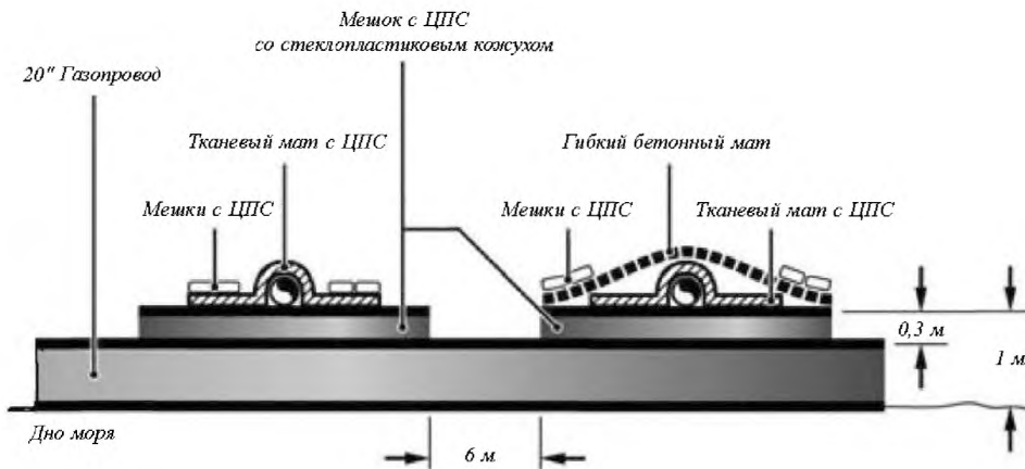
Рис. 11.2-2 Примеры конструктивных решений по пересечениям подводных трубопроводов [2]
