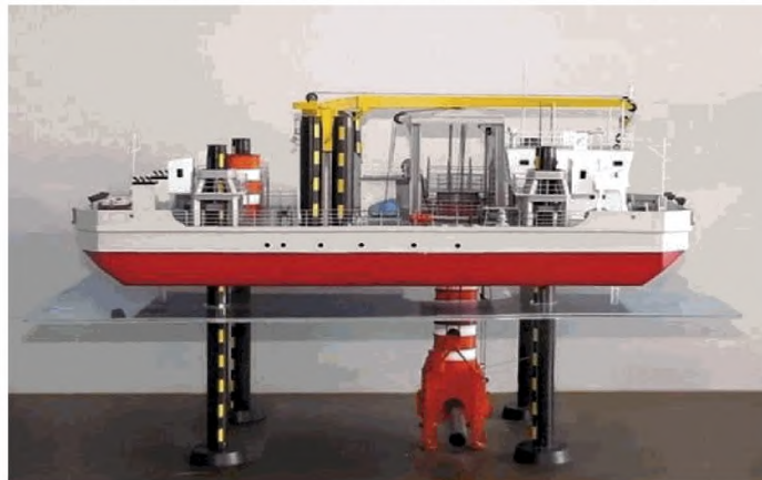
Рис. 12.3-3 Специализированное плавучее ремонтное средство СПРС-К (проект 91030)
