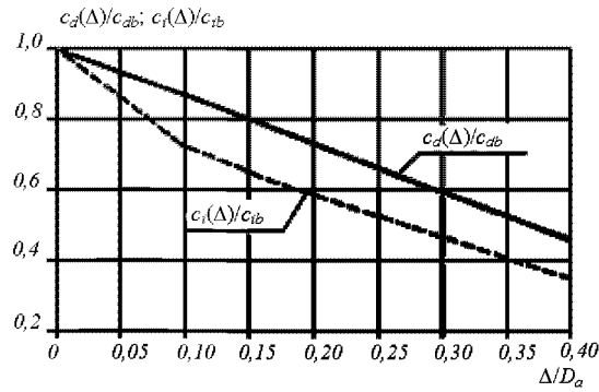
Рис. 3 Коэффициенты c_a и c_i в зависимости от относительного заглубления трубопровода \Delta/D_o
