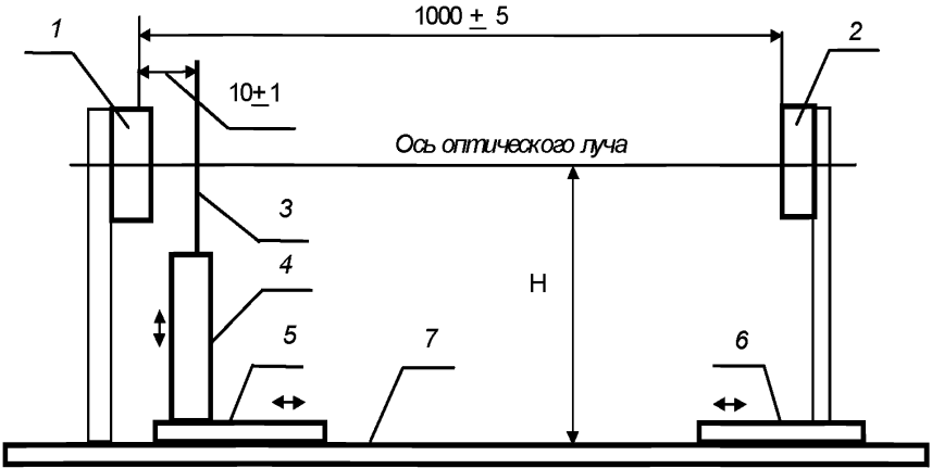
Рисунок А. 2. Схема расположения элементов линейного извещателя и аттенюатора (вариант 2 - приемопередатчик и отражатель):
