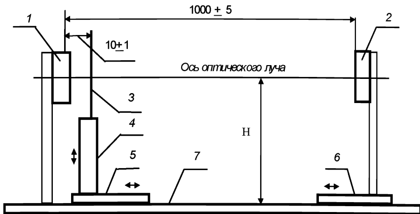
Рисунок А. 1 Схема расположения элементов линейного извещателя и аттенюатора (вариант 1 - передатчик и приемник):
