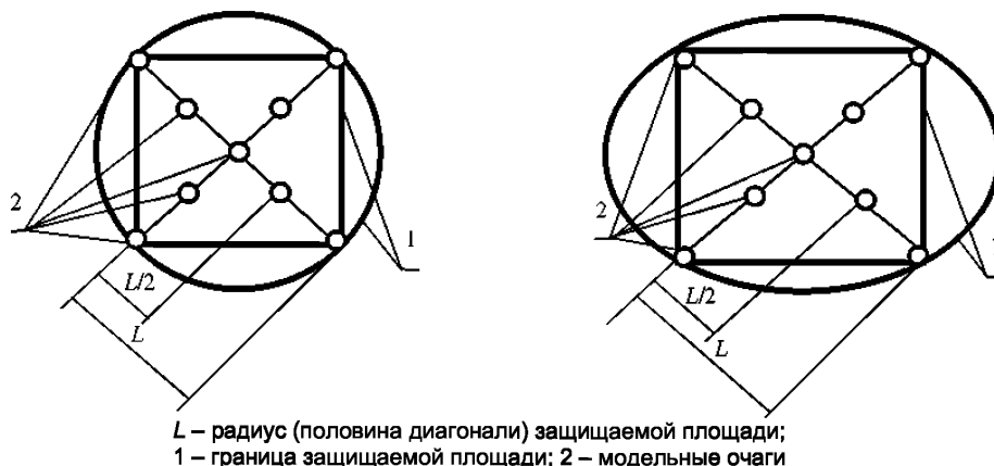
Рисунок 1 – Схема расположения модельных очагов пожара
