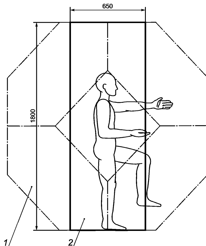
1 — пространственная игровая сеть; 2 — цилиндрический шаблон
