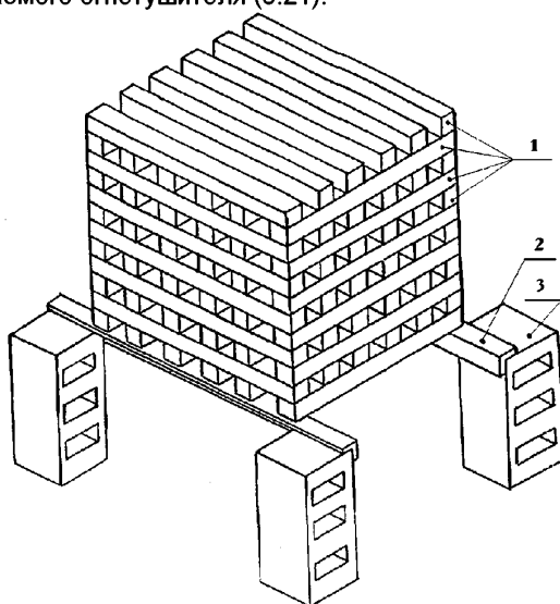
Рисунок В.1 – Устройство деревянного штабеля (модельного очага) для проведения испытаний по тушению модельного очага пожара класса А
