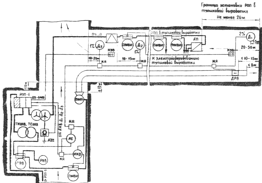
Рис.2. Схема электроснабжения и расстановки электрооборудования при установке передвижной подстанции в тупиковой выработке
