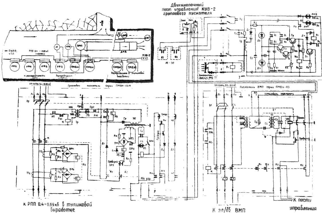
Рис.5. Принципиально-монтажная схема электроснабжения тупиковой выработки с дистанционным управлением групповым пускателем непосредственно от забоя по обособленному кабелю
