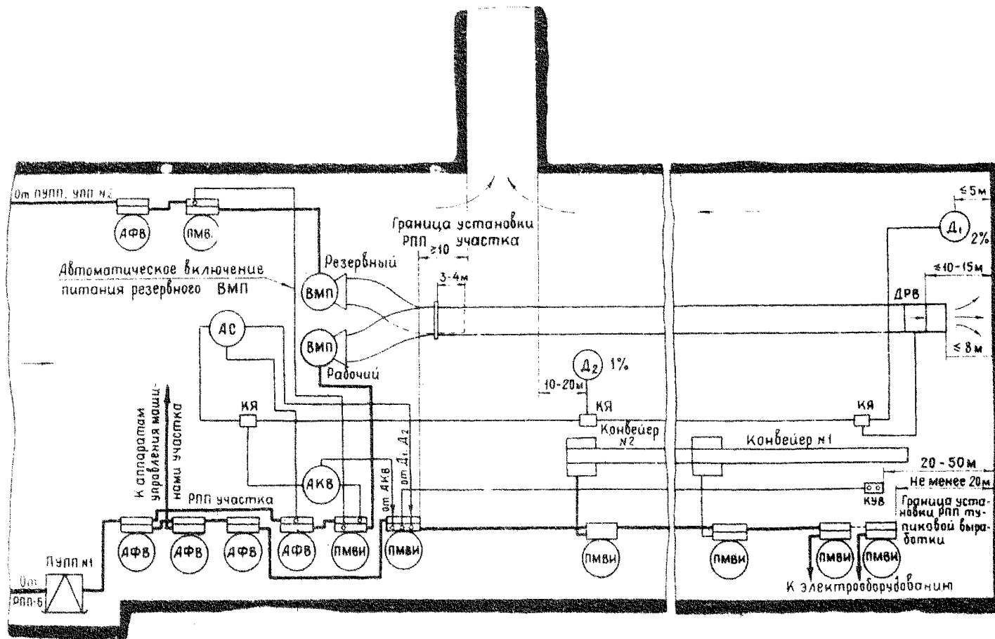
Рис.3. Схема электроснабжения и расстановки электрооборудования в тупиковой выработке с резервным ВМП
