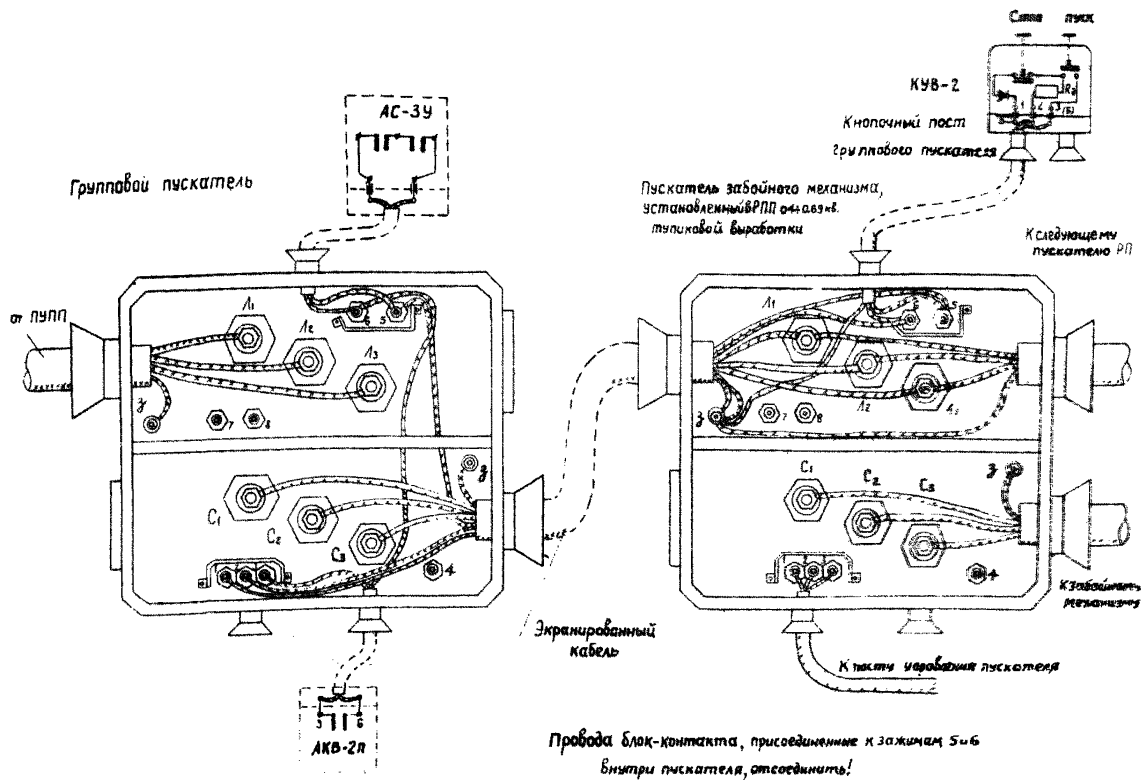
Рис. 6. Монтажная схема соединения цепей дистанционного управления групповым пускателем тупиковой выработки непосредственно от забоя для случая совмещения жил цепи управления в одном кабеле с силовыми жилами
