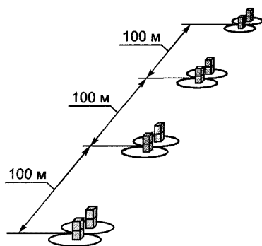
Рисунок 1 — Размещение испытательного оборудования
