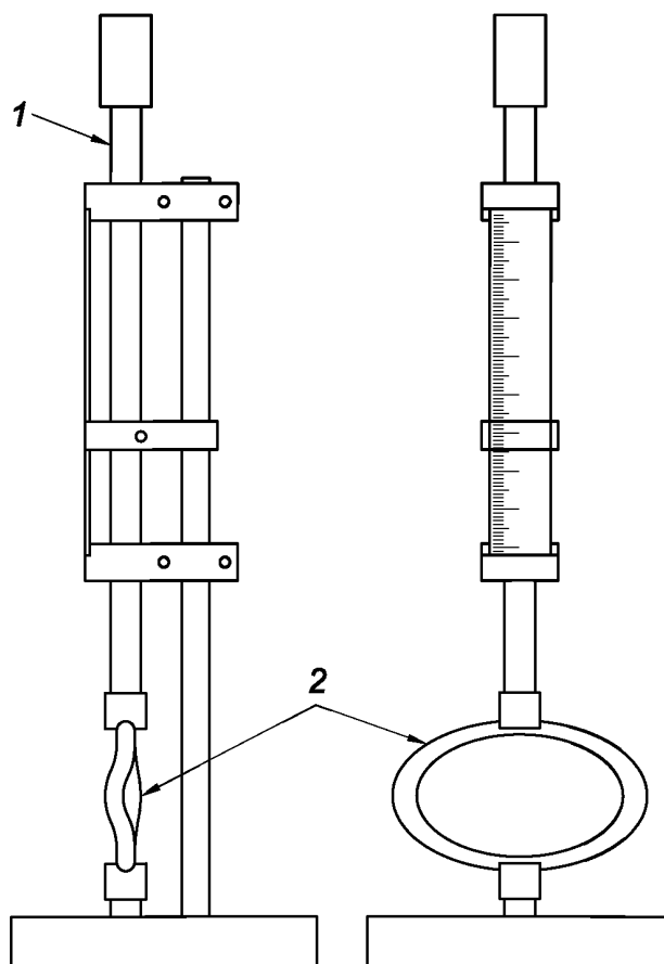
1 — стержень массой 280 г; 2 — диафрагма
