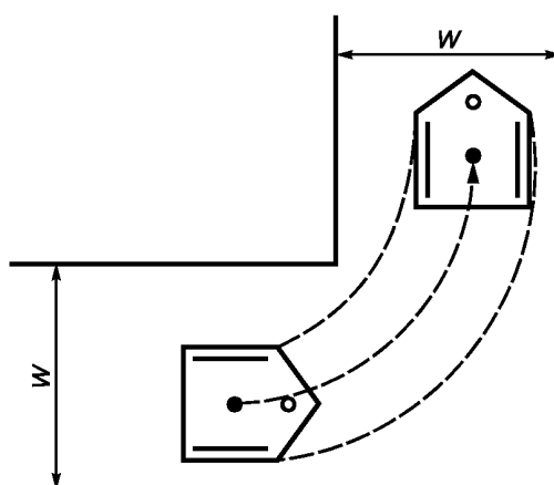
Рисунок А.3 — Ширина L-образного поворота мобильного робота
