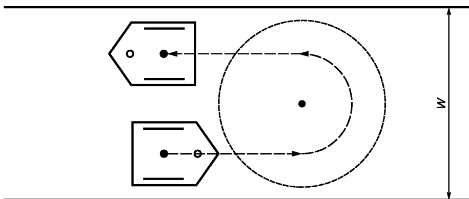
Рисунок А.1 — Ширина U-образного разворота мобильного робота
