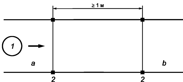
1 — мобильный робот; 2 — датчик; a — участок ускорения, b — участок торможения
