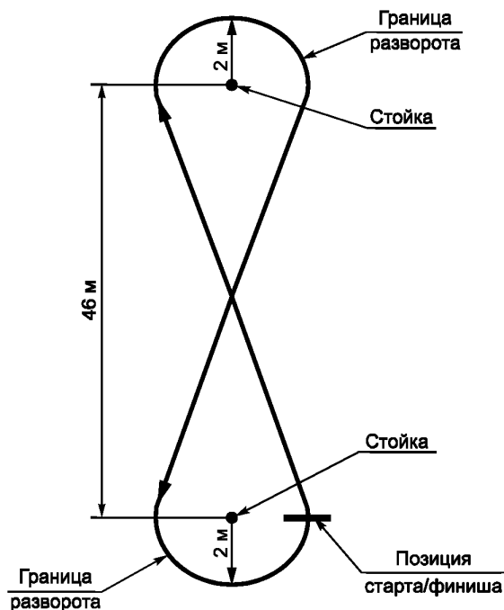
Рисунок 1 — Схема движения робота с буксируемым объектом
