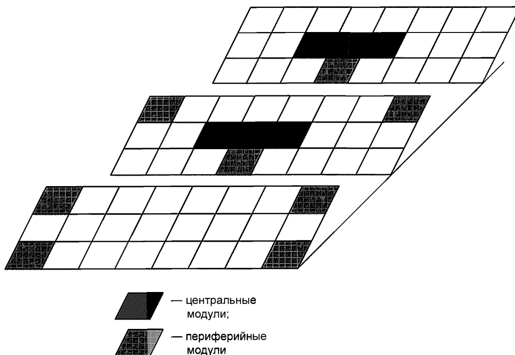
Рисунок 1 — Пример выбора типичных ФМ и ФМ с предельным значением рабочей температуры
