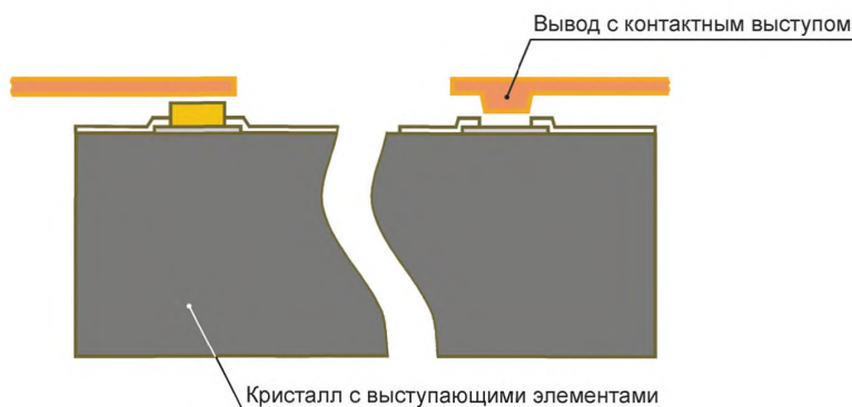
Рисунок 2 — Кристалл с контактными элементами
