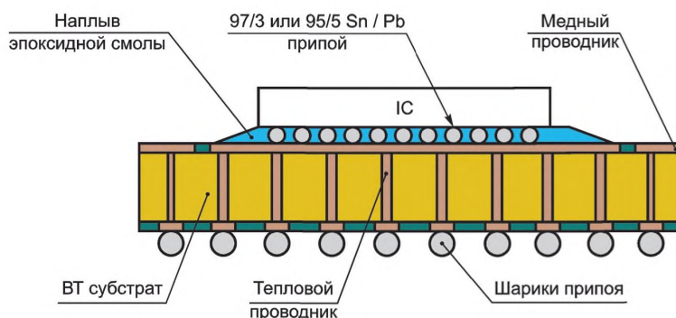
Рисунок 4 — Компонент типа «flip chip»
