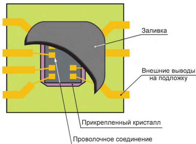
Рисунок 3 — Чип на плате
