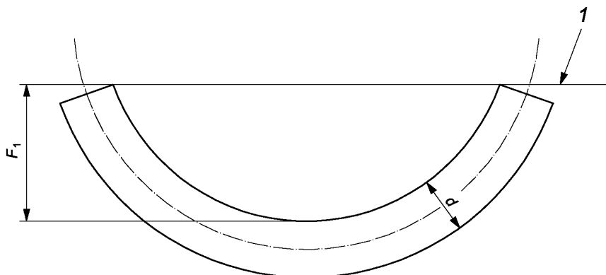
Рисунок 2 — Определение прогиба F_1
