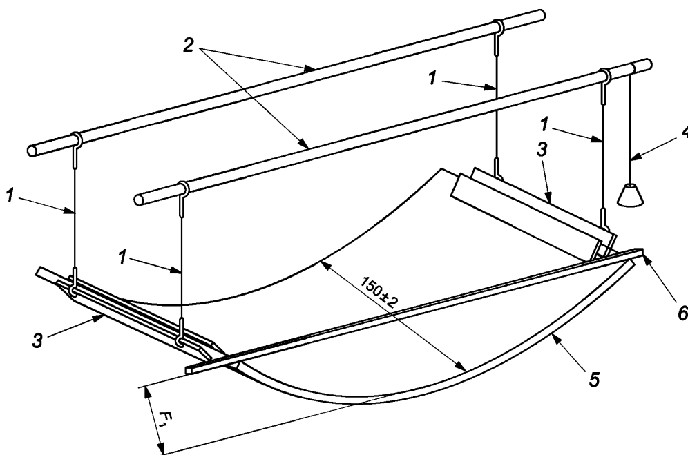
1 — четыре стальных несущих тросика; 2 — две жесткие горизонтальные балки; 3 — два зажима; 4 — шнуровой отвес; 5 — испытуемый образец; 6 — жесткий стержень для установления линии отсчета
