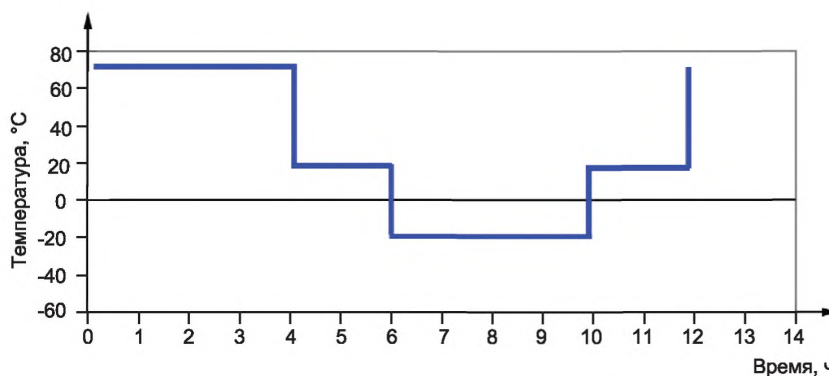
Рисунок 1 — Профиль изменения температуры по 7.2.4 — температурное циклирование
