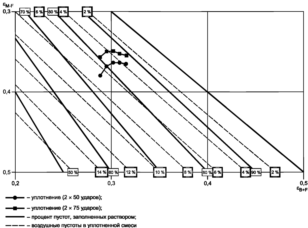
Рисунок С.8 — Кривые в координатах ( \epsilon_{B+F} , \epsilon_{M-F} )
