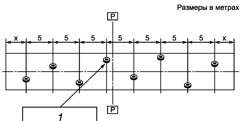
Рисунок 5 — Пример выбора точек отбора зерна на участке испытательного трека длиной 40 м
