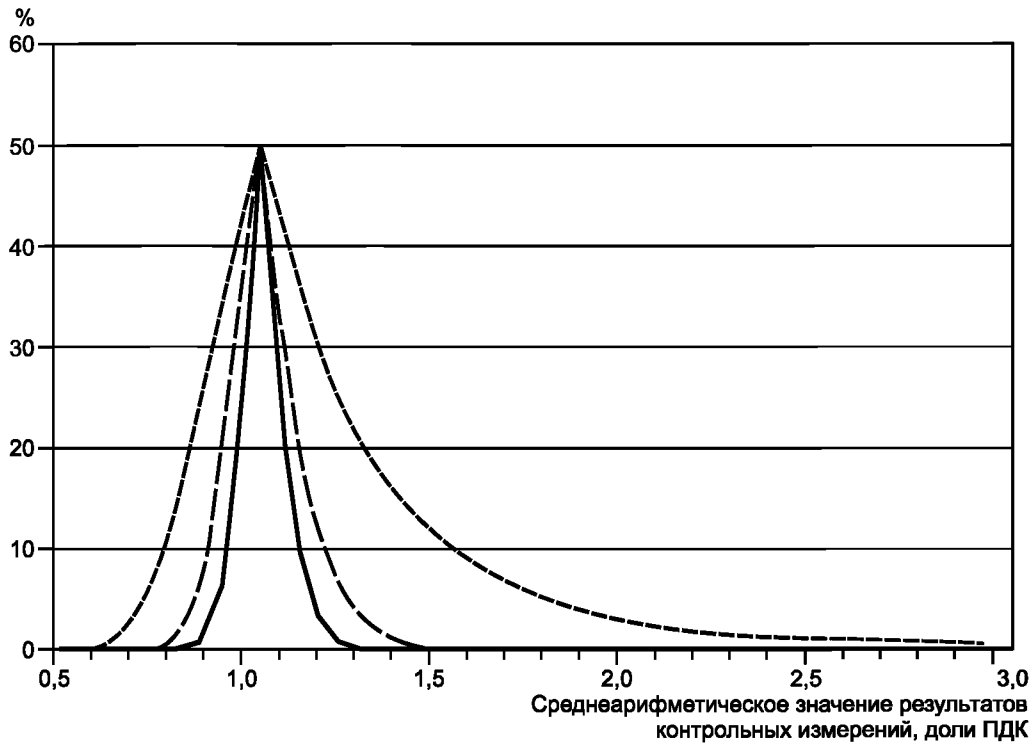
Рисунок 1 — Вероятность ложных заключений о качестве воды (ось ординат) при \delta_{изм} = 10\% . Сплошная линия соответствует \delta_{выб}/\delta_{изм} = 2 , штриховая — \delta_{выб}/\delta_{изм} = 4 , пунктирная — \delta_{выб}/\delta_{изм} = 10
