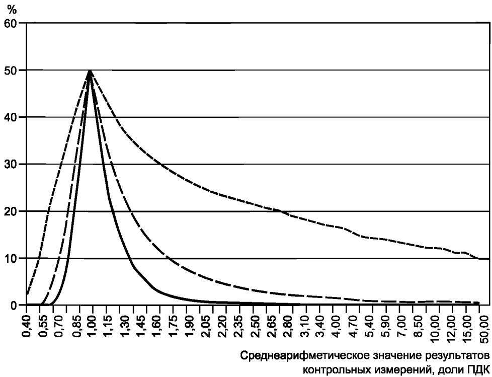
Рисунок 2 — Вероятность ложных заключений о качестве воды (ось ординат) при \delta_{изм} = 30\%
