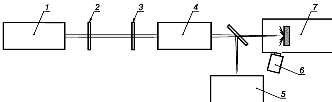
1 — лазерная система; 2 — переменный аттенюатор; 3 — фазовая пластинка; 4 — фокусирующая система; 5 — блок диагностики пучка; 6 — система онлайн-обнаружения разрушения; 7 — отсек для образцов
