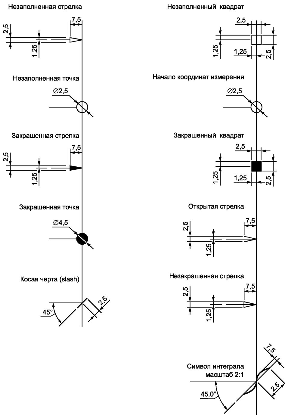
Рисунок 5 — Предопределенные изображения конца линии (размеры в миллиметрах до масштабирования)
