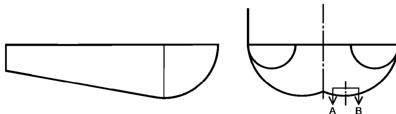
Рисунок 1 — Схема PRCLI
