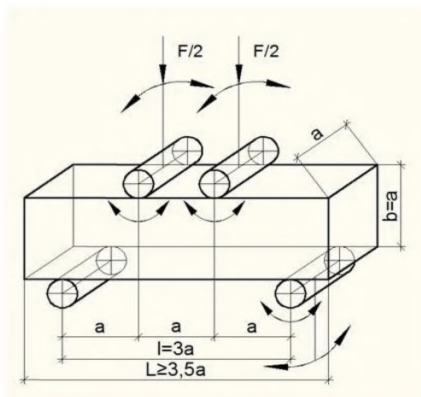
Рисунок ба – Базовая схема испытания бетона на прочность на растяжение при изгибе (цилиндрический контакт, двухточечное приложение нагрузки)
