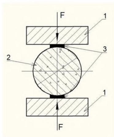
Рисунок 7 – Схема испытания кернов на растяжение при раскалывании:
