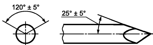
Рисунок 2 — Рекомендуемое острие скелетного штифта Стейнманна
