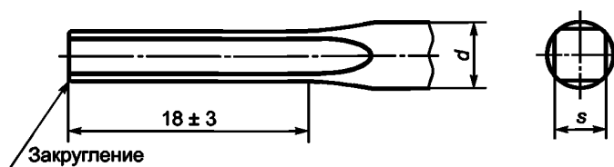
Рисунок 4 — Форма В (конец квадратного сечения)
