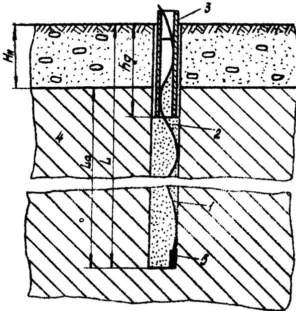
Рис.2. Скважинный глубинный заземлитель в мерзлых коренных осадочных породах:
