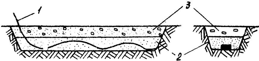
Рис.3. Траншейный заземлитель:
