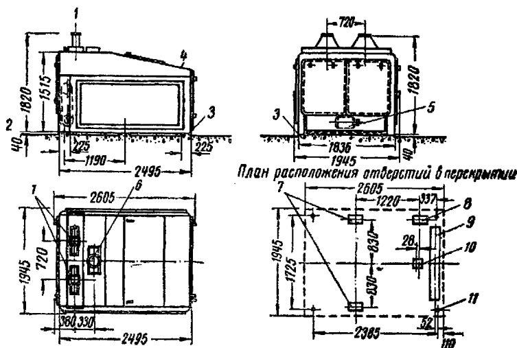
Рис. 2. Сепаратор ЗСП-10:
