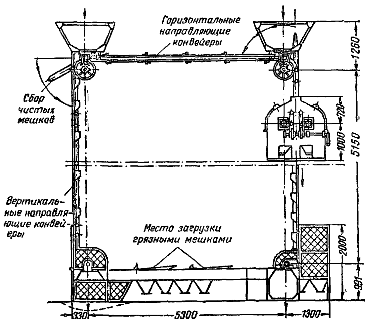
Рис. 59. Машина мешковколачивающая МВН (МТ-2)
