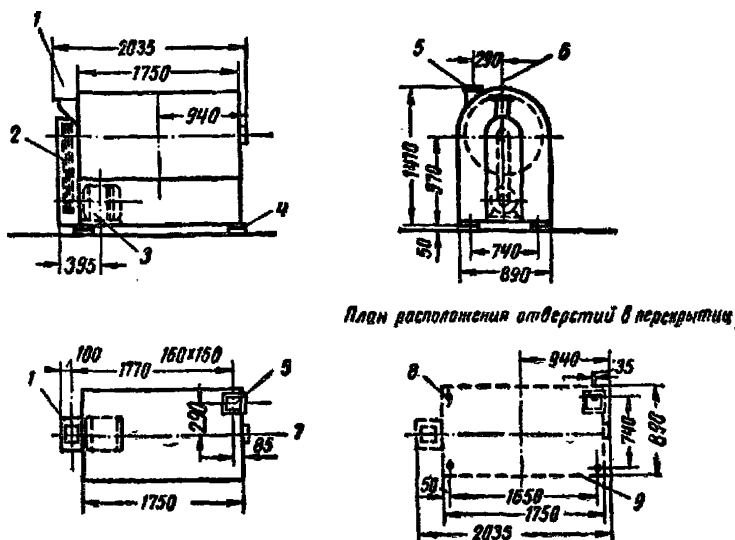
Рис. 6. Обоечная машина ЗН-10
