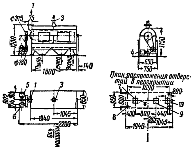
Рис. 30. Бурат цельнометаллический ЦМБ-1
