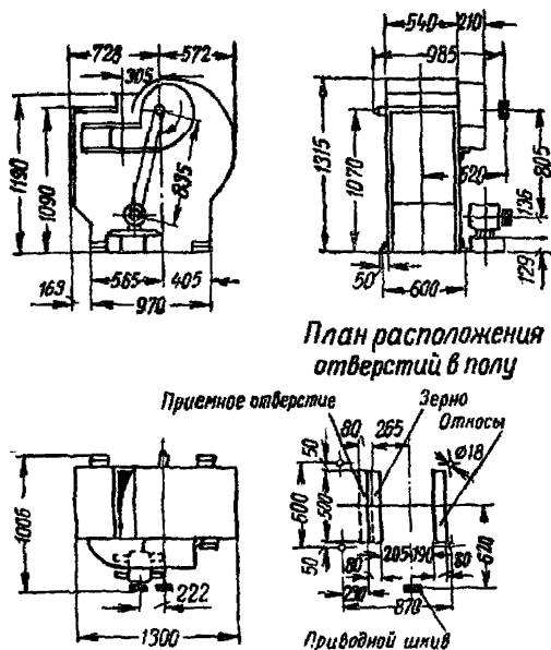
Рис. 12. Аспиратор ЗД-2,5
