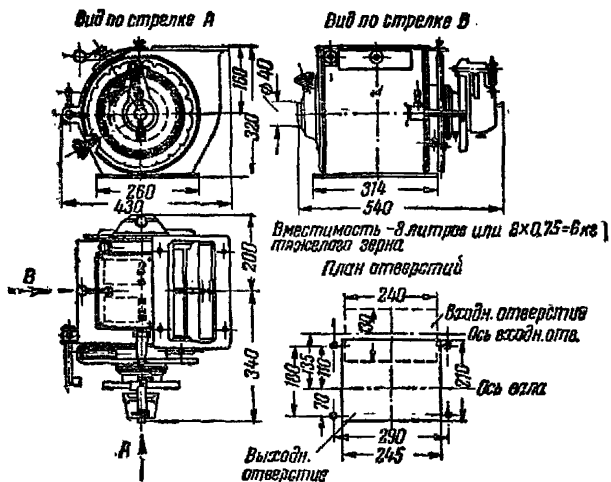
Рис. 9. Дозировщик зерновой ЗС-250 производительностью 4,5 т/ч
