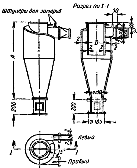
Рис. 92. Разгрузитель ЦР
