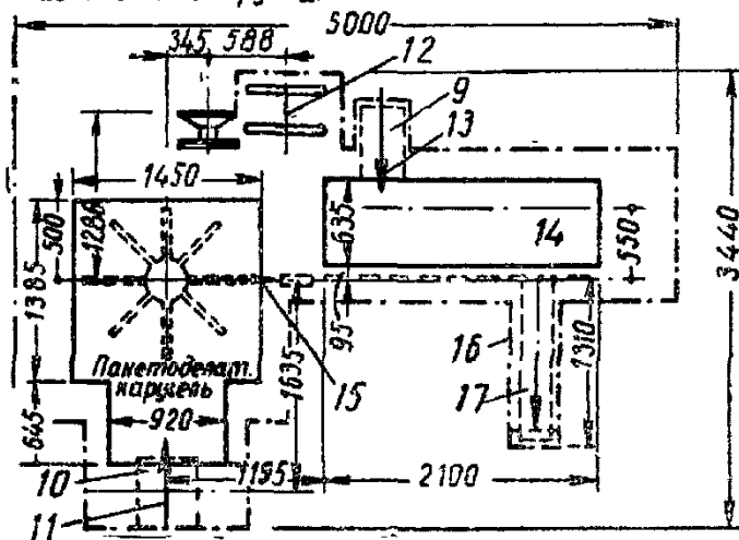
Расположение фундаментных плит в плане
