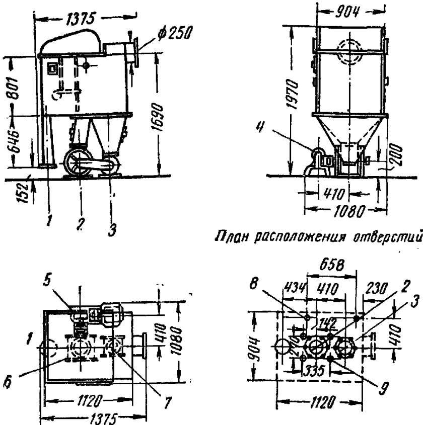
Рис. 13. Aspirатор пневматический ЗПА-10:
