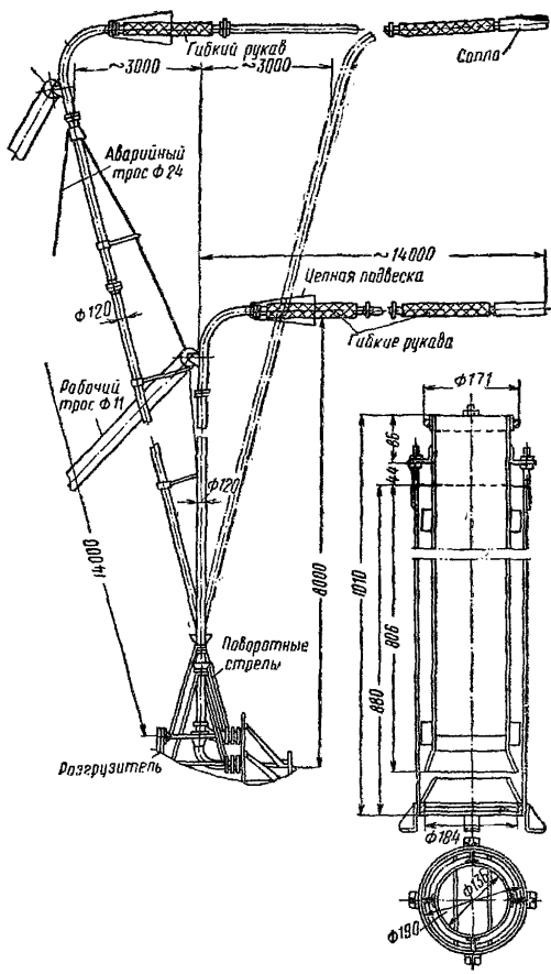
Рис. 101. Подвижной зернопровод
