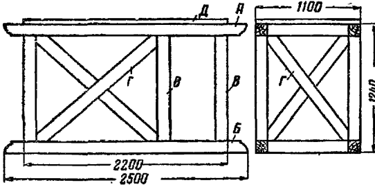
Рис. 60. Стол приемный
