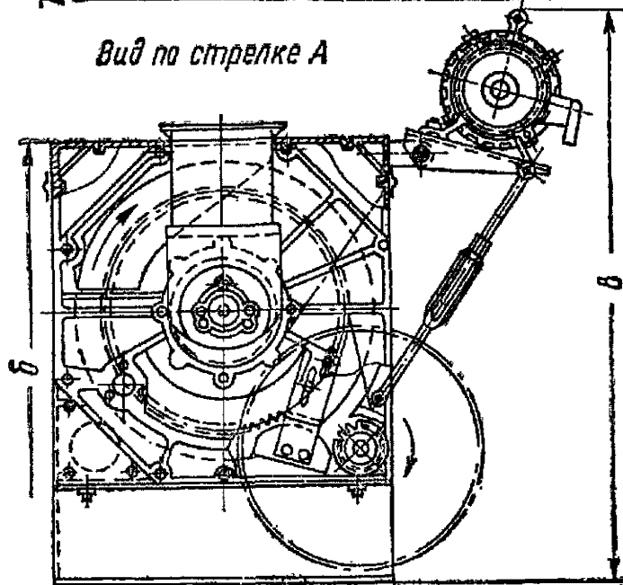
Рис. 20. Общий вид триера
