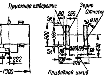
Рис. 12. Аспиратор ЗД-2,5
