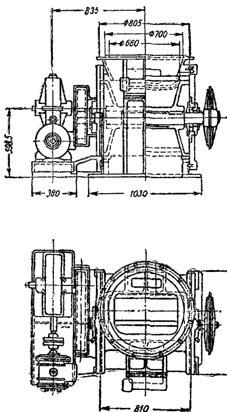
Рис. 93. Шлюзовой затвор для зерна емкостью 200 л
