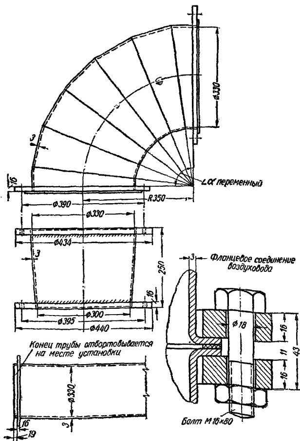
Рис. 100. Детали воздухопровода
