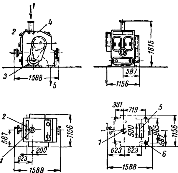
Рис. 38. Станок вальцедековый универсальный СВУ-2; 1 — прием зерна; 2 — аспирация машины; 3 — электродвигатель 10 квт; 4 — питательный валик; 5 — выход продукта; 6 — четыре отверстия \varnothing 30 мм
