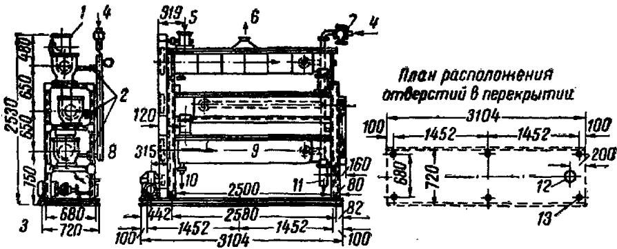
Рис. 48. Сушилка паровая
