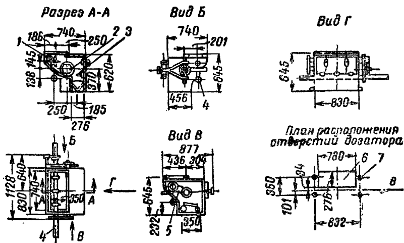
Рис 45. Дозатор ДП-1:
