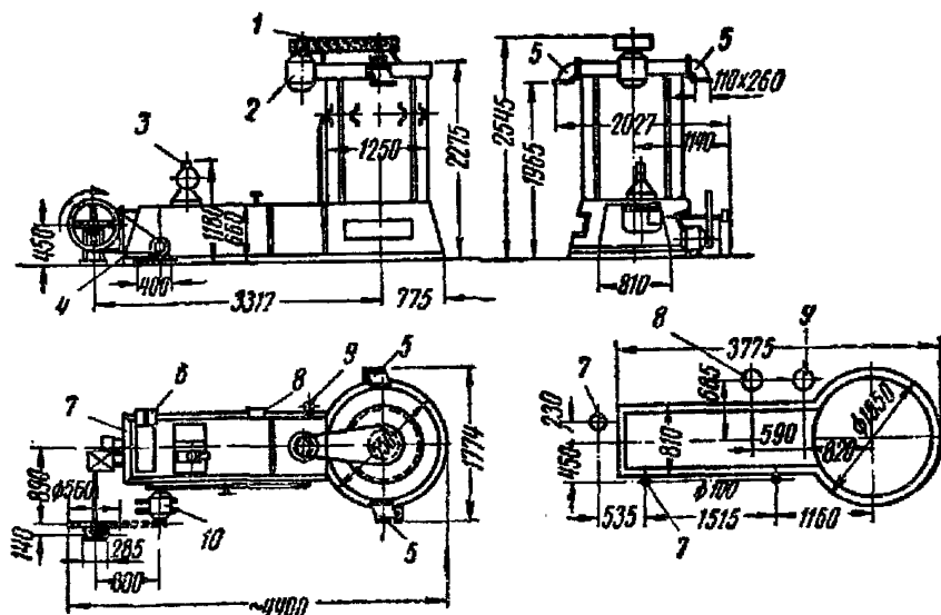
Рис. 8. Машина моечная комбинированная ЗКМ-60:
