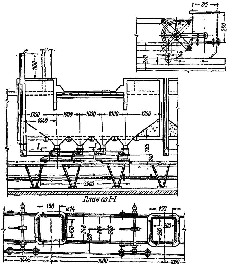
Рис. 76. Подамбарные задвижки автотранспортного приема
