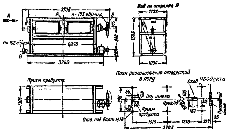
Рис. 29. Бурат центробежный ЗЦ-1Б
