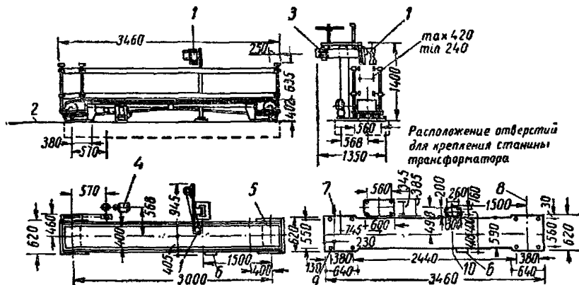
Рис. 58. Мешкозашивочная машина ЗЗЕМ
