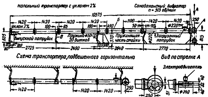
Рис. 68. Вибрационный транспортер
