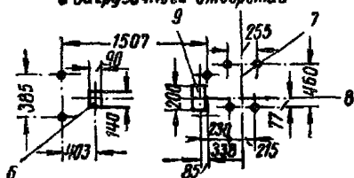
Расположение фундаментных болтов выходного и загрузочного отверстий
