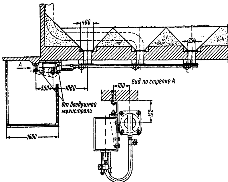
Рис. 83. Надвесовая задвижка с пневмоэлектроприводом на 9 отверстий (разрез)
