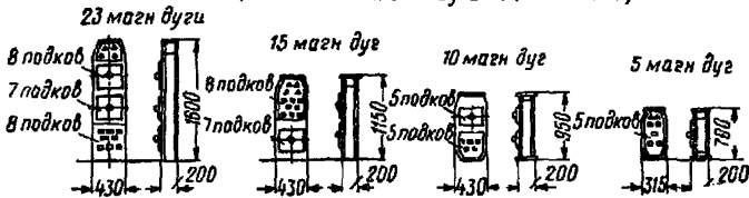
Ящики с магнитными дугами (подковами)
