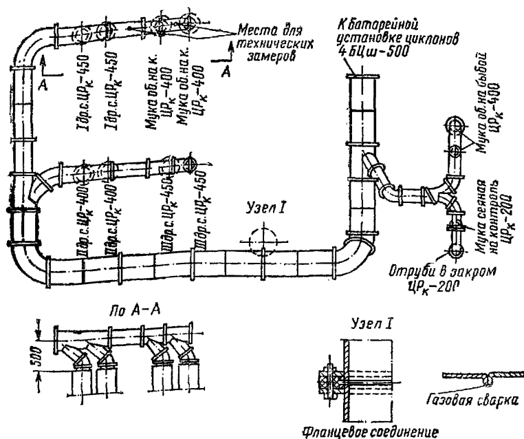
Рис. 97. Коллектор размольного отделения
