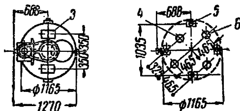
Рис. 33. Вертикальная щеточная машина
