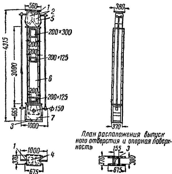
Рис. 39. Колонка охладительная
