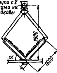
Установка магнитных сборок для муки с 2 ящиками на 15 подков
