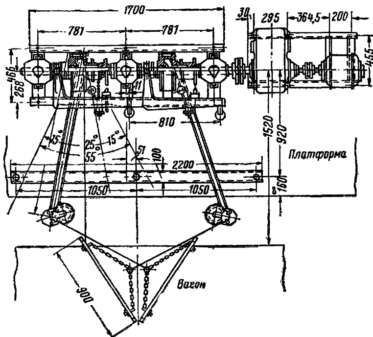
Рис. 78. Сдвоенная механическая лопата ТМЛ-2
