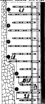
Положение забоя после снятия стругом полосы 1,0 м и при посадке
