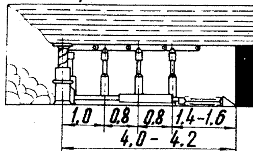
Разрез по III-III
