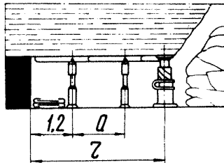
Разрез I-I
