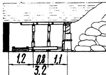
Разрез по III-III
